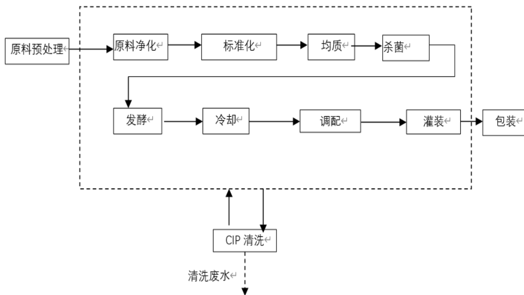
图2 发酵乳饮料生产工艺流程图
