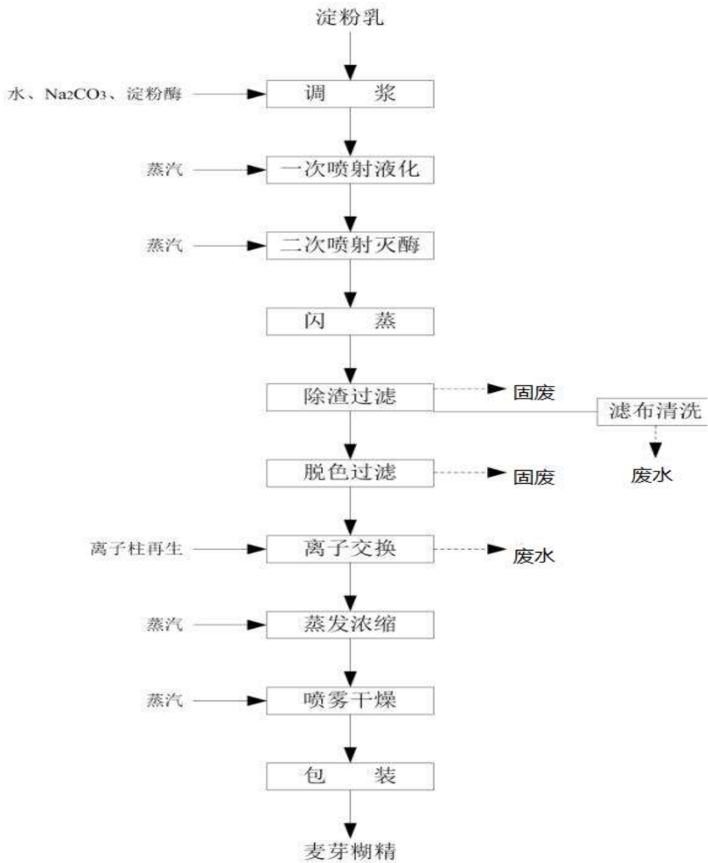
麦芽糊精生产工艺及排污节点图
