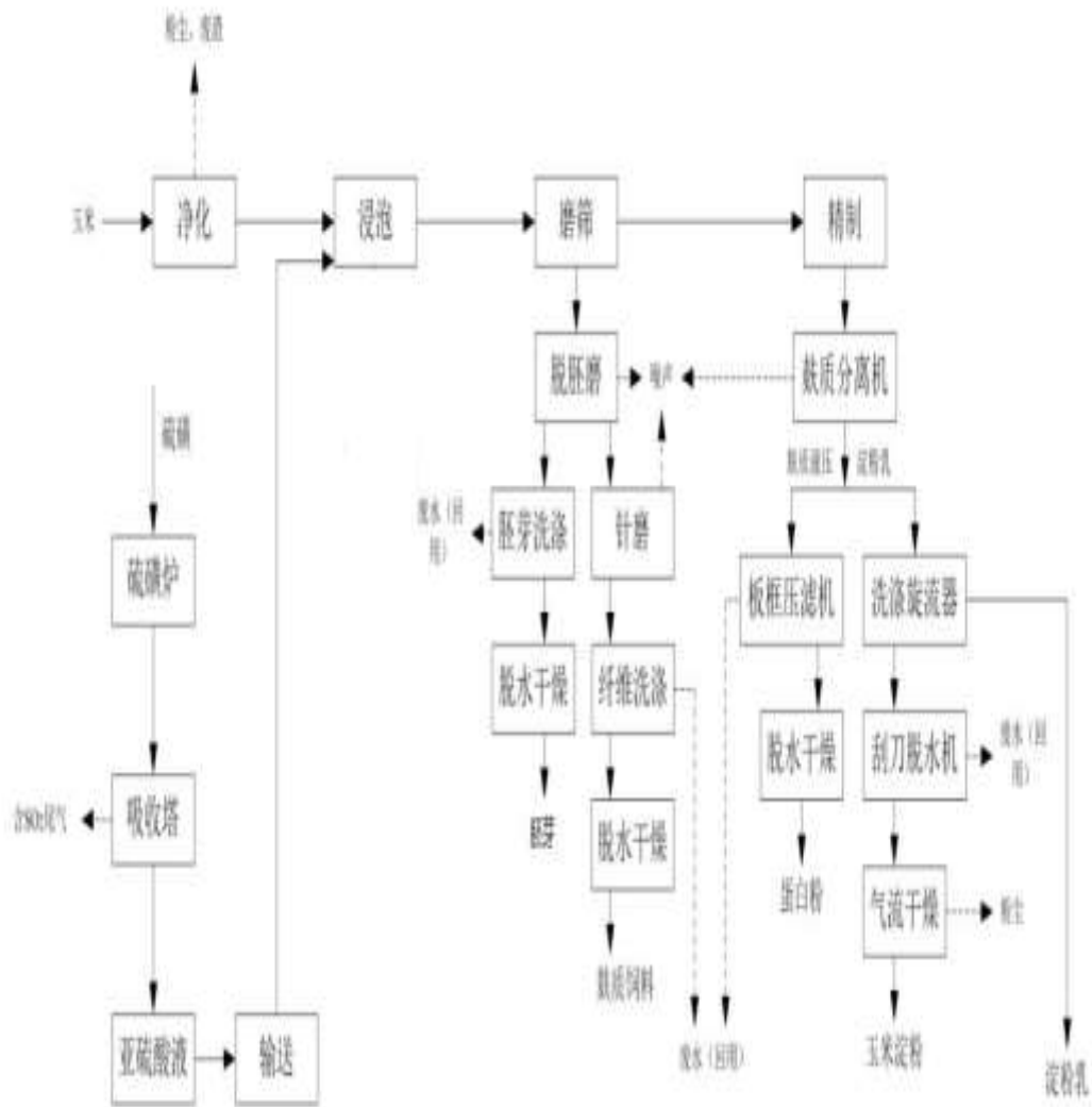
淀粉生产工艺流程及排污节点图
