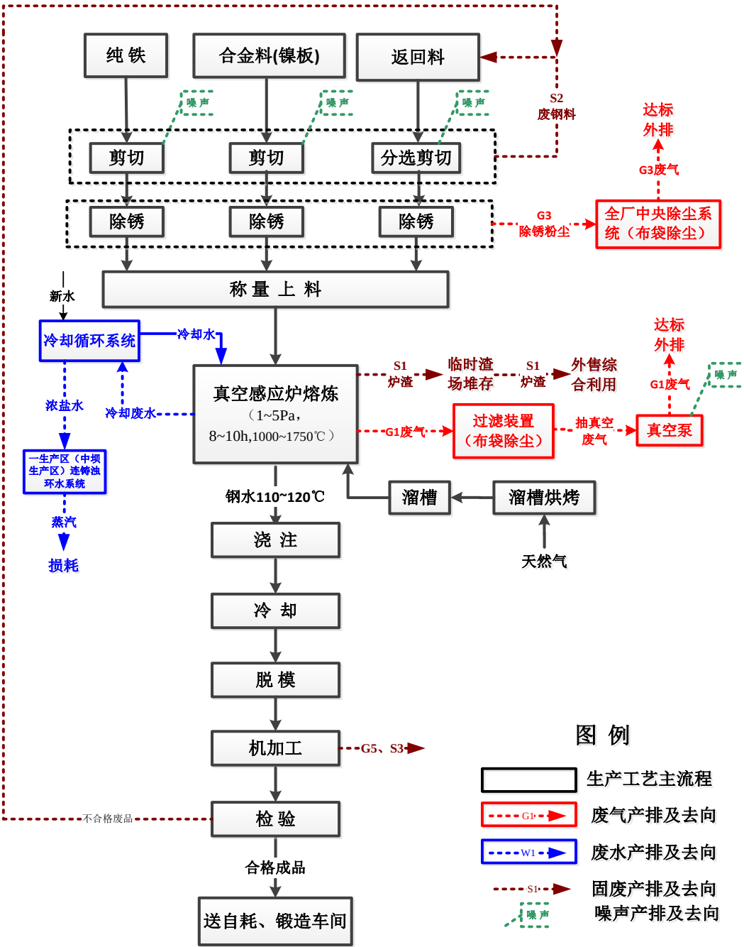
图 3.5-6 真空感应炉冶炼工艺流程及产污位置图
