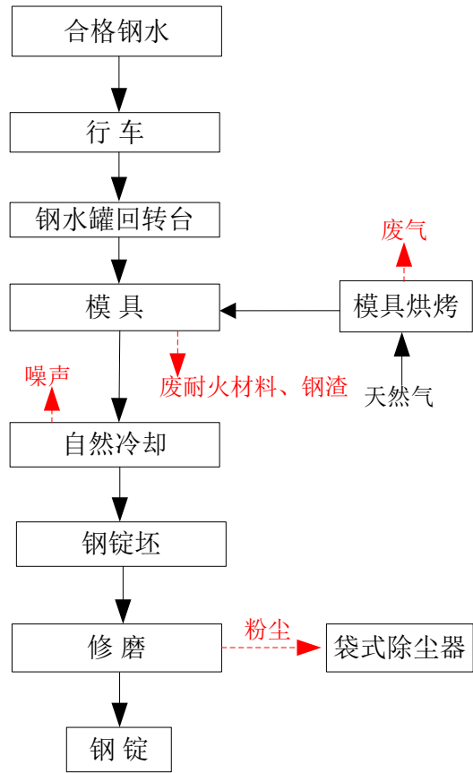
图 3.5-5 模铸生产工艺流程及产污位置图
