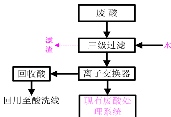
图 3.5-14 废酸再生工艺流程及产污位置图
