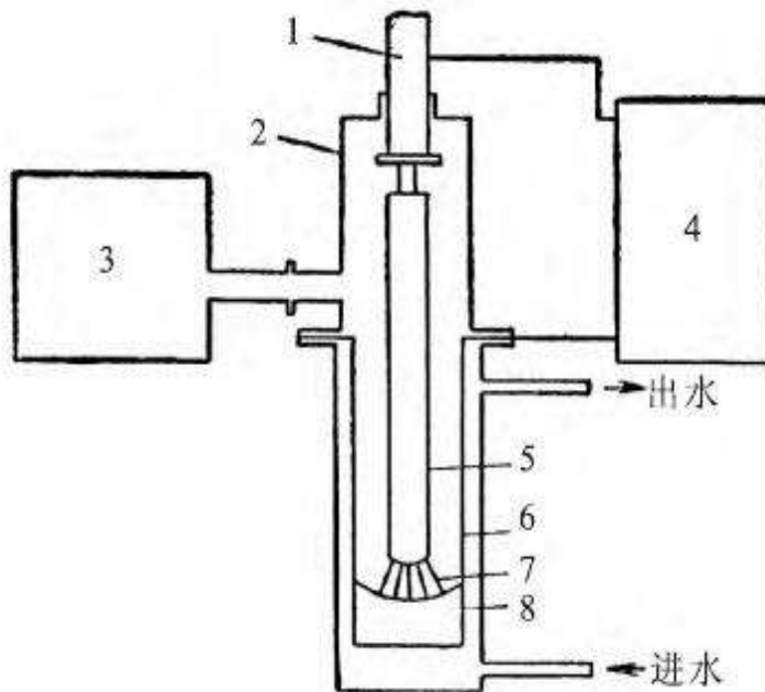
1.电极夹持器 2.炉室 3.真空泵 4.供电电源和控制柜 5.自耗电极； 6.水冷结晶器 7.电弧 8.熔炼好的钢锭
