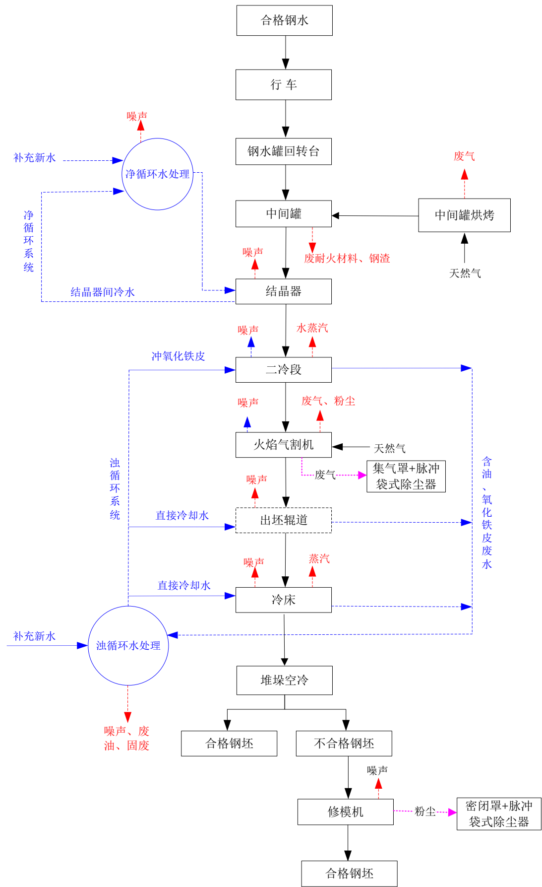
图 3.5-4 连铸生产工艺流程及产污位置图
