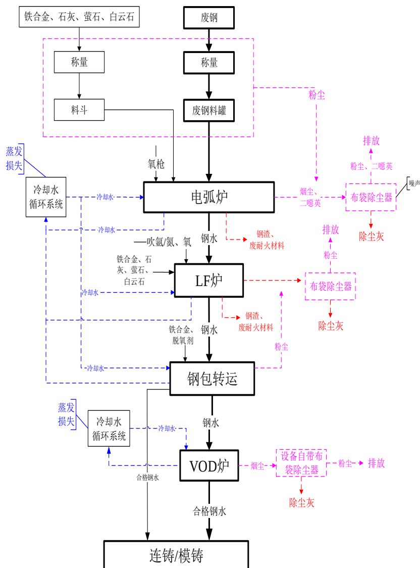
图 3.5-2 特种不锈钢冶炼工艺流程及产污位置图
