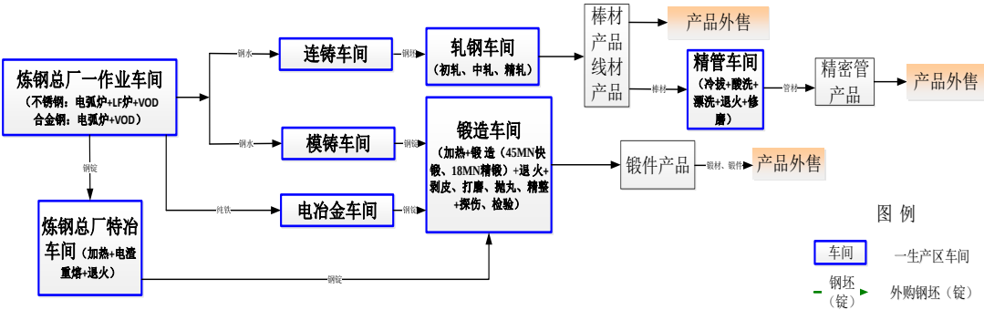
图 3.5-1 一生产区生产区（中坝生产区）各自车间相互关联图
