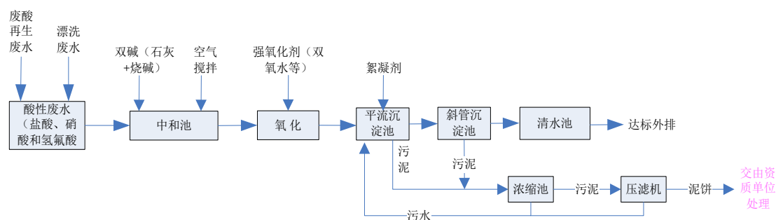
图 3.5-15 酸性废水处理系统工艺流程
