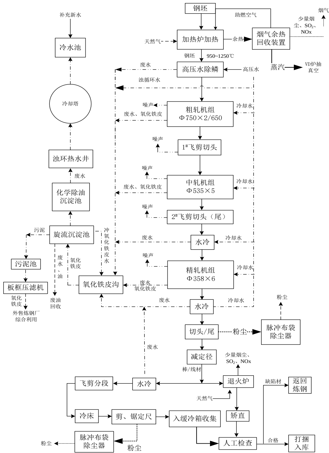
图 3.5-11 连轧生产工艺流程及污染位置图
