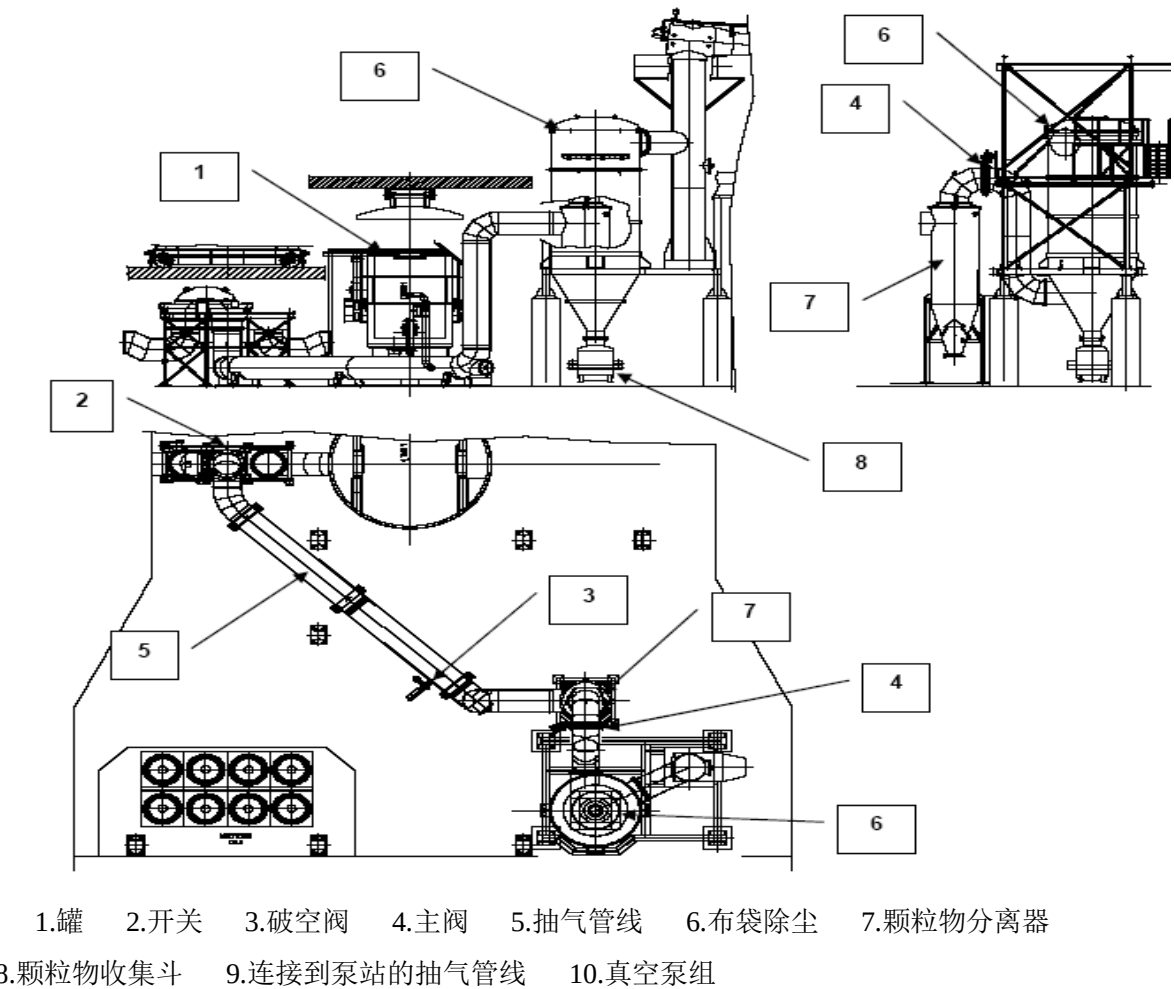
图 4.2-6 除尘系统示意图
