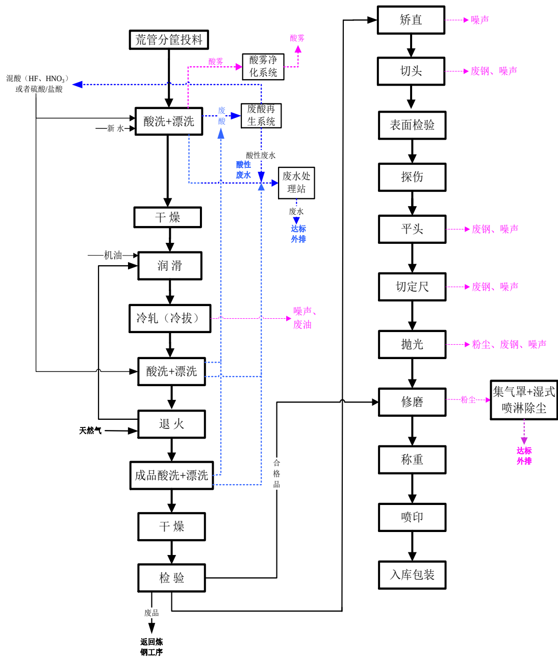
图 3.5-13 精密管生产工艺流程及产污位置图
