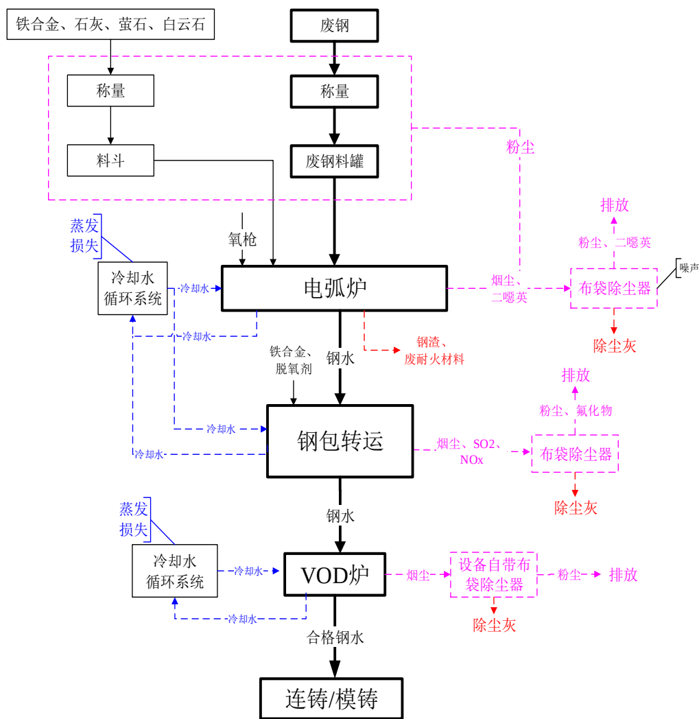
图 3.5-3 合金钢（碳钢）冶炼工艺流程及产污位置图
