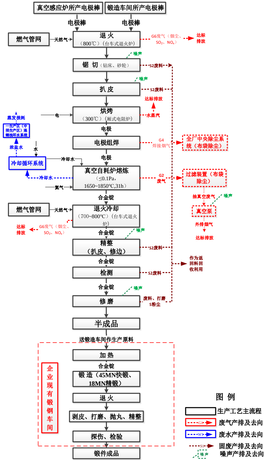
图 3.5-8 真空自耗炉冶炼工艺流程及产污位置图
