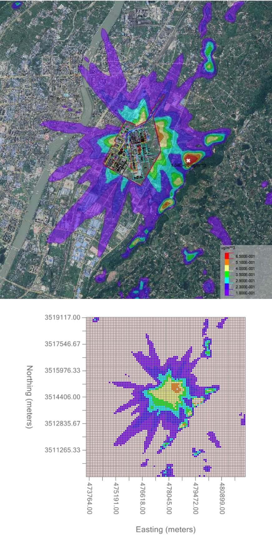
图 8.1-3 \text{NO}_x 区域最大日平均浓度贡献浓度图 单位: \mu\text{g}/\text{m}^3
