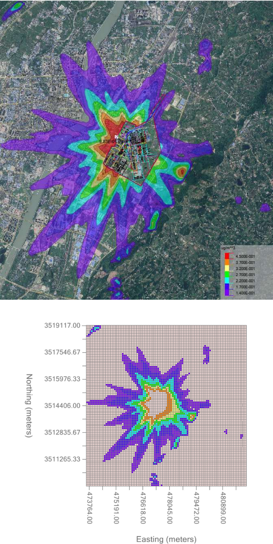
图 8.1-11 氟化物区域最大日平均浓度贡献浓度图 单位： \mu\text{g}/\text{m}^3
