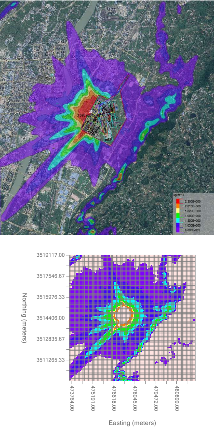
图 8.1-10 氟化物区域最大小时平均浓度贡献浓度图 单位: \mu\text{g}/\text{m}^3
