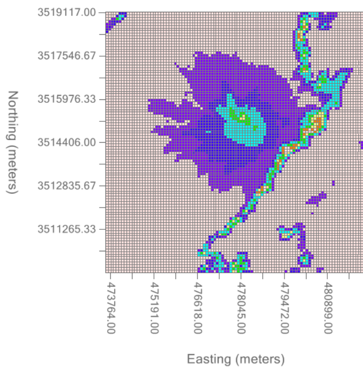
图 8.1-2 NO x 区域最大小时平均浓度贡献浓度图 单位: \mu\text{g}/\text{m}^3
