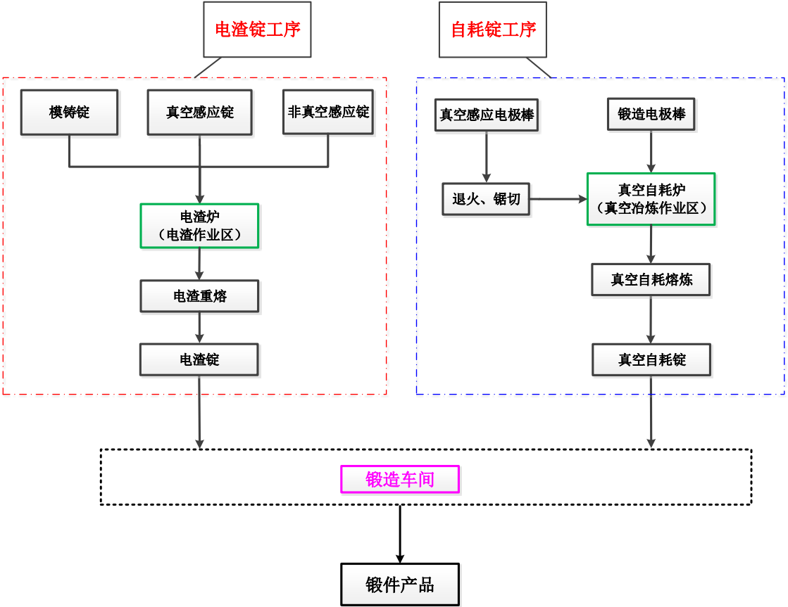
图 4.2-1 本项目电渣炉生产工序与真空自耗炉工序生产工序相互关联图
