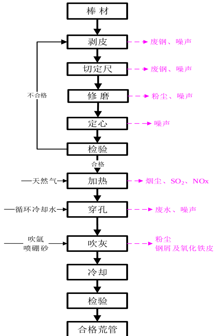
图 3.5-12 热穿孔生产工艺流程及产污位置图
