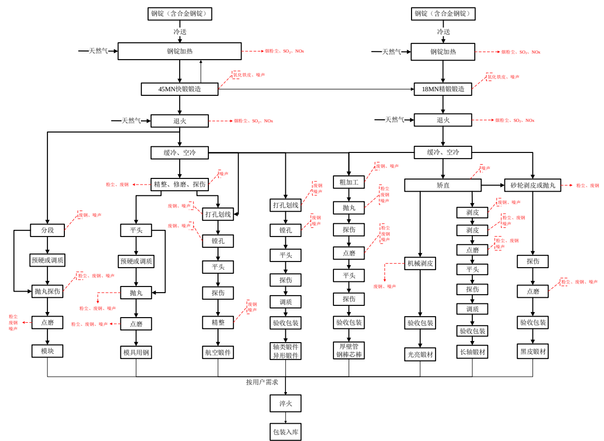
图 3.5-10 锻钢生产工艺流程及产污位置图
