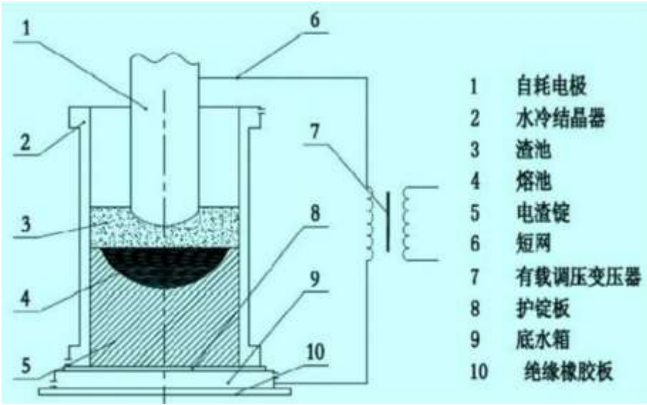
图 4.2-2 电渣重熔原理示意图
