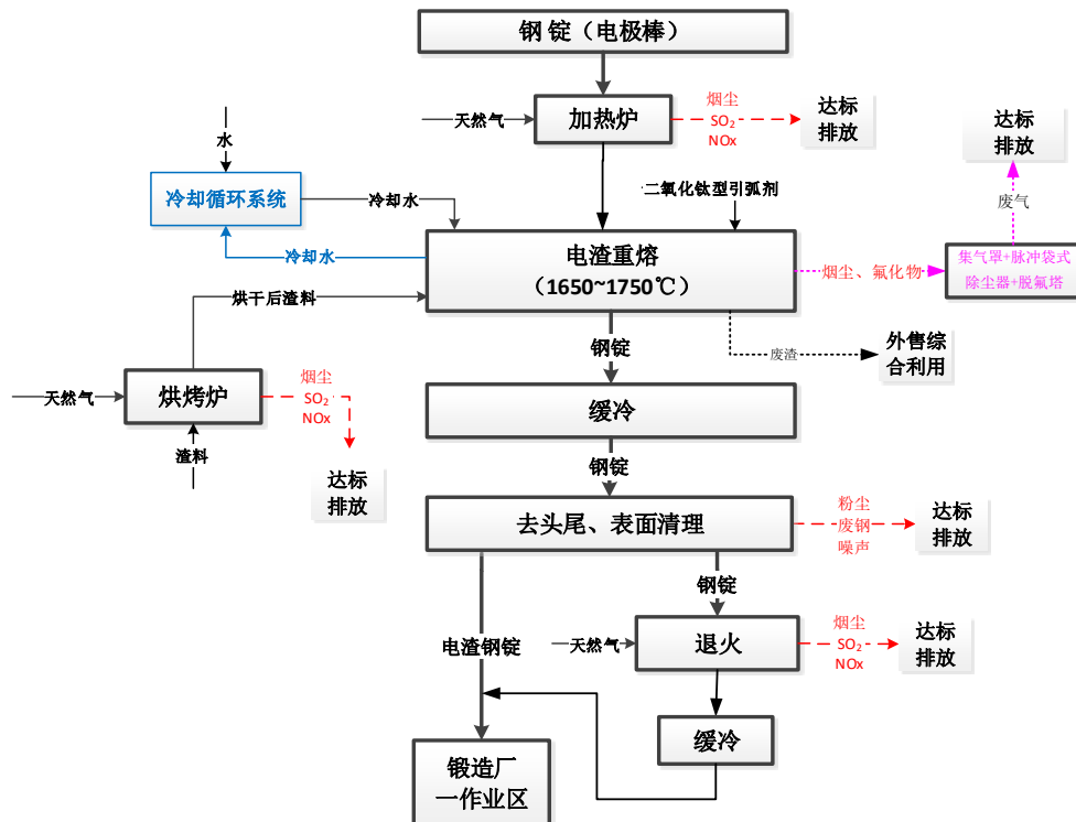
图 3.5-9 高端模具钢锻件生产工艺流程及产污示意图
