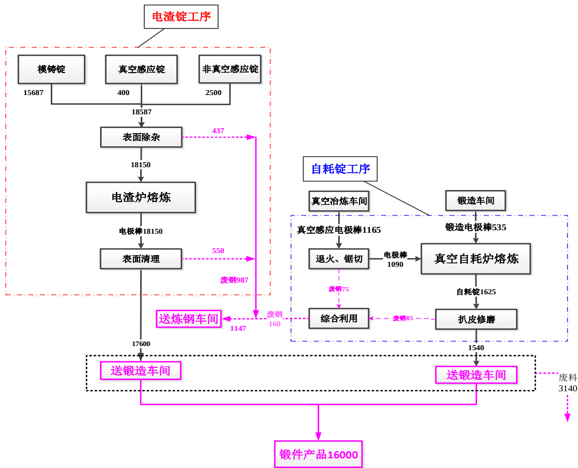
图 4.1-1 项目生产工序与企业现有生产系统相互关联图
