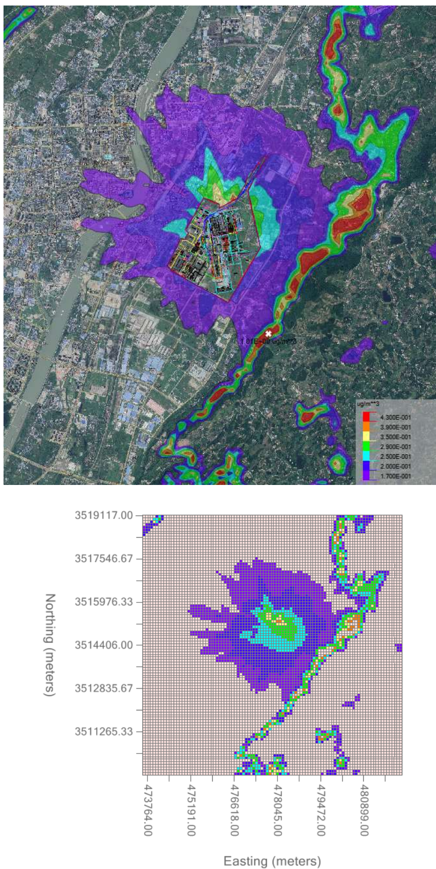
图 8.1-5 SO 2 区域最大小时平均浓度贡献浓度图 单位: \mu\text{g}/\text{m}^3
