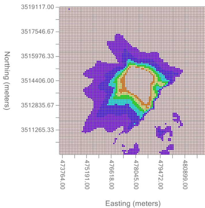
图 8.1-4 \text{NO}_x 区域最大年平均浓度贡献浓度图 单位: \mu\text{g}/\text{m}^3
