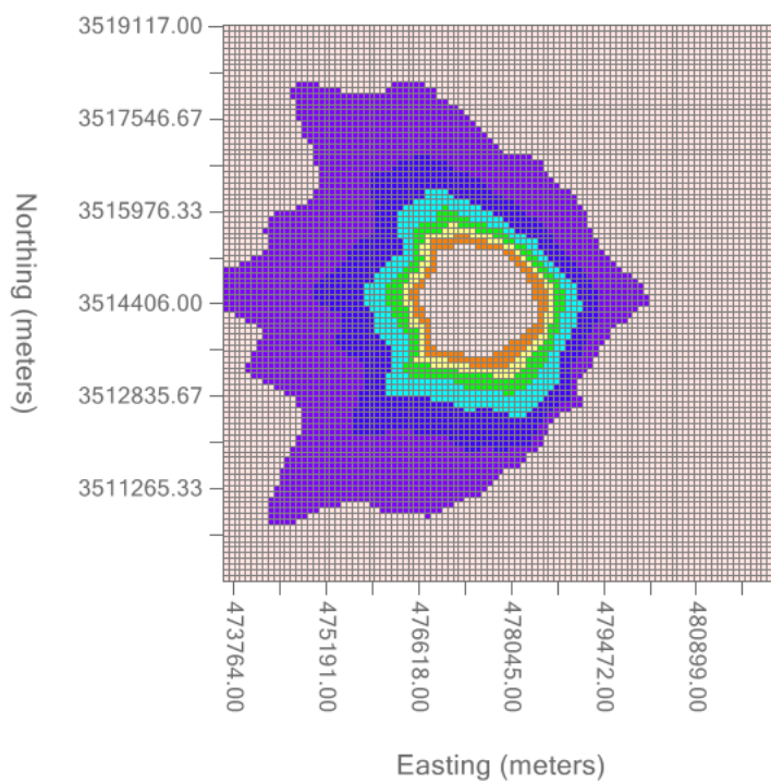
图 8.1-9 PM 10 区域最大年平均浓度贡献浓度图 单位: \mu\text{g}/\text{m}^3
