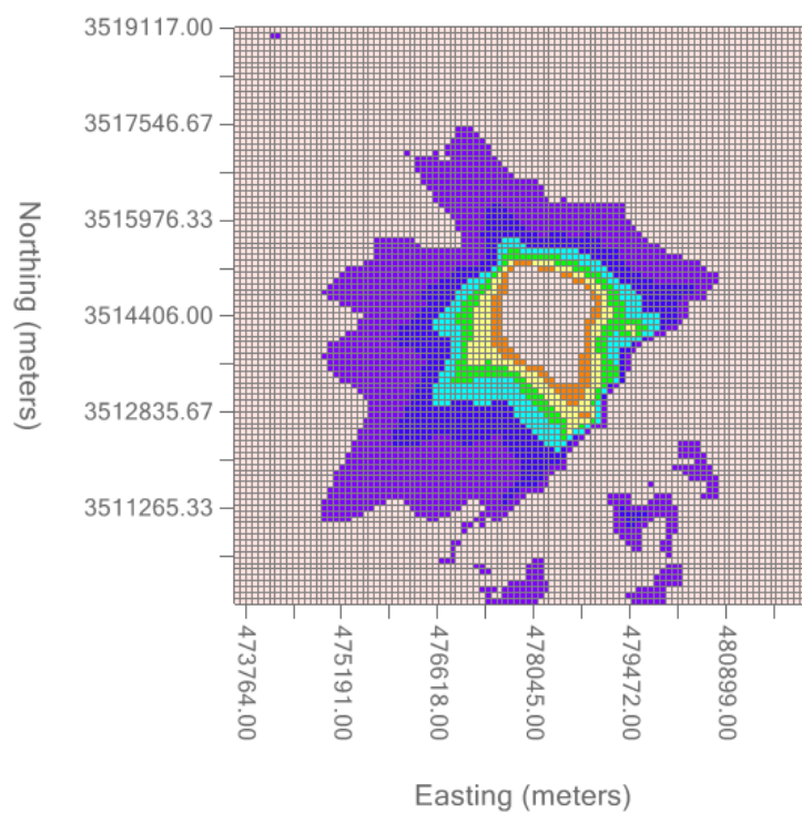
图 8.1-7 SO 2 区域最大年平均浓度贡献浓度图 单位: \mu\text{g}/\text{m}^3
