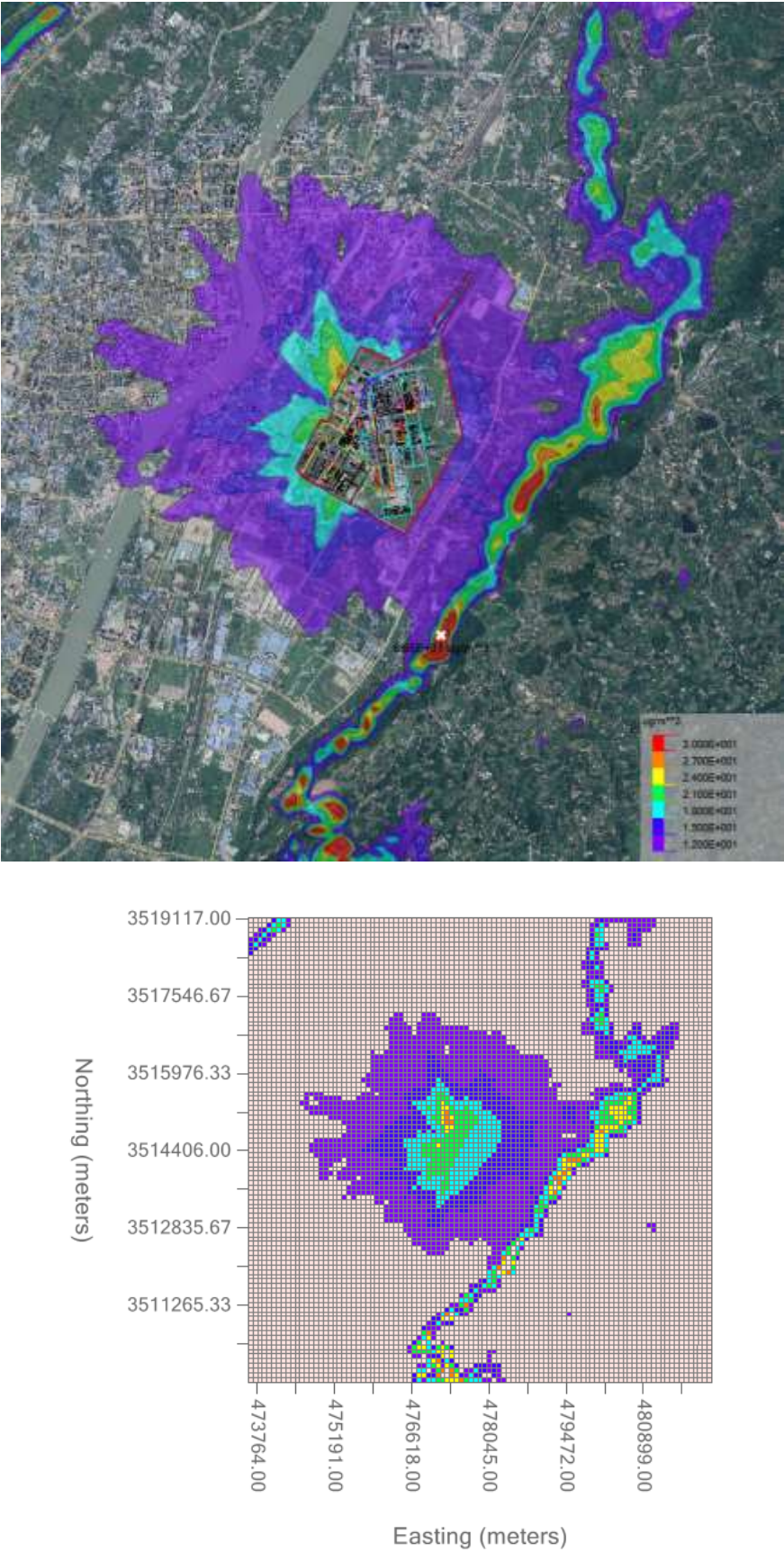
图 8.1-12 非正常排放下 PM_{10} 小时最大浓度等值线图 (2018 年 1 月 17 日 18 时)
