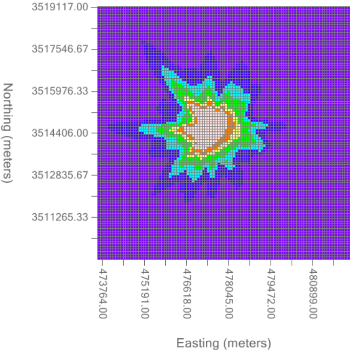
图 8.1-8 PM 10 区域最大日平均浓度贡献浓度图 单位: \mu\text{g}/\text{m}^3
