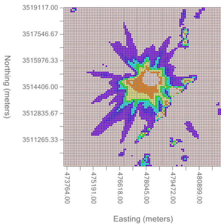
图 8.1-6 SO 2 区域最大日平均浓度贡献浓度图 单位: \mu\text{g}/\text{m}^3
