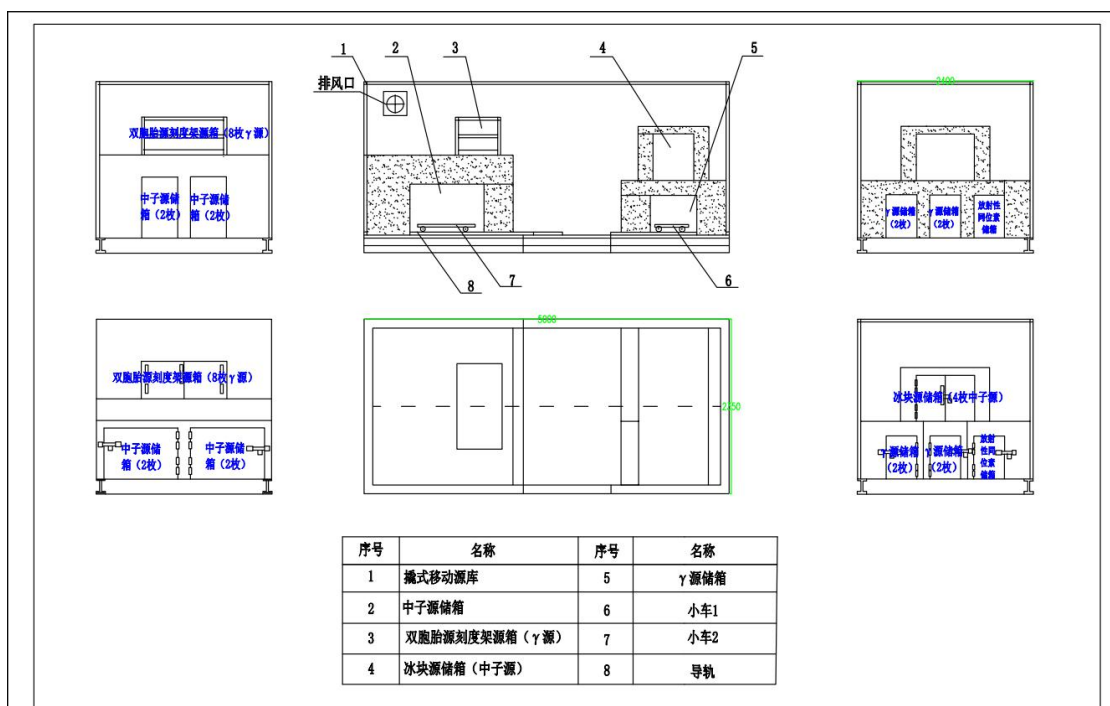
图 10-2 源库结构示意图
