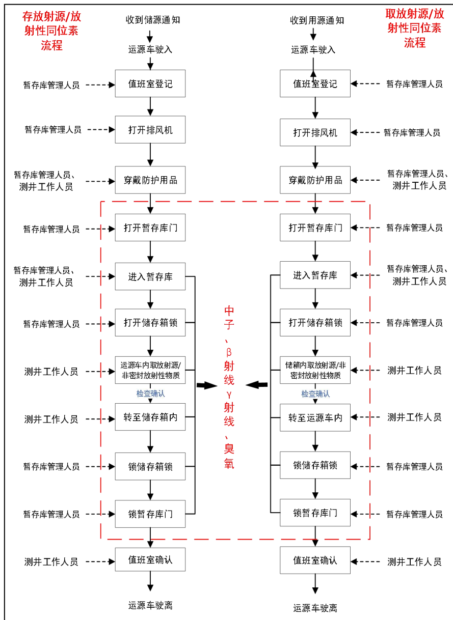
图 9-1 放射源/非密封放射性物质贮存管理流程及产污环节图
