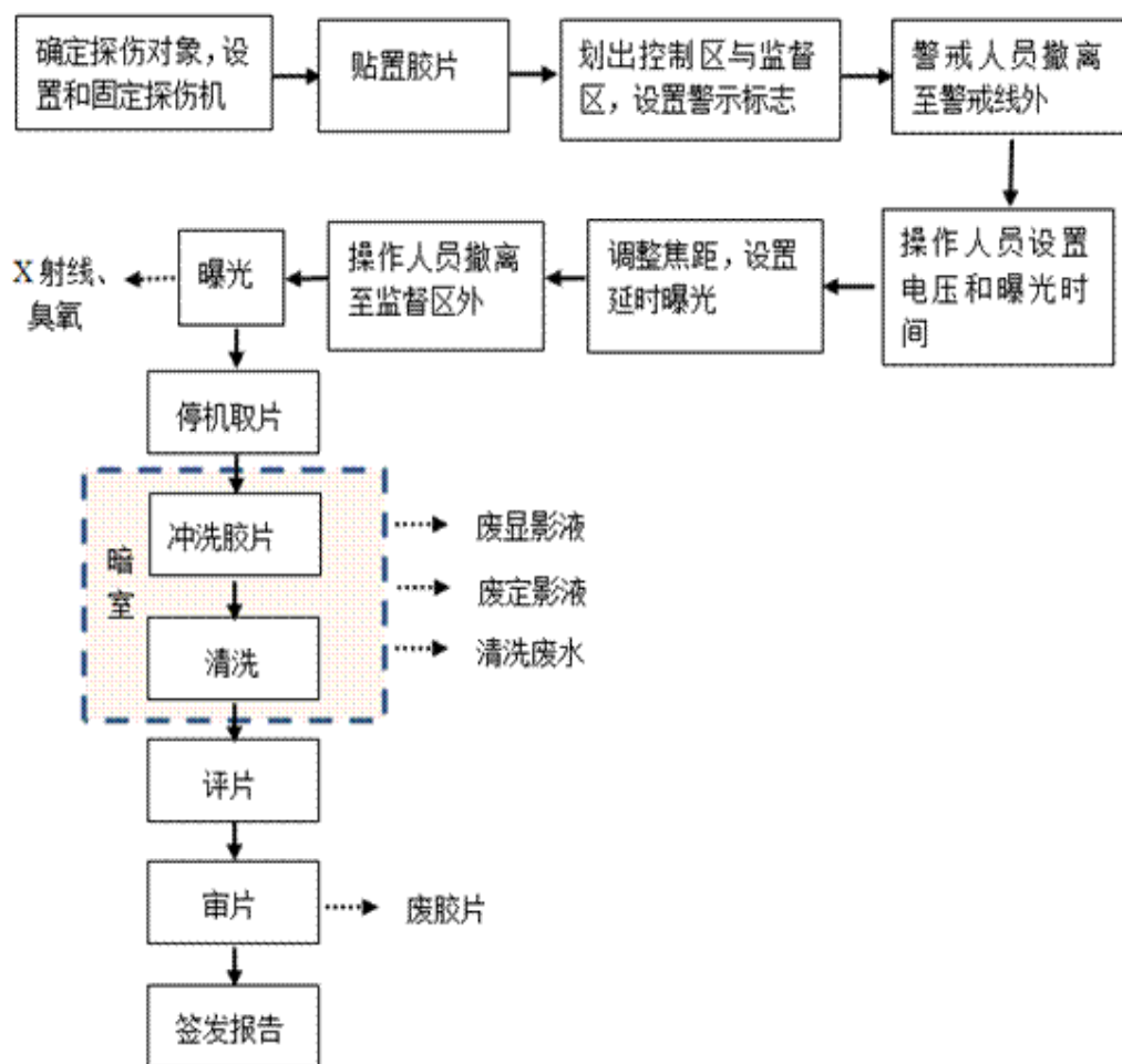
图 9-2 探伤机操作流程及产污环节示意图
