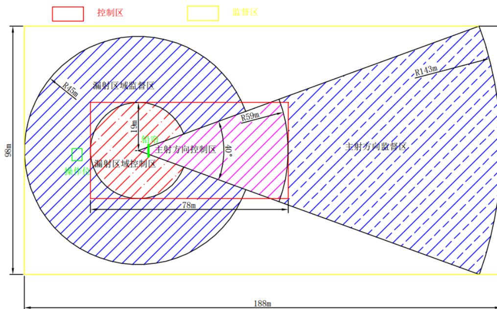
10-1 本项目 XXG-3005 型探伤机正常工作时监督区和控制区划分示意图 (主射方向 2.5mm 铅当量铅屏风屏蔽状态下)
