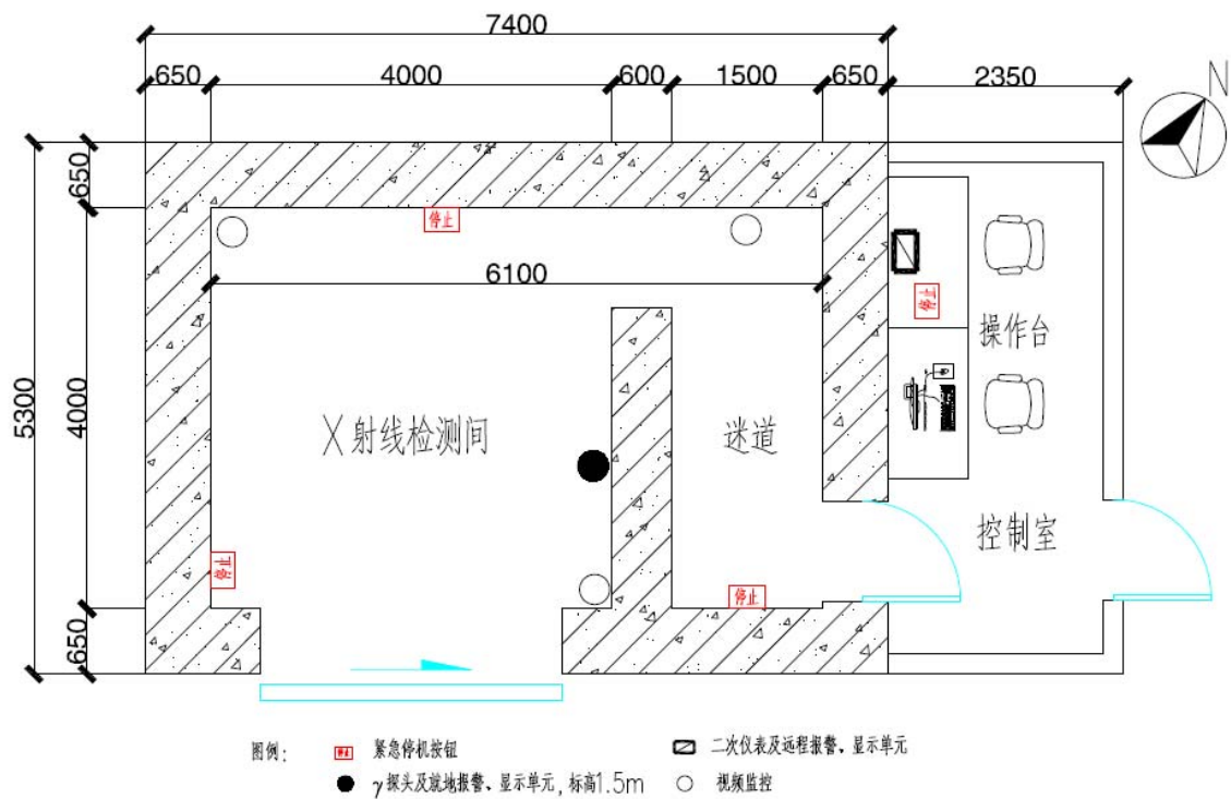
图 10-4 探伤室安全设施布置示意图
