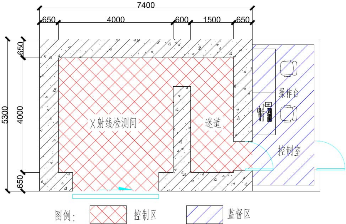
图10-1 本项目“两区”分布图
