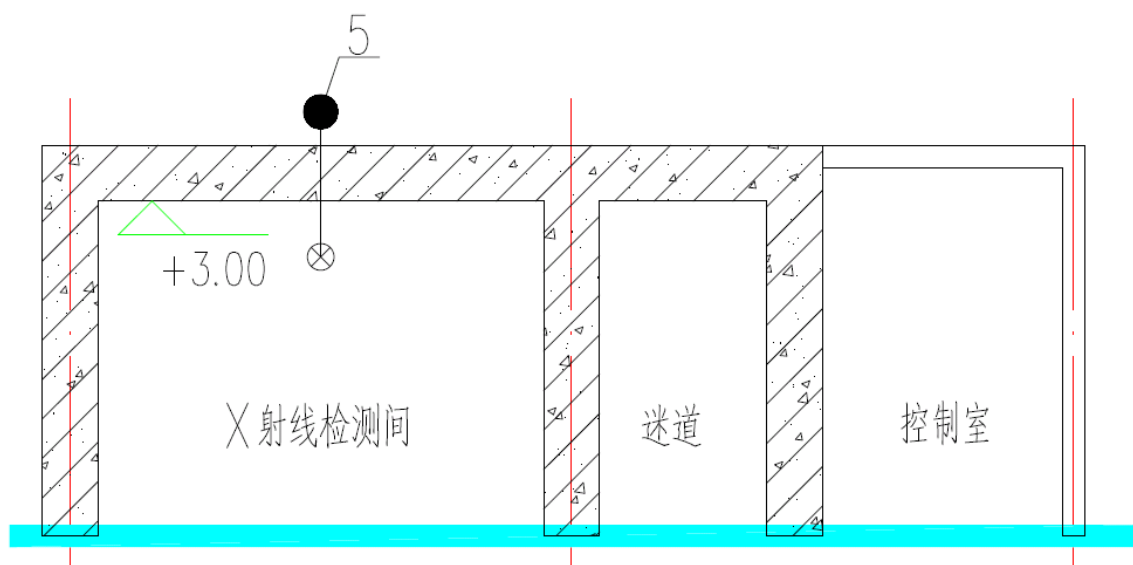
图11-2 探伤室关注点位图（剖面）
