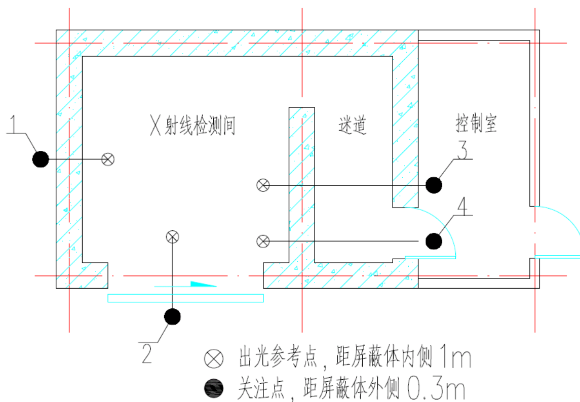
图11-1 探伤室关注点位图（平面）
