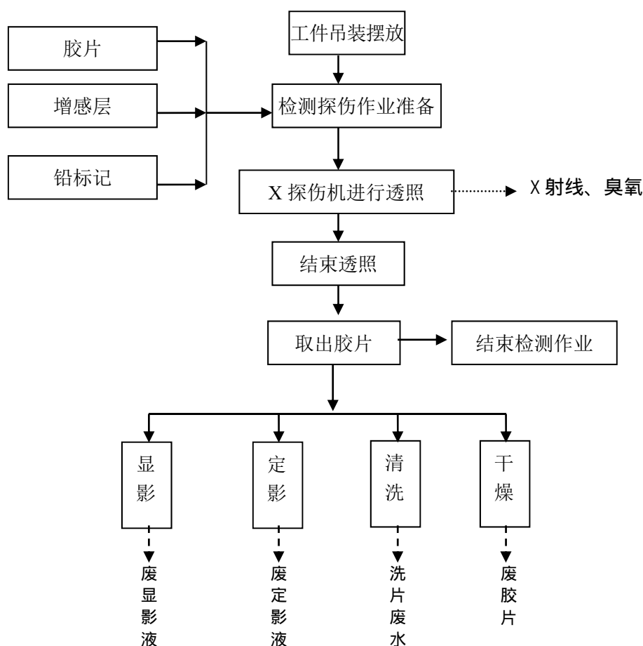
图 9-3 X 射线探伤机工艺流程及产污图
