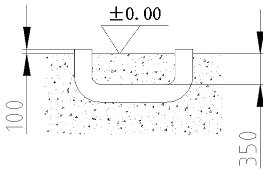
图 10-3 通排风管道及电缆进出口管道结构图
