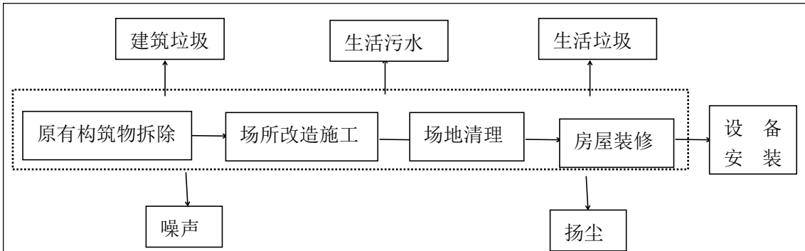
图 9-1 施工期施工流程图
