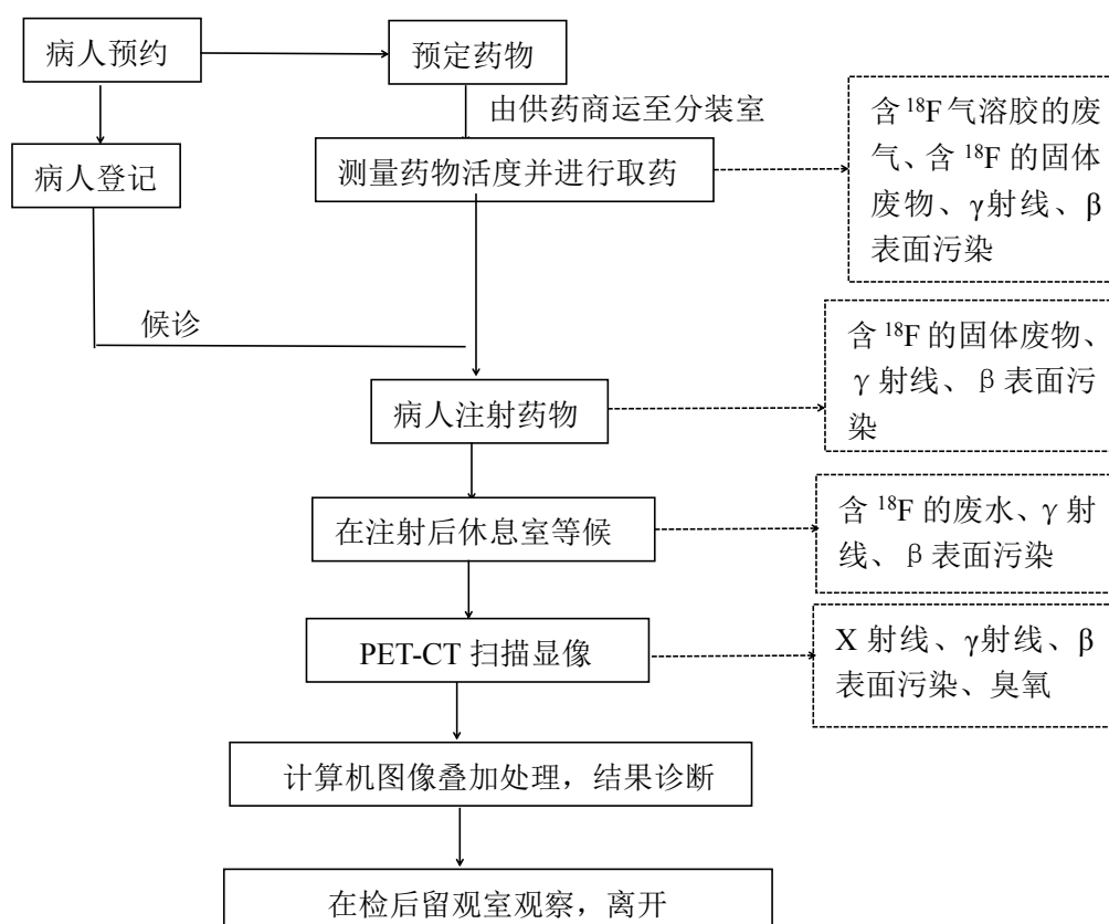
图 9-2 PET-CT 显像诊断及产污流程图
