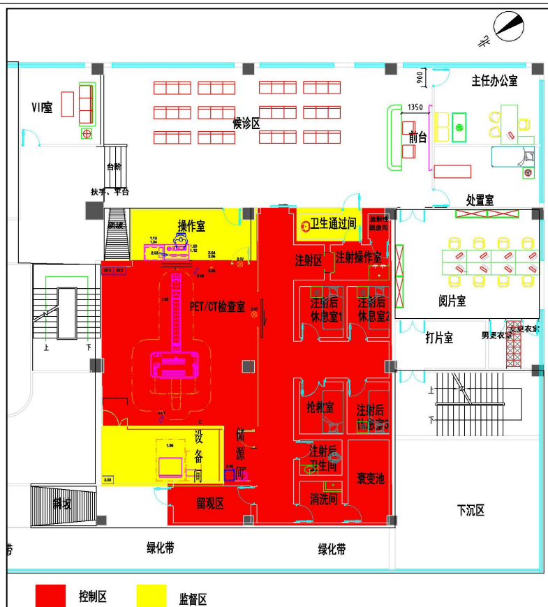
图 10-2 PET/CT 检查区域两区划分图
