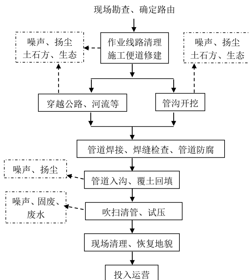
图 4.1-8 集输管线主要施工工序及产污环节示意图
