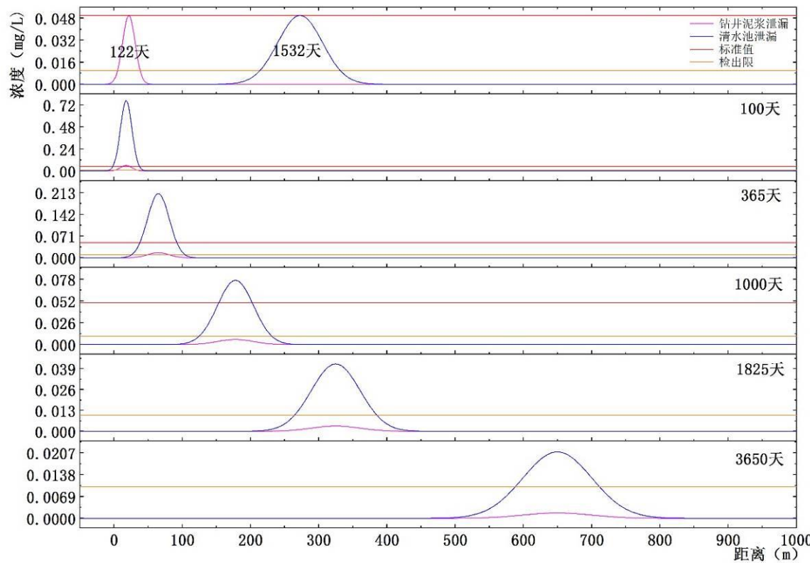
图 6.4-5 污染物石油类距离与浓度关系曲线示意图
