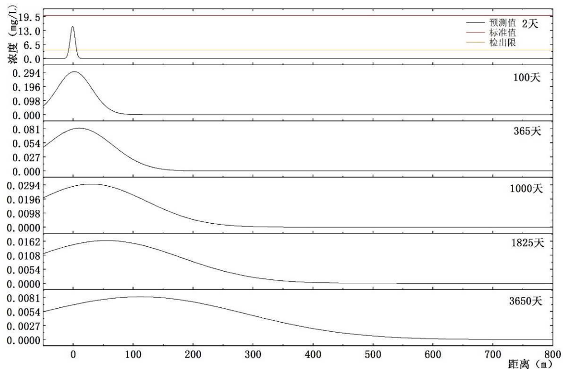
图 7.3-1 污染物 COD 距离与浓度关系曲线示意图
