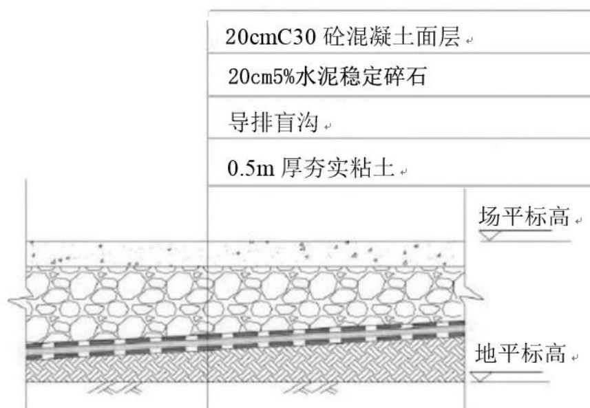
图9.5-3 重点防渗区地坪防渗结构剖面示意图
