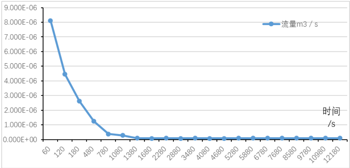
T1 渗水试验 Q—t 曲线图
