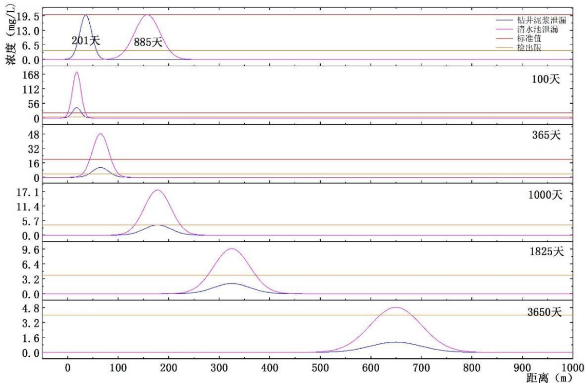
图 6.4-4 污染物 COD 距离与浓度关系曲线示意图
