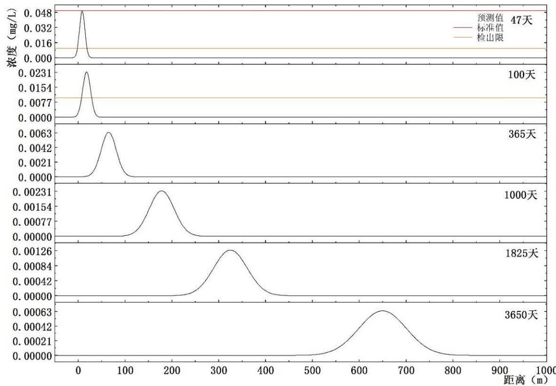
图 7.3-5 污染物石油类距离与浓度关系曲线示意图
