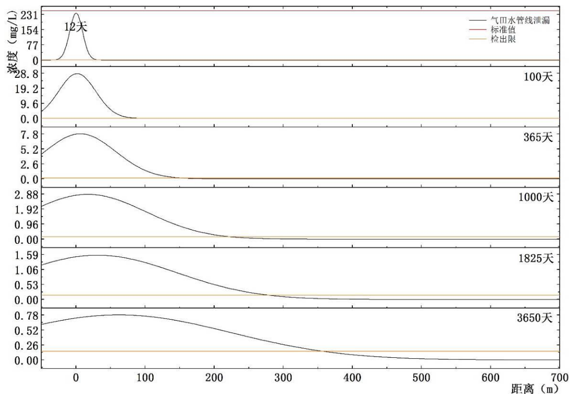
图 6.4-9 污染物氯化物距离与浓度关系曲线示意图
