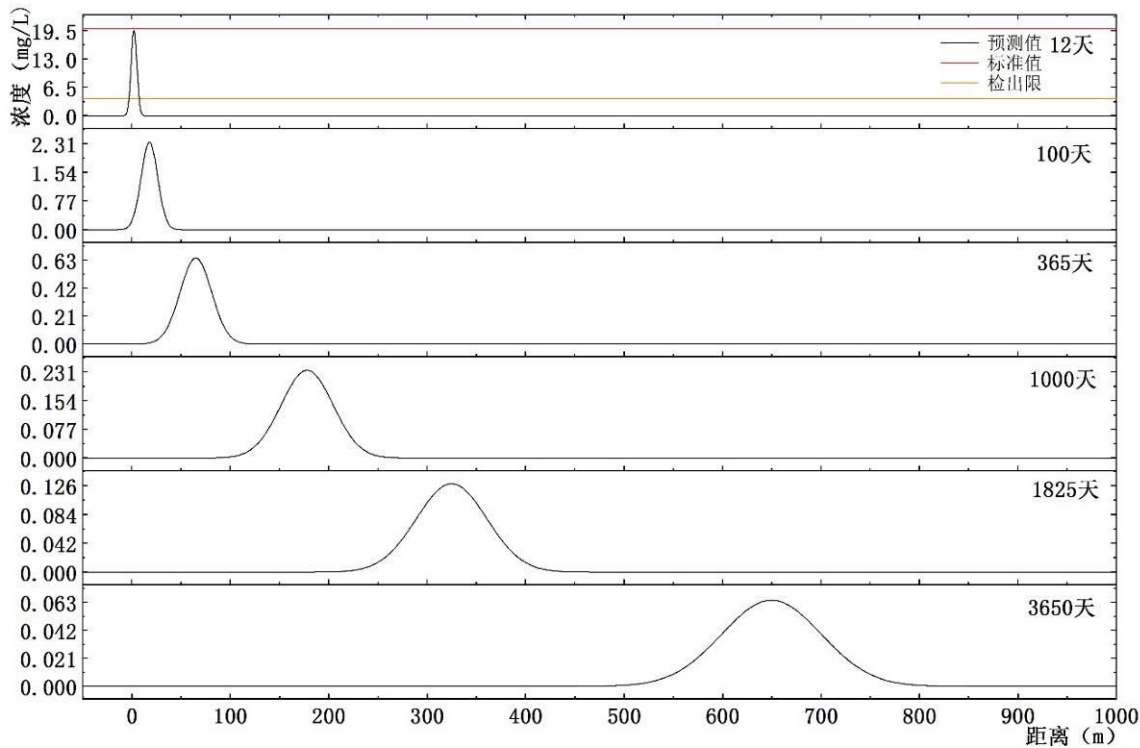
图 7.3-4 污染物 COD 距离与浓度关系曲线示意图
