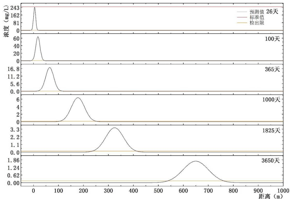
图 7.3-6 污染物氯化物距离与浓度关系曲线示意图
