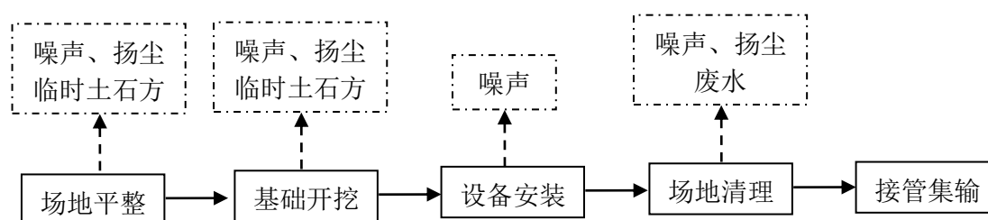
图 4.1-7 场站施工工序及产污环节示意图
