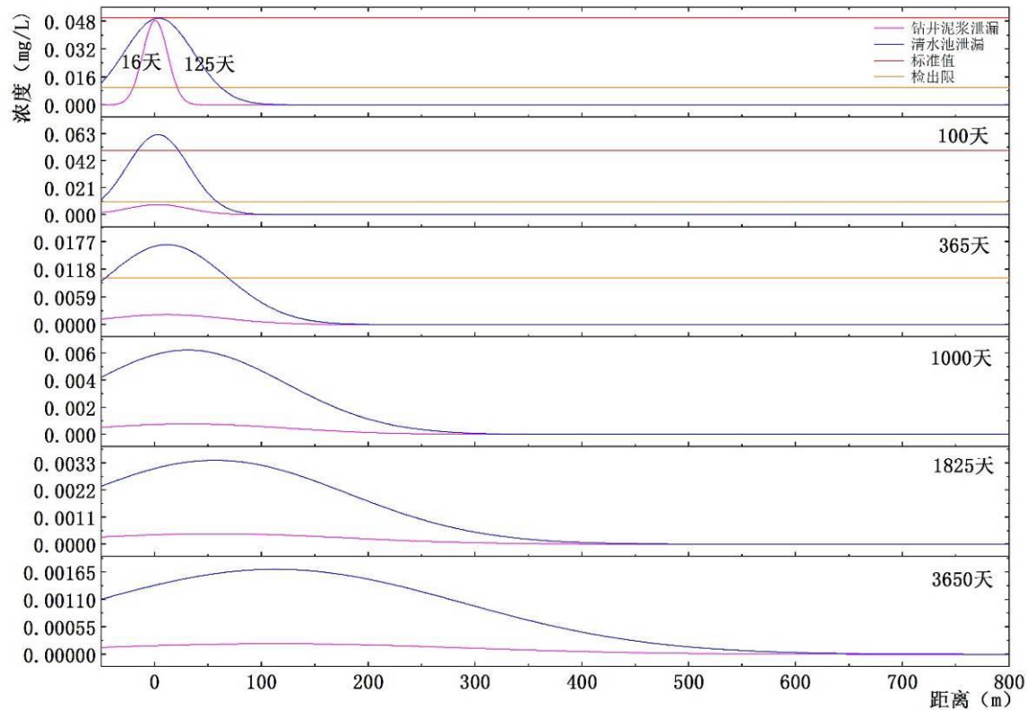
图 6.4-2 污染物石油类距离与浓度关系曲线示意图
