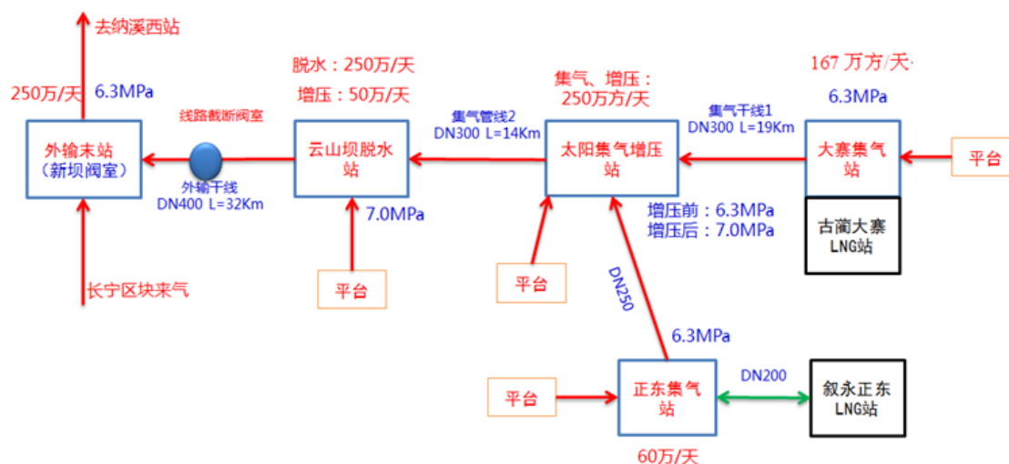
图2.2-1 太阳-大寨区块页岩气总体流程框图
