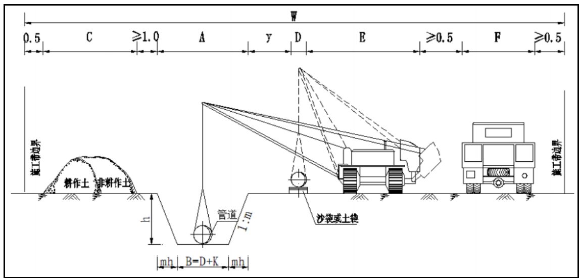
图 3.2-4 施工作业带示意图
