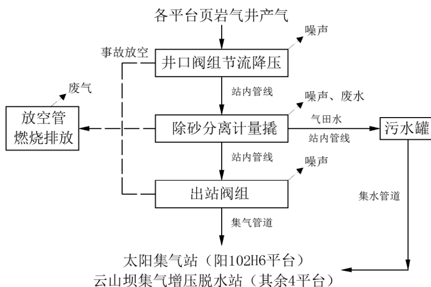
图 4.2-1 运营期生产工艺流程及产污环节示意图
