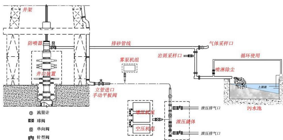
图 4.1-2 空气钻井水喷淋除尘示意图
