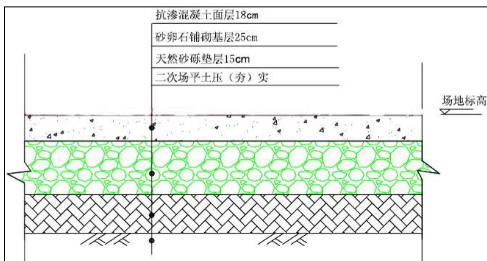
图9.5-4 一般防渗区地坪防渗结构示意图
