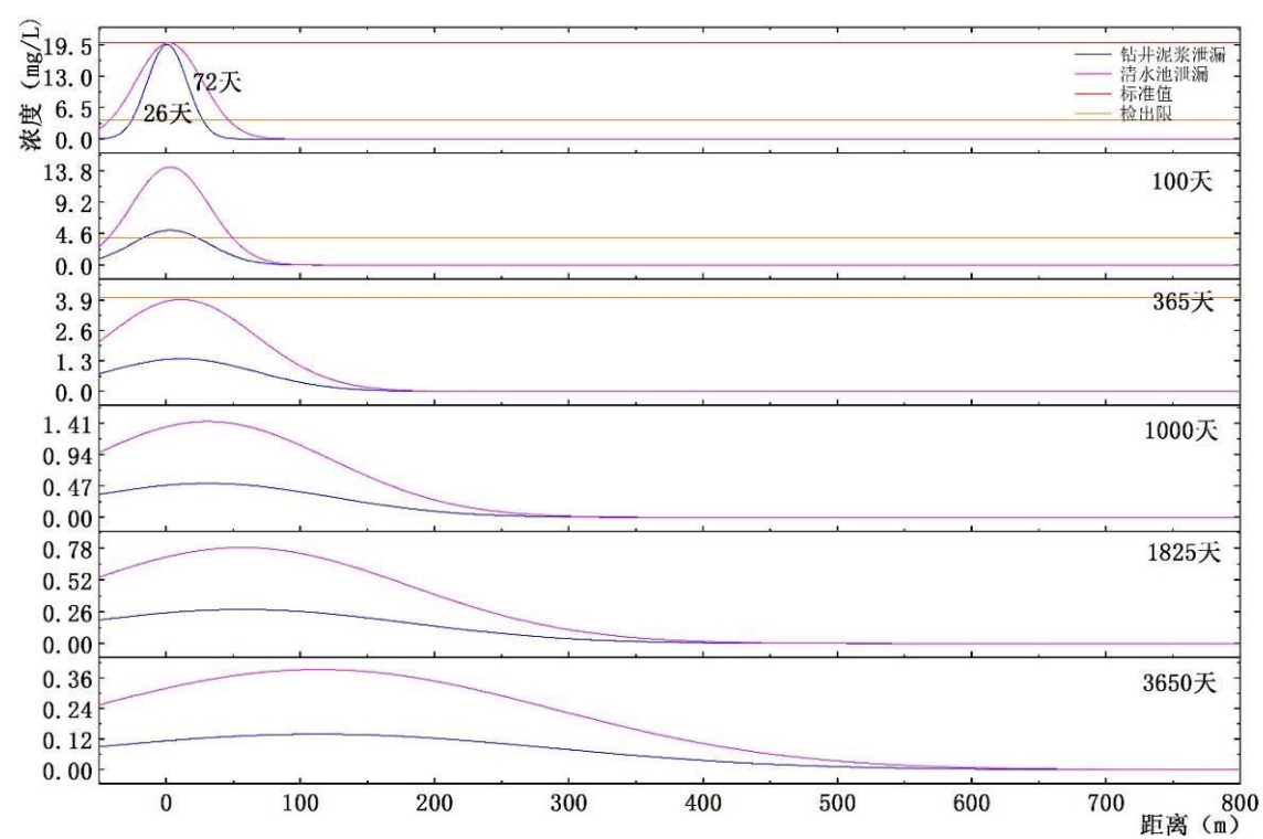
图 6.4-1 污染物 COD 距离与浓度关系曲线示意图
