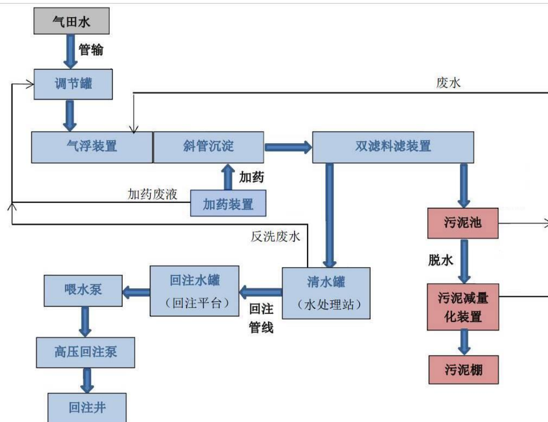
图 3.2-5 阳 1 井回注工程回注工艺流程示意图
