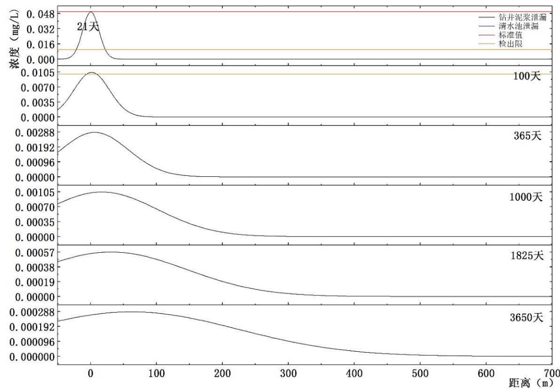
图 6.4-8 污染物石油类距离与浓度关系曲线示意图
