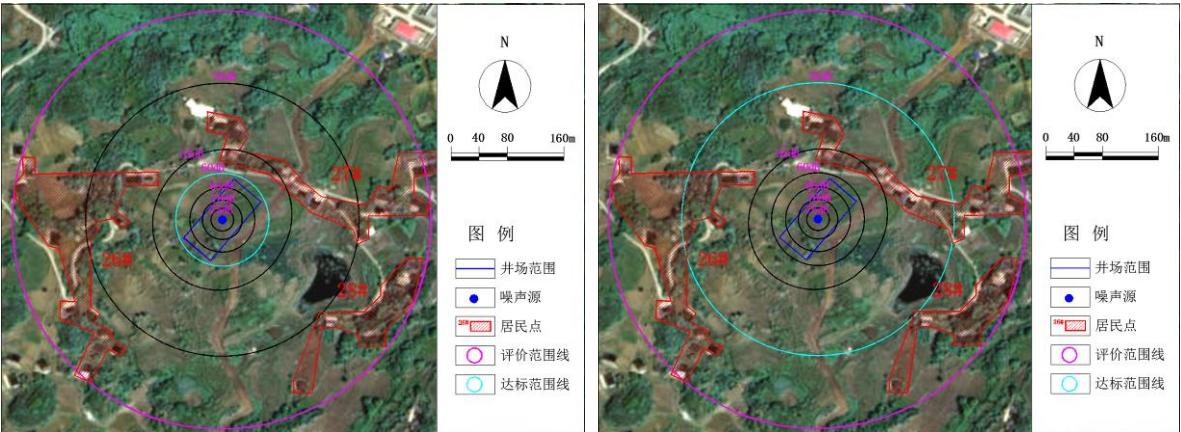
图 6.5-2 典型平台（阳 102H28）钻井期间噪声等值线图（停电情况）
