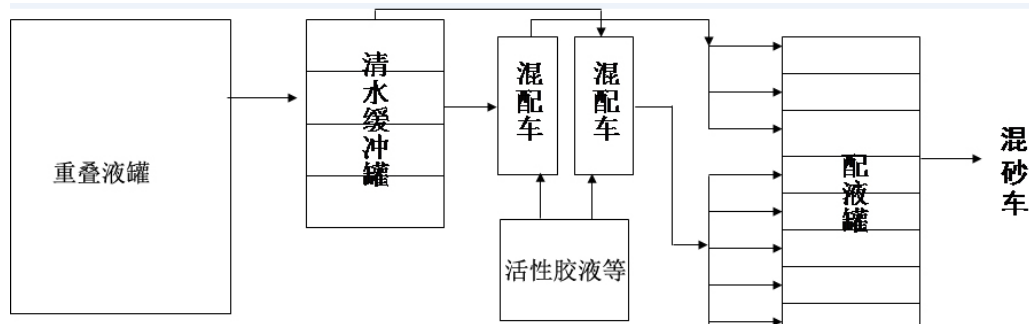
图 4.1-6 压裂液连续混配工艺流程示意图
