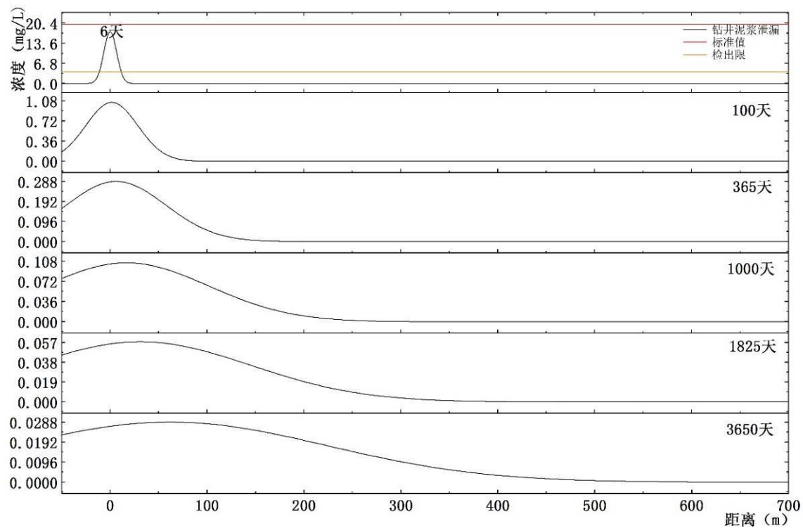
图 6.4-7 污染物 COD 距离与浓度关系曲线示意图
