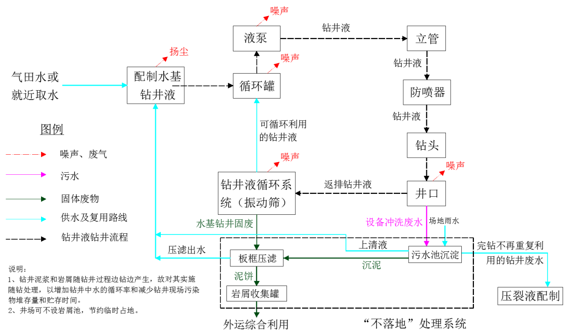
图 4.1-3 清水及水基泥浆钻井工艺流程及产排污环节图
