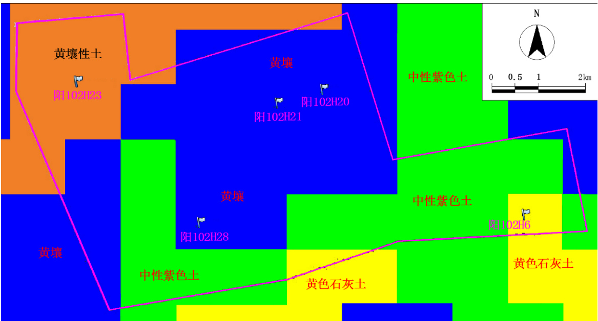
图 5.3-2 井区内土壤类型分布情况图
