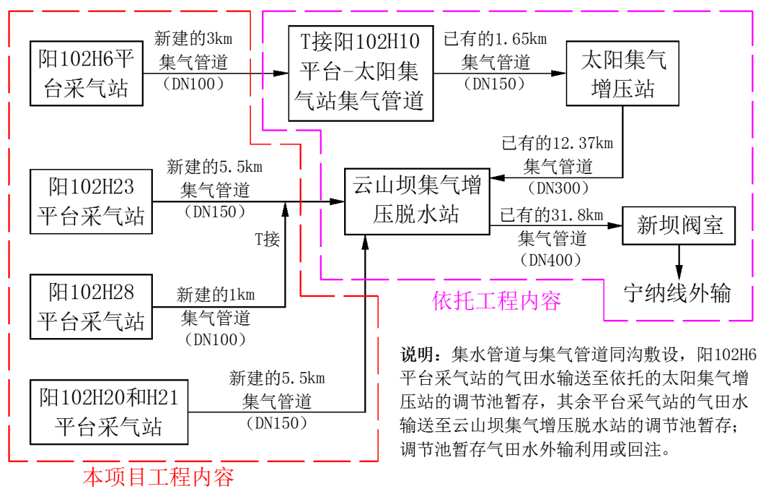
图 3.2-3 阳 102 井区集气及集水流程示意图
