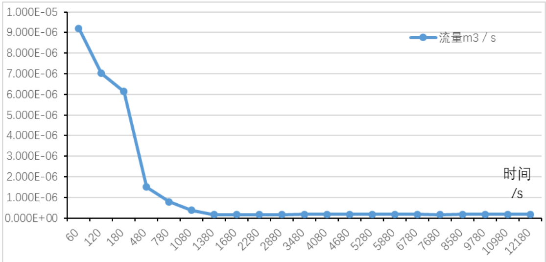
T2 渗水试验 Q—t 曲线图
