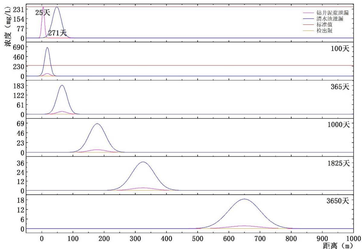
图 6.4-6 污染物氯化物距离与浓度关系曲线示意图
