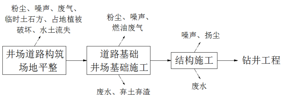
图 4.1-1 钻前工程施工过程及主要环境影响
