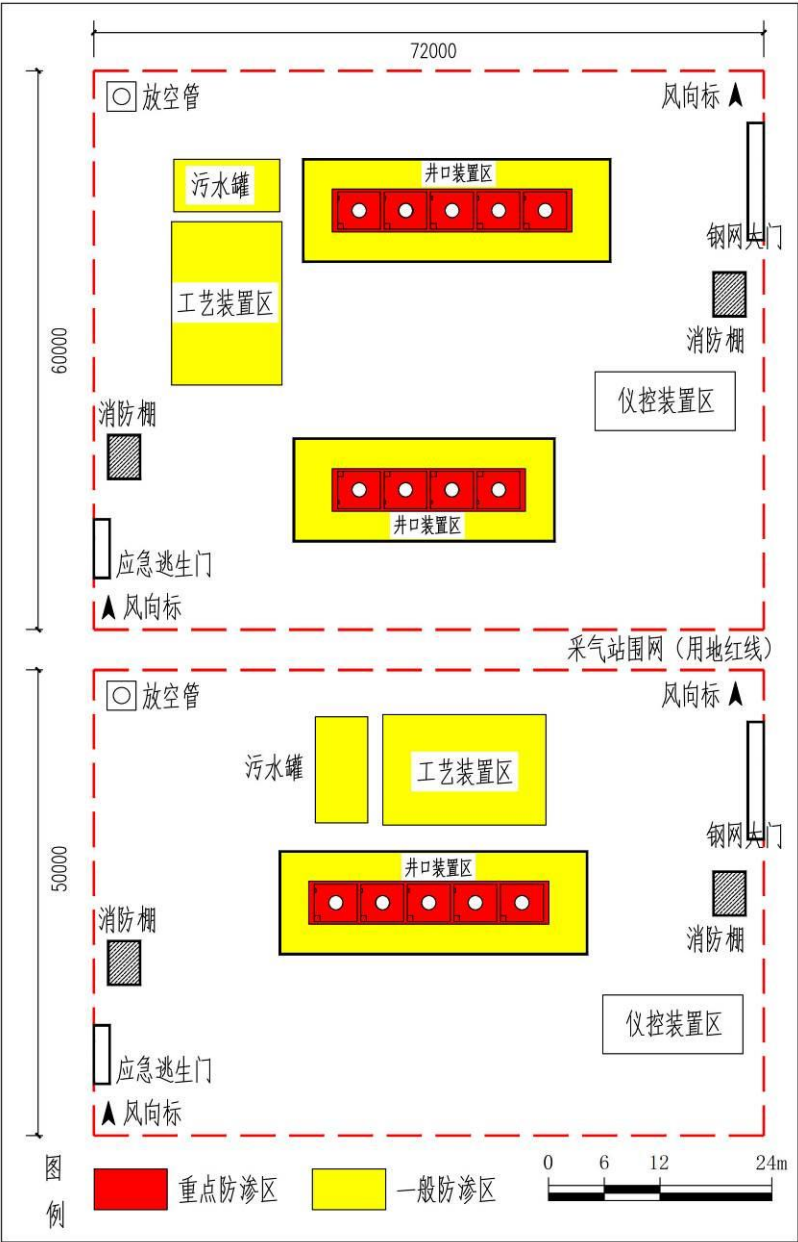
图 9.5-2 运营期典型井站分区防渗划分示意图
