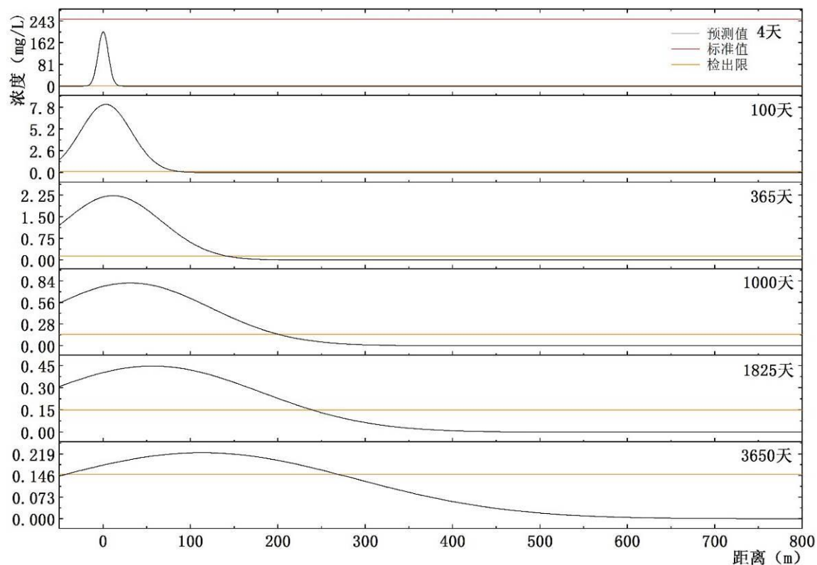
图 7.3-3 污染物氯化物距离与浓度关系曲线示意图
