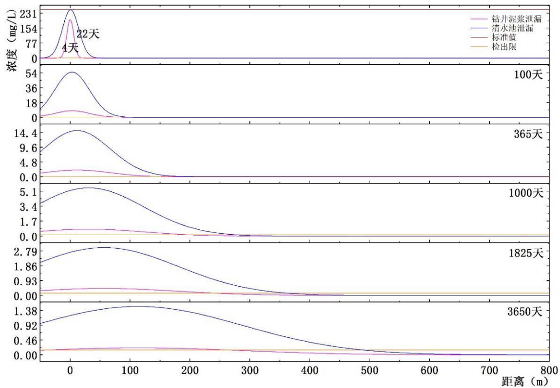
图 6.4-3 污染物氯化物距离与浓度关系曲线示意图
