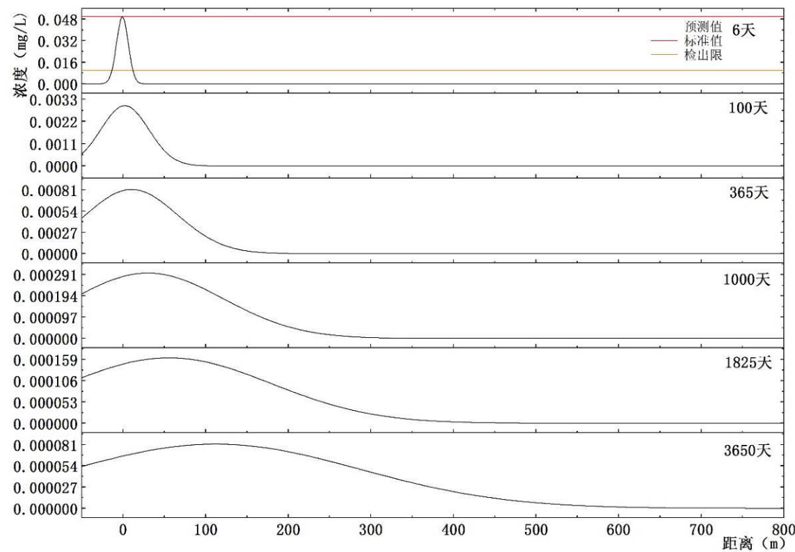
图 7.3-2 污染物石油类距离与浓度关系曲线示意图
