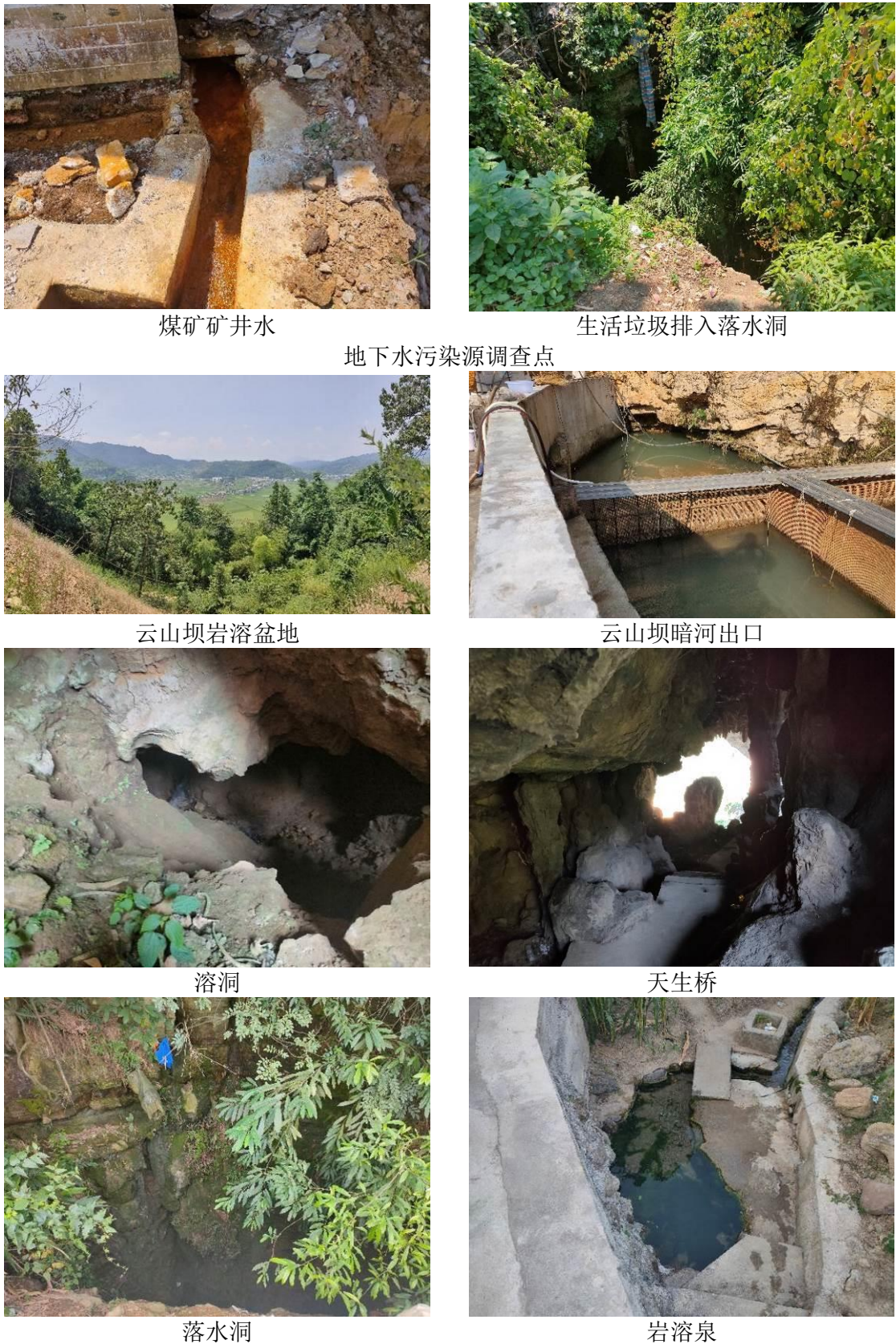
岩溶发育情况调查点
