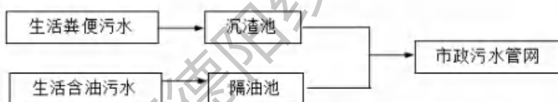
图 6.4.2-3 生活污水处理工艺流程图
