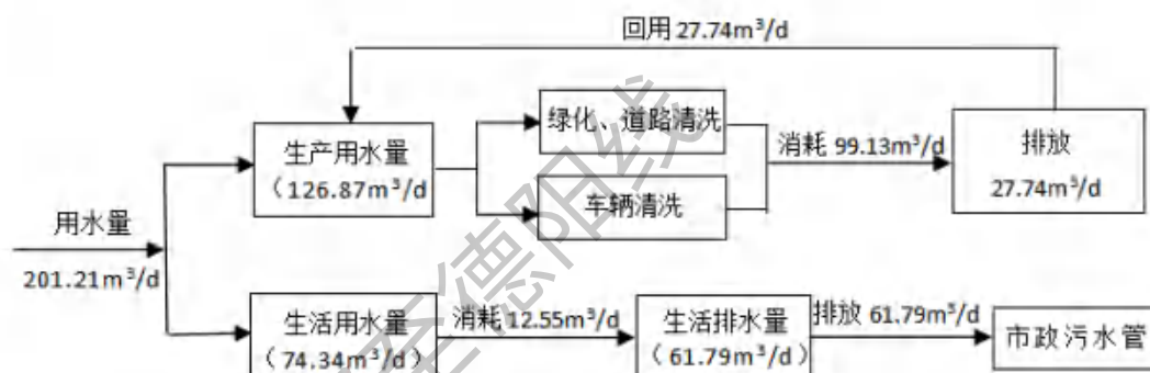
图 6.4.2-1 凤凰山停车场水平衡图
