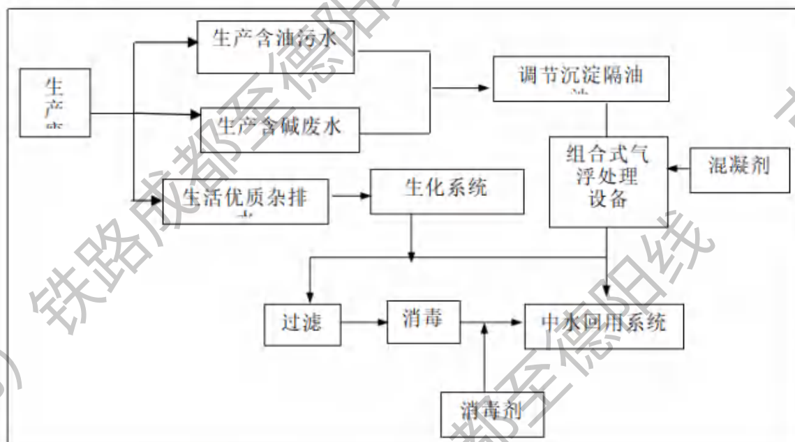
图 6.4.2-4 德阳北车辆段废水处理工艺
