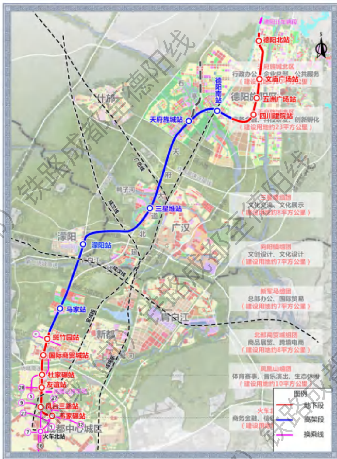
市域（郊）铁路成都至德阳线工程线路平面示意图
