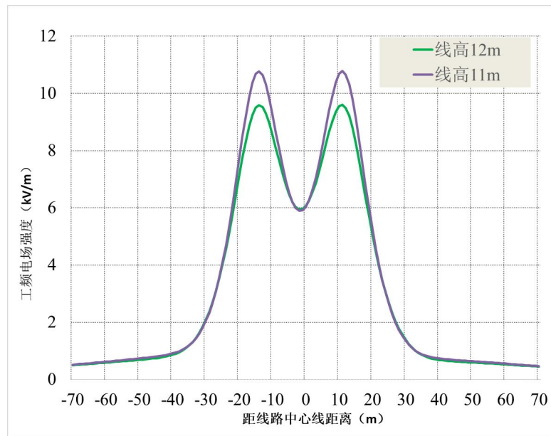
图 6-4 线路同塔双回排列段通过耕地、园地、牧草地、畜禽饲养地、养殖水面、道路等场所最不利塔型电场强度随距离变化趋势图
