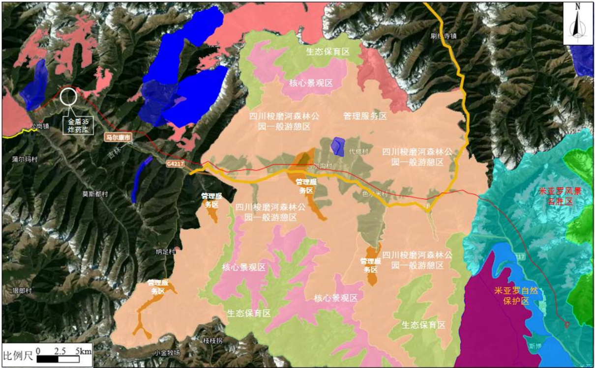
图 3-9 巴拉水电站～马尔康 500 千伏线路改接工程路径方案示意图
