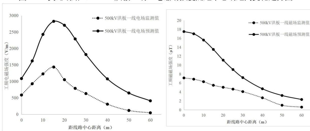
图 6-3 类比线路（500kV 洪板一线）电磁场强度随距中心线距离变化趋势图
