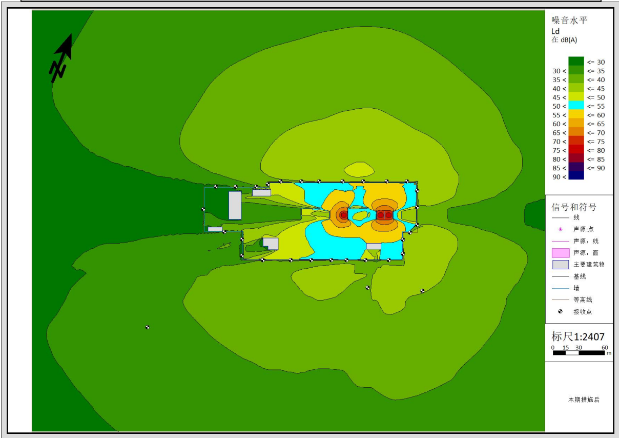
图 6-18 马尔康 500kV 变电站本期采取降噪措施后噪声预测（贡献值）等声级线图
