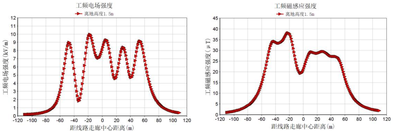
图 6-15 同塔双回路线路与单回路线路并行段工频电磁场预测结果分布曲线
