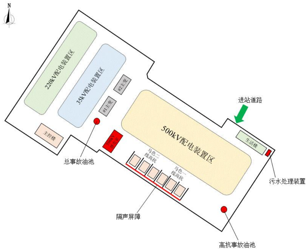
图 3-5 色尔古变电站前期工程主要环保设施布置图
