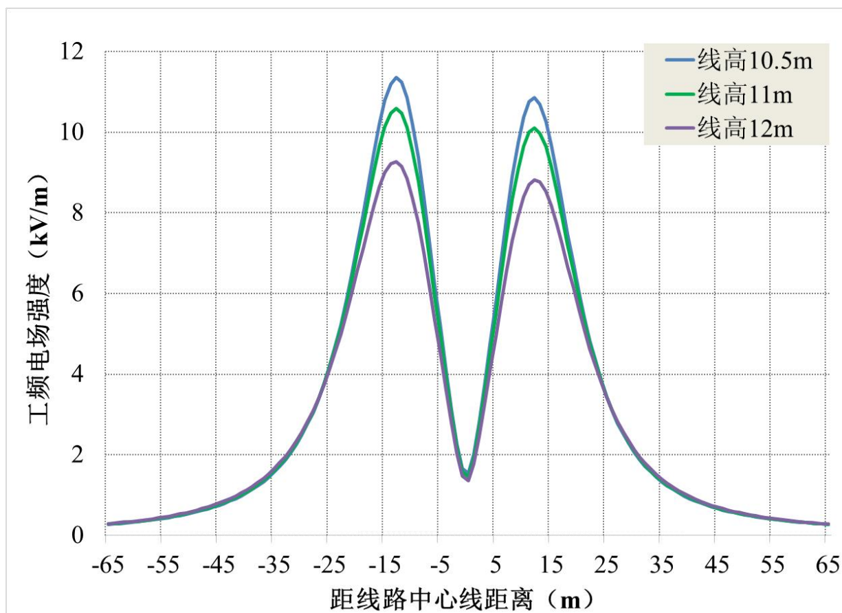
图 6-6 线路单回三角排列段通过耕地、园地、牧草地、畜禽饲养地、养殖水面、道路等场所最不利塔型电场强度随距离变化趋势图
