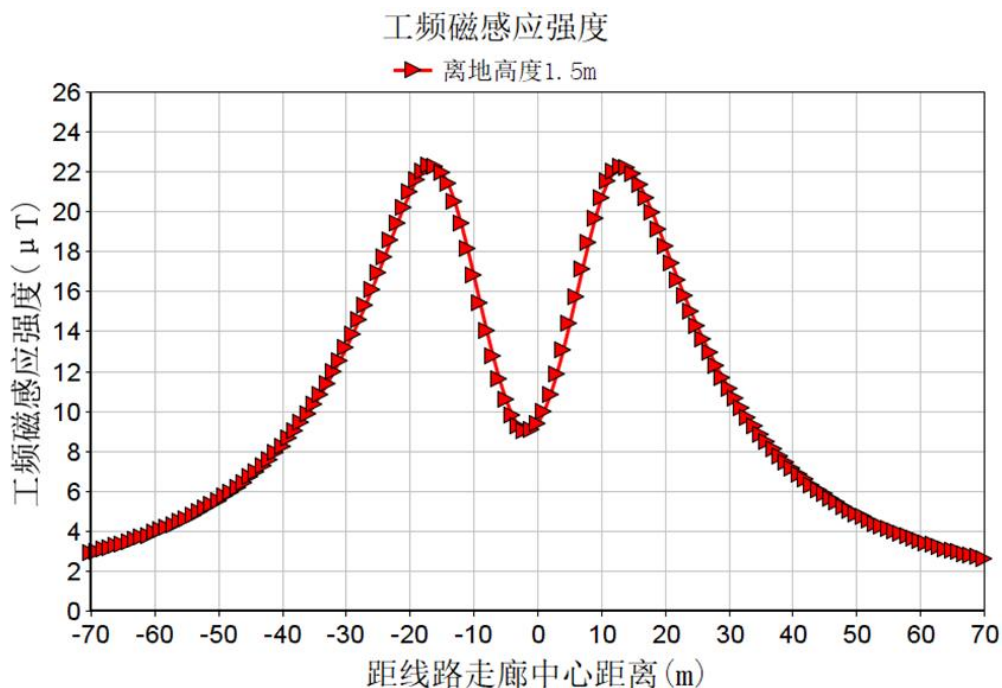
图 6-5 同塔双回排列段导线通过耕地、园地、牧草地、畜禽饲养地、养殖水面、道路等场所最不利塔型工频磁感应强度分布曲线
