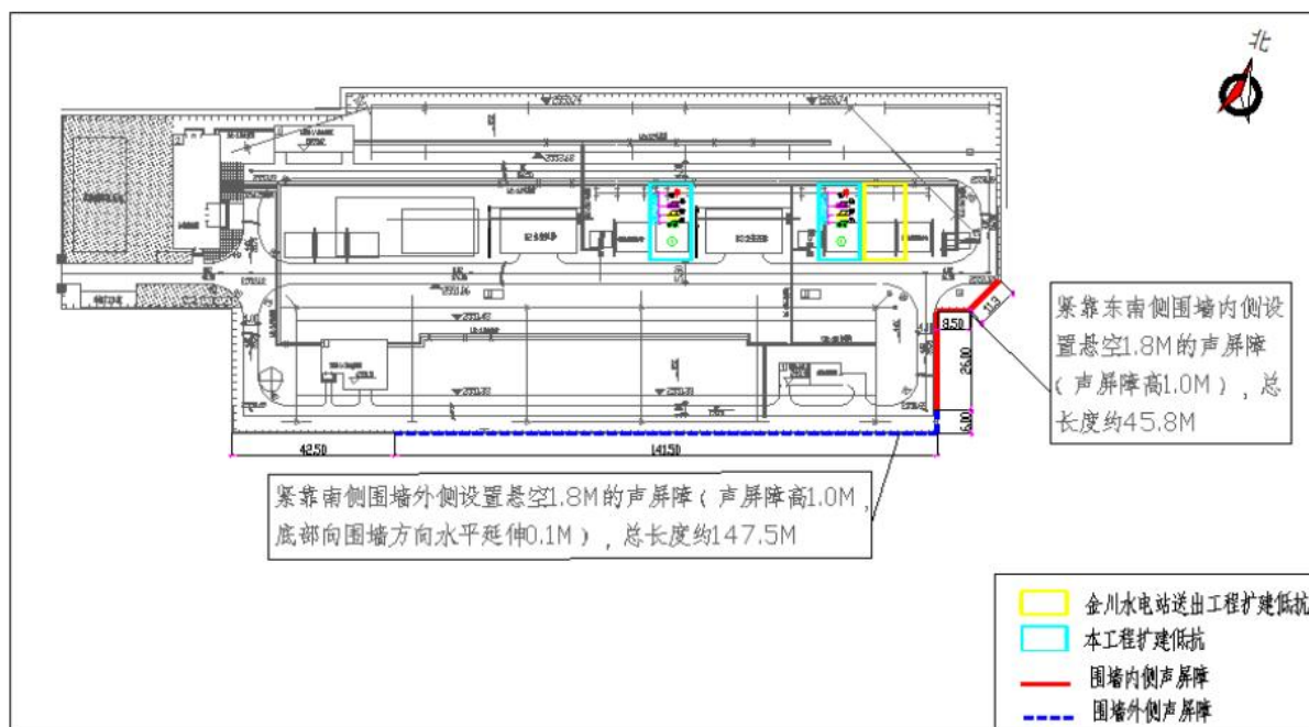
图 6-17 马尔康 500kV 变电站站前期工程及本次扩建降噪措施示意图
