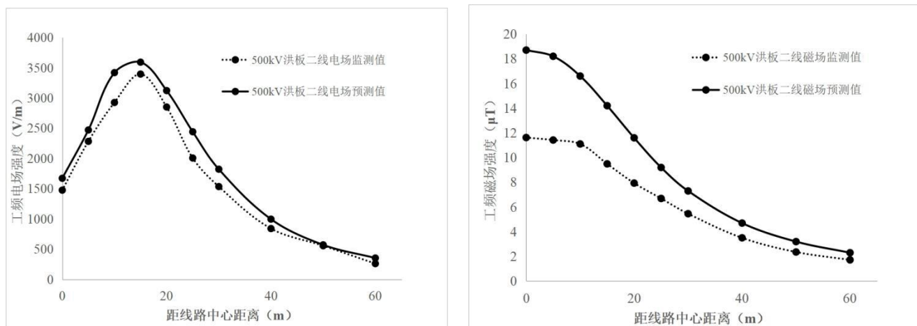
图 6-2 类比线路（500kV 洪板二线）电磁场强度随距中心线距离变化趋势图
