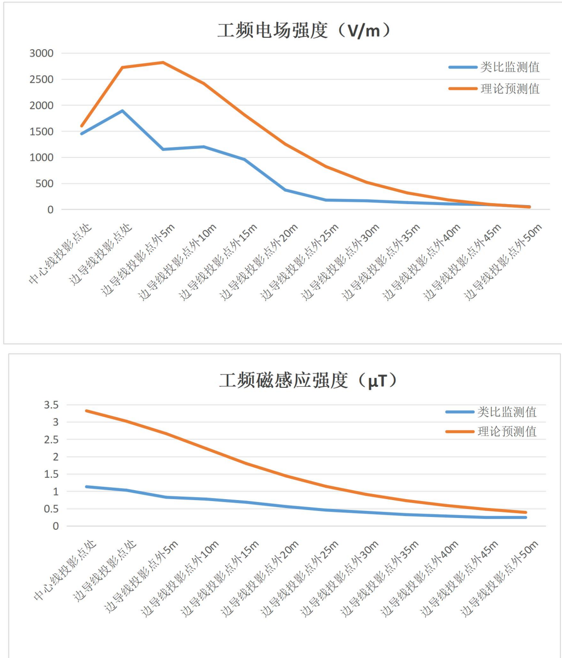
图6-1 类比线路(500kV瀑布沟电站一东坡I、II回线路)电磁场强度随距中心线距离变化趋势图
