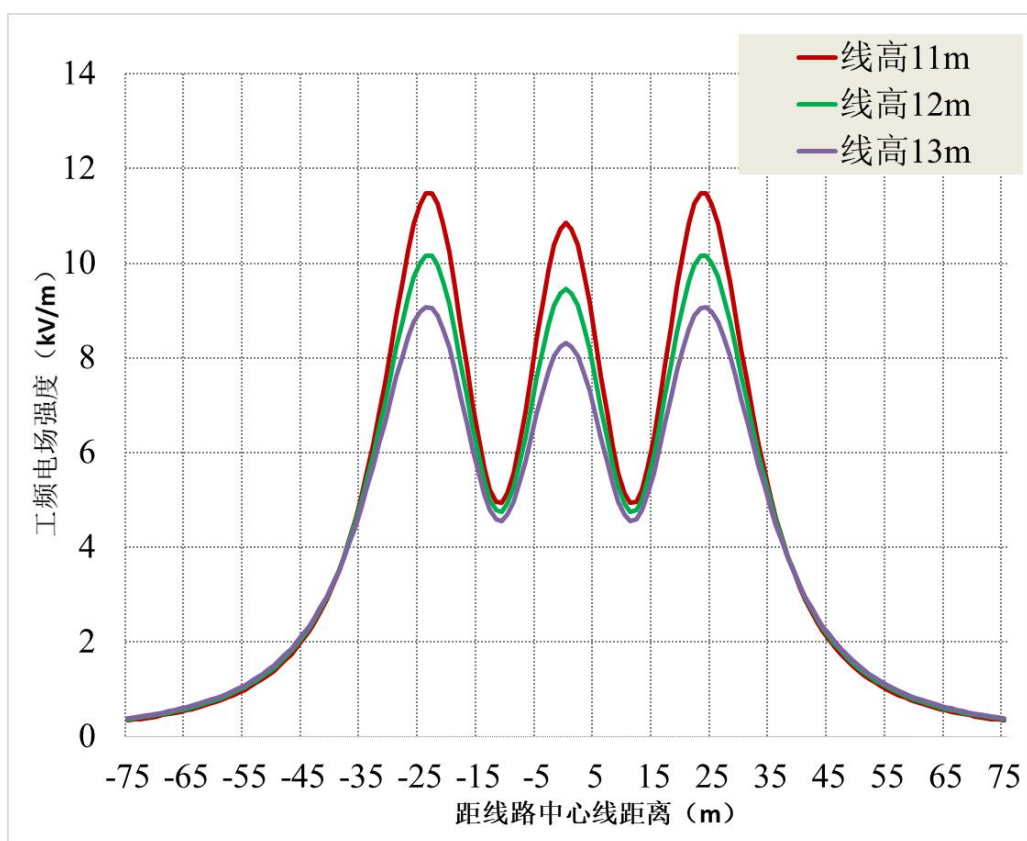
图 6-9 线路单回水平排列段通过耕地、园地、牧草地、畜禽饲养地、养殖水面、道路等场所最不利塔型电场强度随距离变化趋势图
