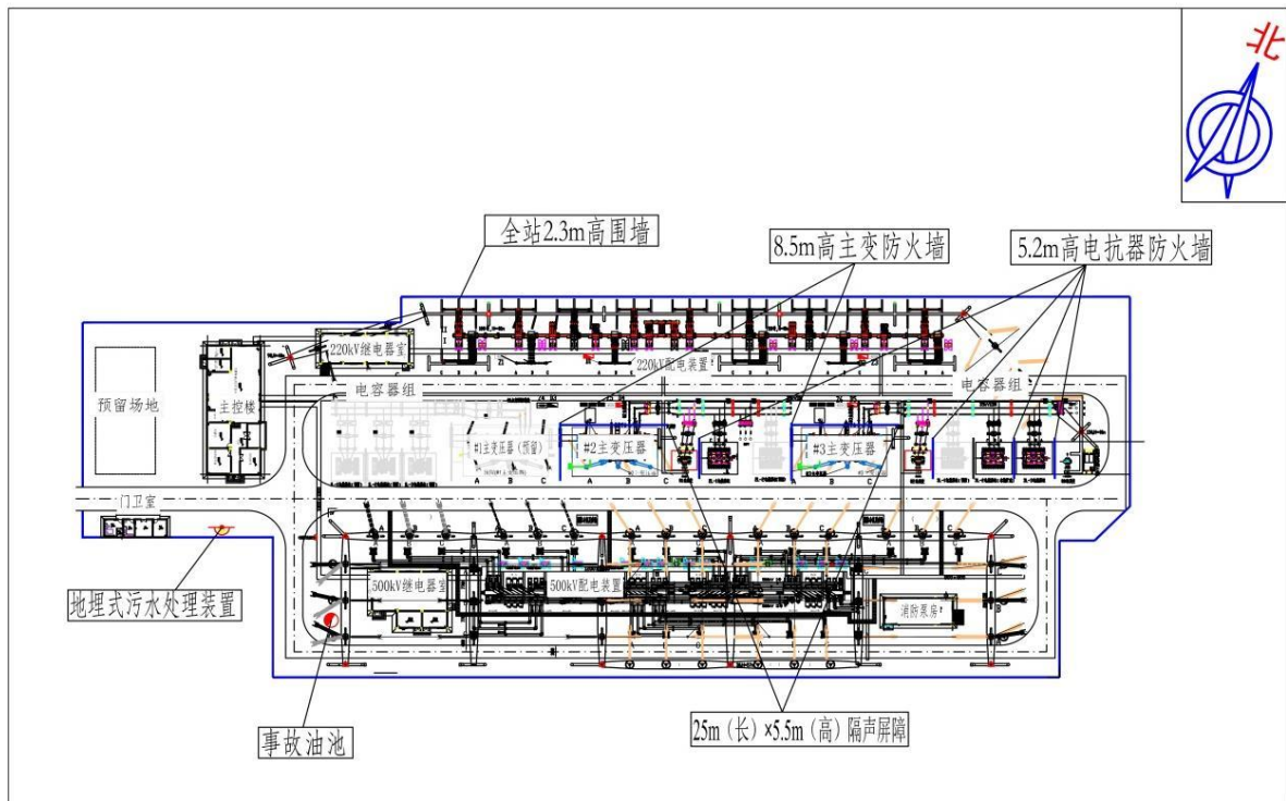
图 3-3 马尔康变电站前期工程主要环保设施布置图
