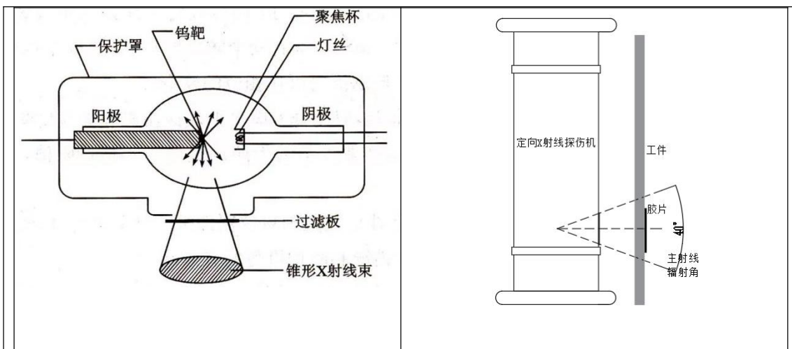
图 9-2 典型的 X 射线管结构图及常见 X 射线探伤机照射工件示意图
