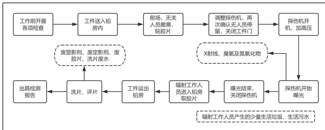
图9-3 本项工作流程及产污环节示意图
