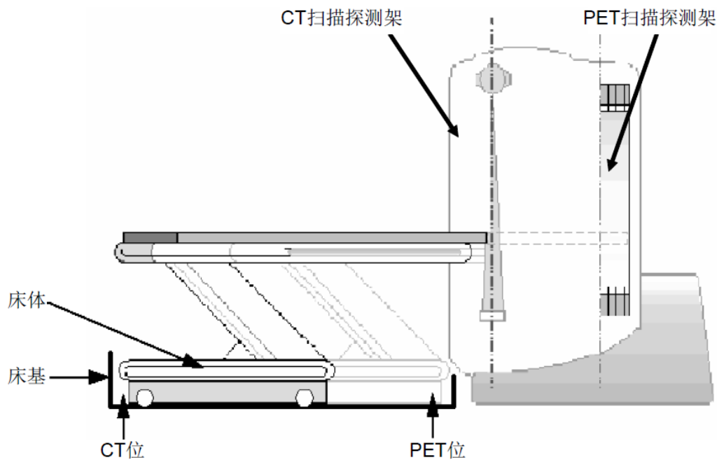
图 9-7 PET/CT 结构示意图
