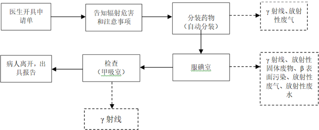
图 9-12 131 I 甲状腺吸碘功能测定项目工作流程及产污环节分析示意图
