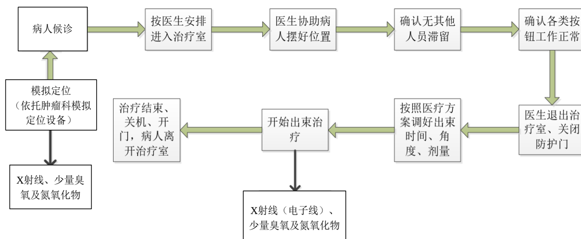
图 9-3 医用电子直线加速器放疗流程及产污环节示意图
