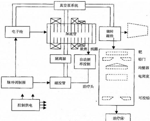
图 9-2 医用电子直线加速器系统示意图
