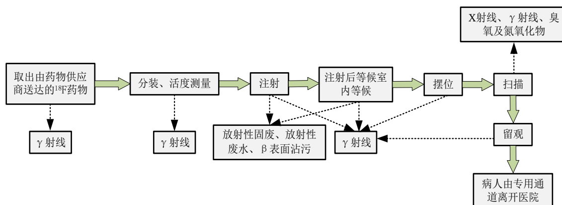
图 9-10 本项目核医学诊断流程及产污环节示意图
