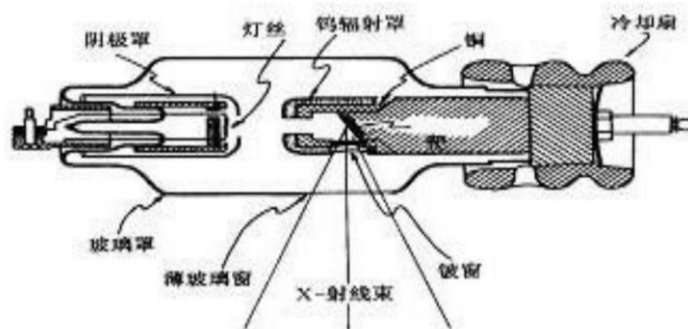
图 9-4 X 射线管基本结构示意图
