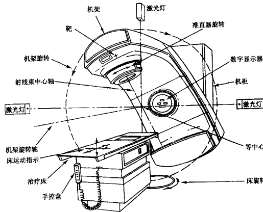
图 9-1 典型医用电子直线加速器基本结构示意图
