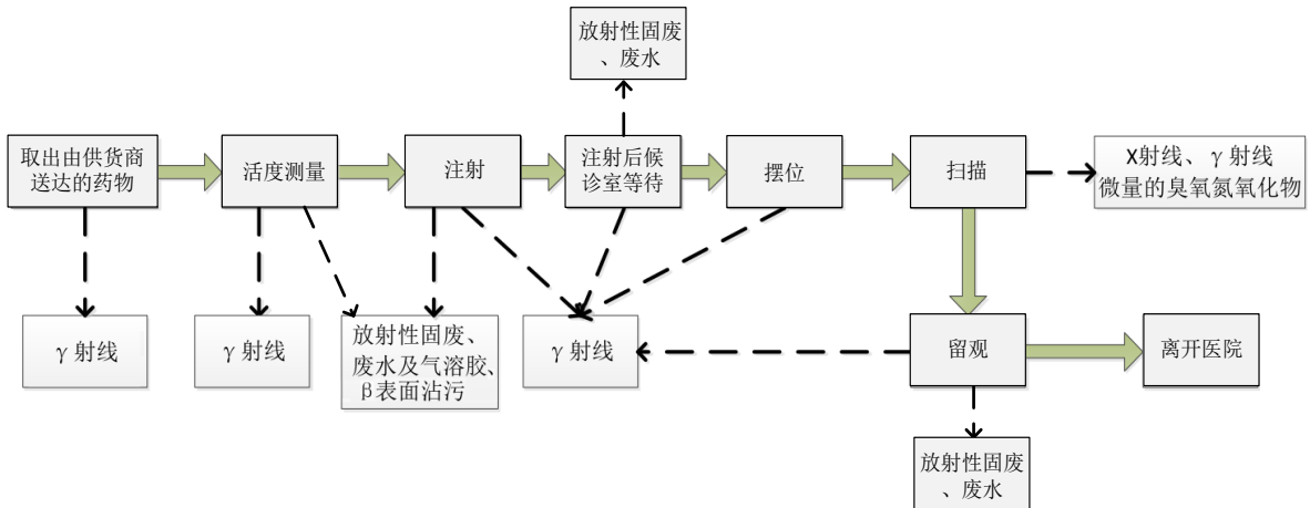
图 9-11 SPECT/CT 诊断项目工作流程及产污环节分析示意图
