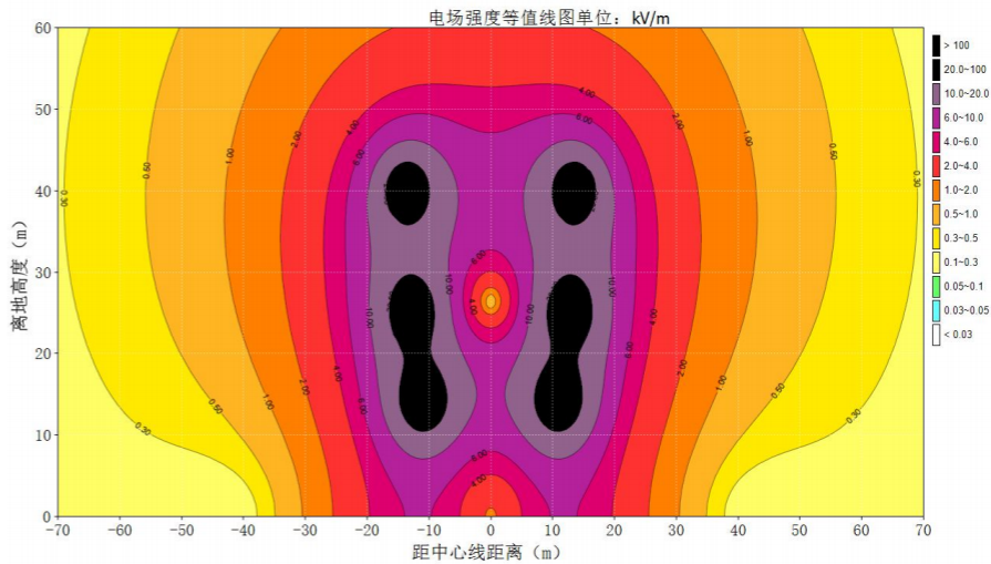
图 6-7 线高 14m 时电场强度等值线图
