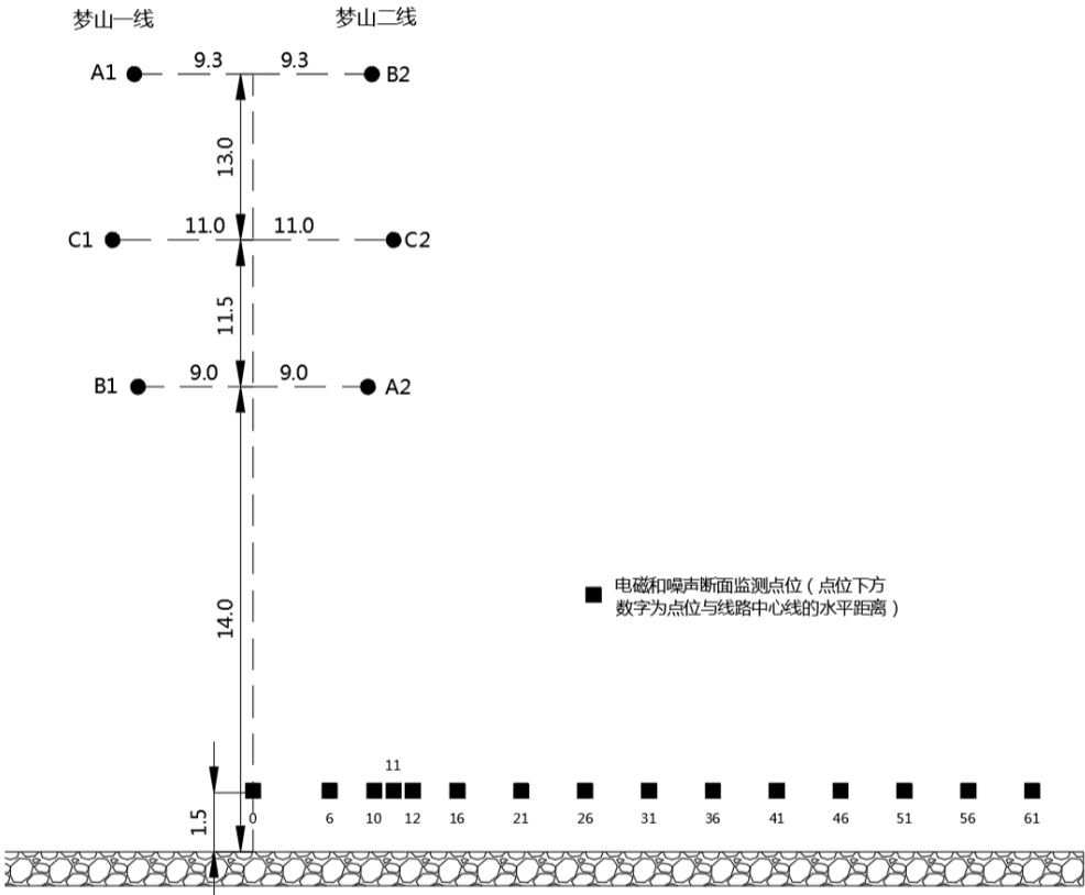
图 4-2 本次改造线路监测断面布点情况
