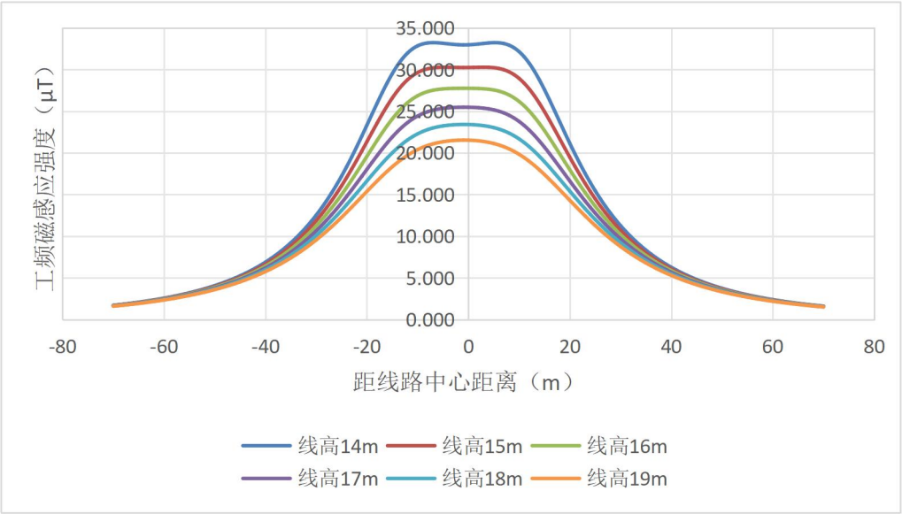
图 6-56 线路在公众曝露区磁感应强度随距离变化趋势图（距地面 1.5m 高处）
