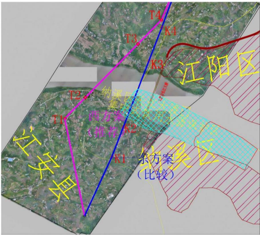
图 3-12 长江跨越点方案比选
