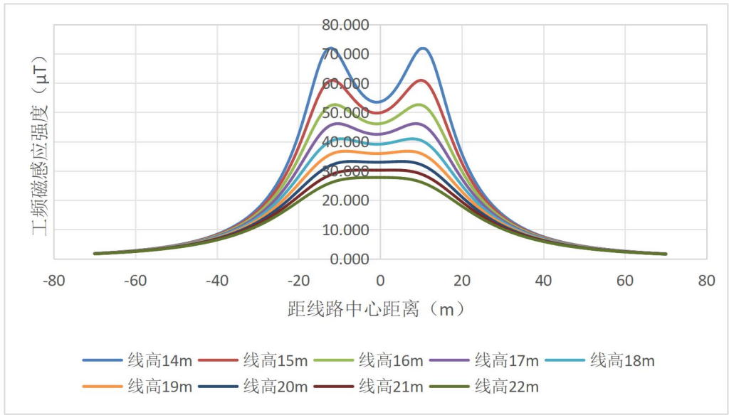
图 6-58 线路在公众曝露区磁感应强度随距离变化趋势图（距地面 7.5m 高处）
