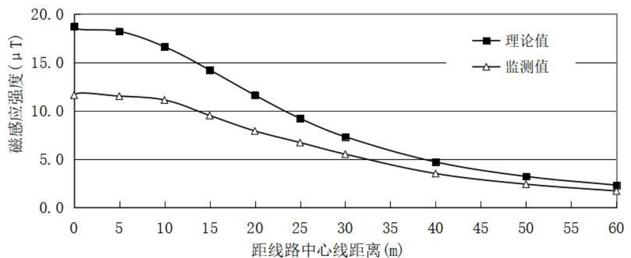
图 6-64 类比线路（500kV 洪板二线）磁感应强度随距中心线距离变化趋势图
