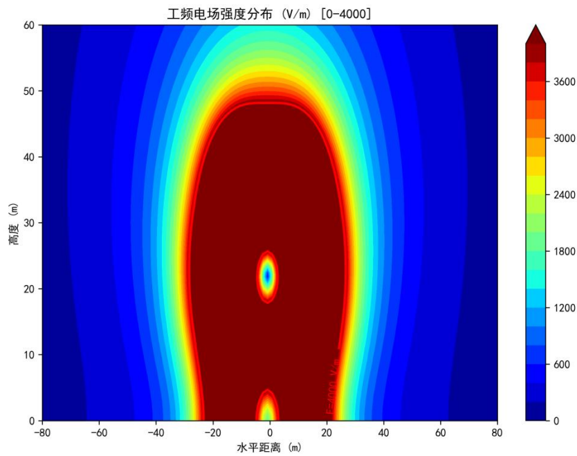
图 6-53 同塔双回长江跨越段对地高度 11m 的电场强度等值线图（单位：kV/m）
