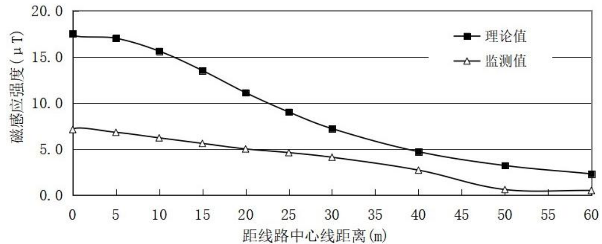
图 6-62 类比线路（500kV 洪板一线）磁感应强度随距中心线距离变化趋势图
