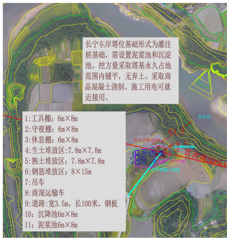
图 3-6 长宁河跨越东岸施工布置图
