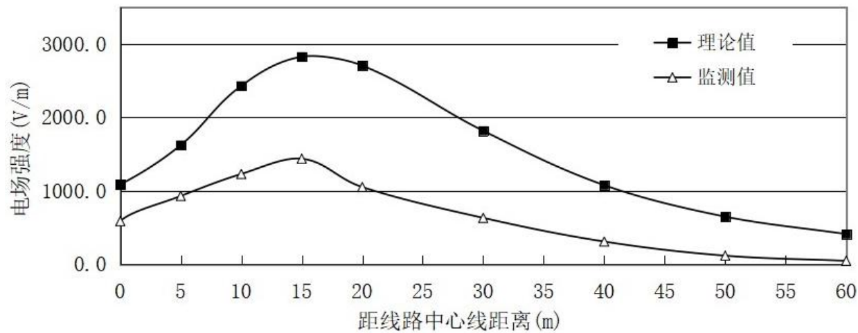
图 6-61 类比线路（500kV 洪板一线）电场强度随距中心线距离变化趋势图
