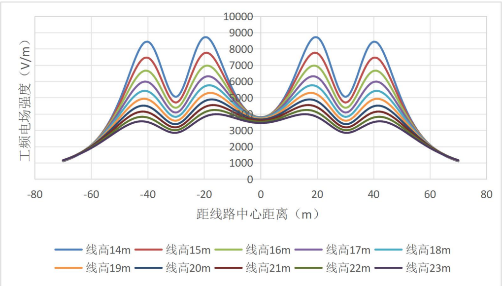
图 6-27 线路在公众暴露区电场强度随距离变化趋势图（距地面 4.5m 高处）
