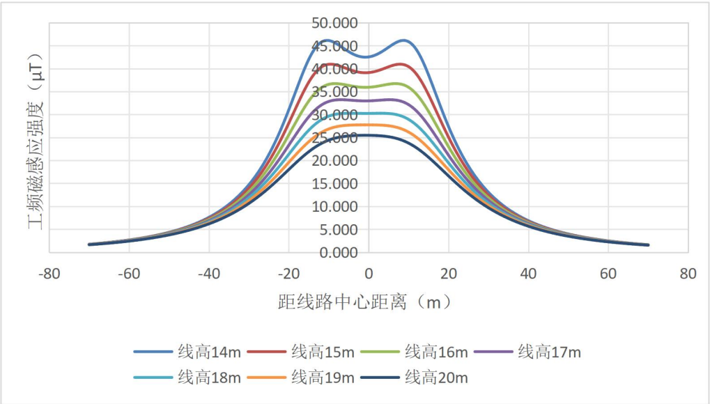
图 6-57 线路在公众曝露区磁感应强度随距离变化趋势图（距地面 4.5m 高处）
