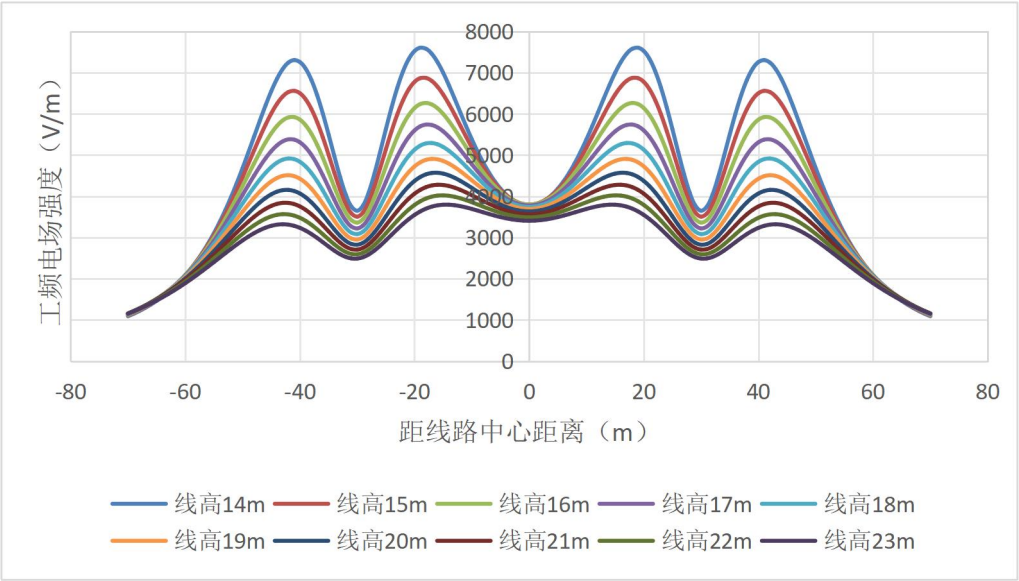
图 6-26 线路在公众暴露区电场强度随距离变化趋势图（距地面 1.5m 高处）
