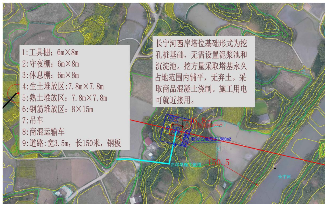
图 3-5 长宁河跨越西岸施工布置图
