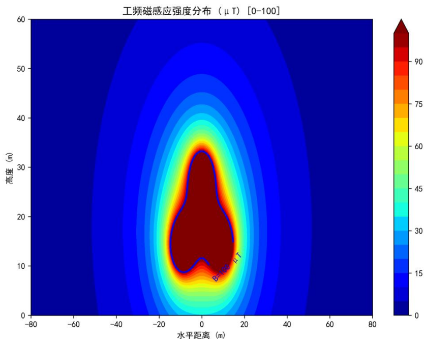
图 6-24 单回三角段对地高度 14m 的磁感应强度等值线图
