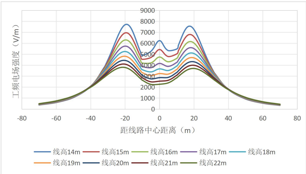
图 6-4 线路在公众曝露区电场强度随距离变化趋势图（距地面 1.5m 高处）
