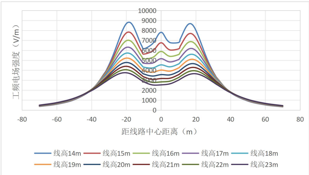
图 6-5 线路在公众曝露区电场强度随距离变化趋势图（距地面 4.5m 高处）
