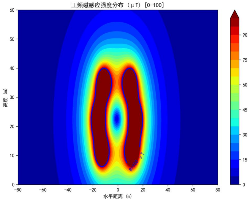
图 6-59 同塔双回长江跨越段对地高度 11m 的磁感应强度等值线
