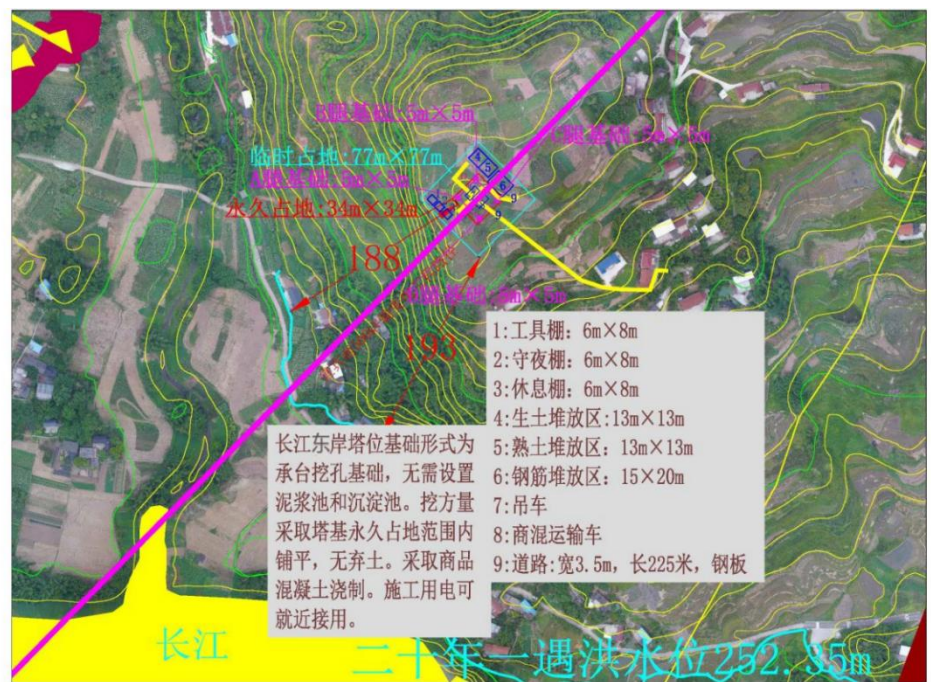
图 3-4 长江跨越东岸施工布置图
