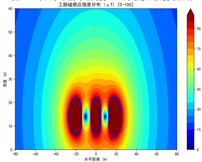
图 6-12 单回水平段对地高度 14m 的磁感应强度等值线
