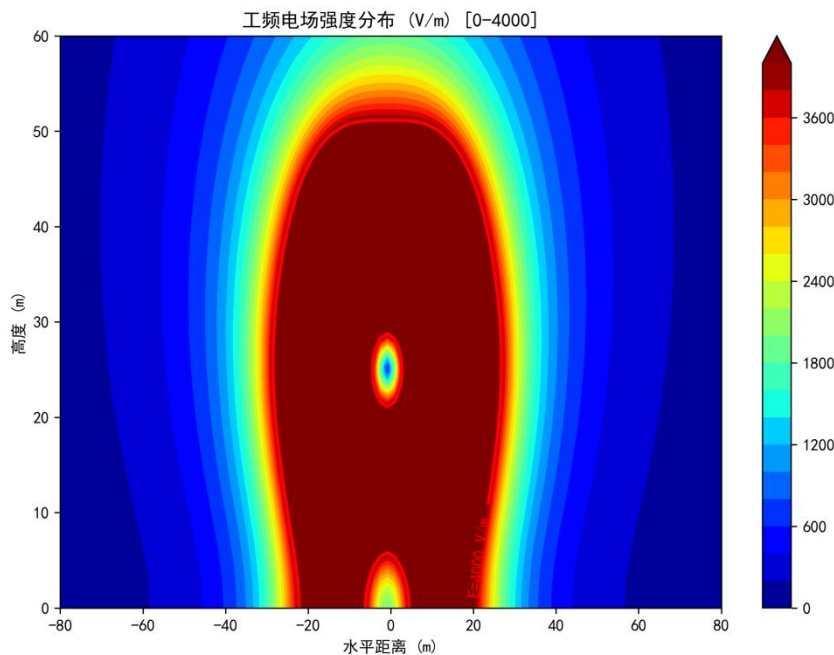
图 6-54 同塔双回长江跨越段对地高度 14m 的电场强度等值线图（单位：kV/m）
