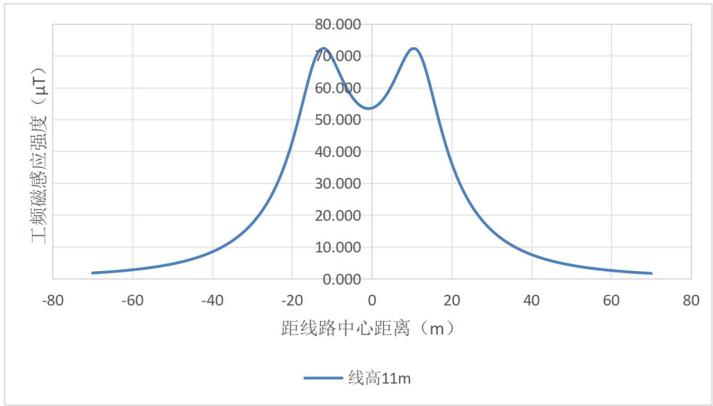
图 6-55 本段线路通过耕地、园地等场所最不利塔型磁感应强度随距离变化趋势图
