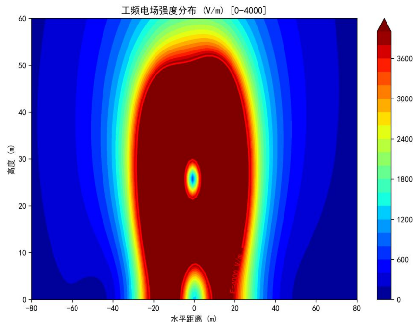
图 6-42 同塔双回路对地高度 14m 的电场强度等值线图（单位：kV/m）
