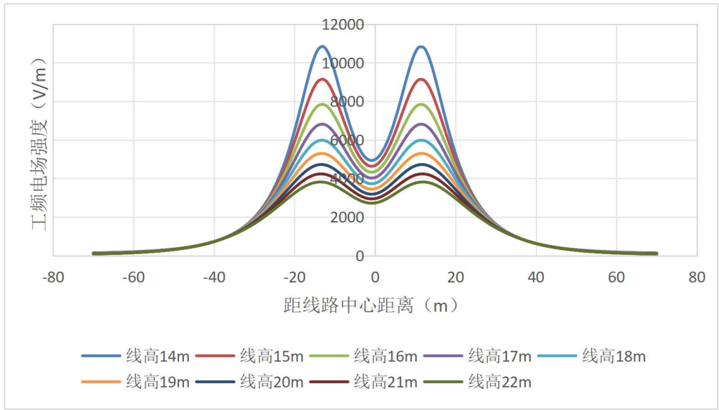
图 6-52 线路在公众曝露区电场强度随距离变化趋势图（距地面 7.5m 高处）
