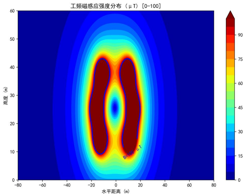
图 6-60 同塔双回长江跨越段对地高度 14m 的磁感应强度等值线
