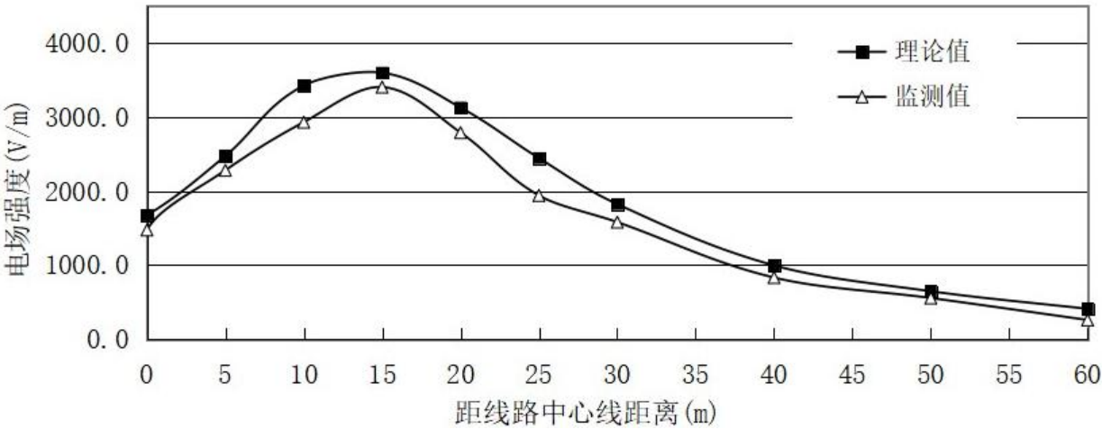
图 6-63 类比线路（500kV 洪板二线）电场强度随距中心线距离变化趋势图
