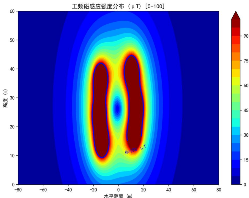
图 6-48 同塔双回路对地高度 14m 的磁感应强度等值线
