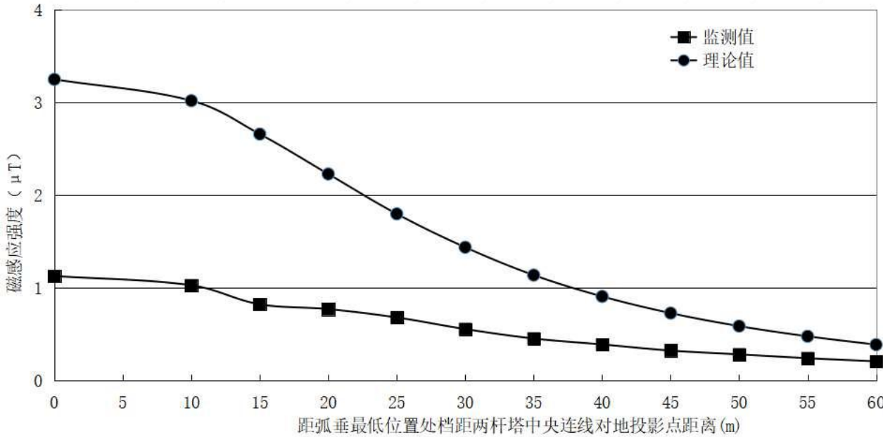
图 6-66 类比线路（瀑布沟电站-东坡一、二回线）磁感应强度随距中心线距变化图
