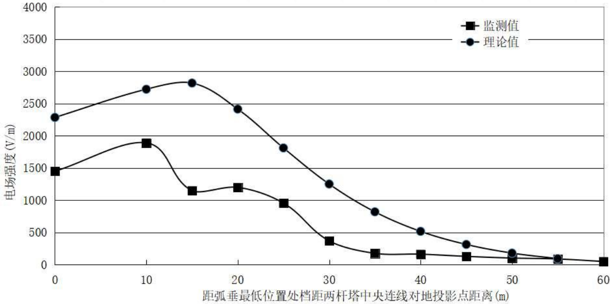
图 6-65 类比线路（瀑布沟电站-东坡一、二回线）电场强度随距中心线距变化趋势图
