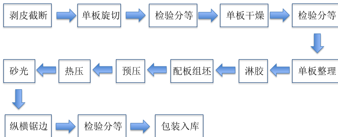
图 1 生产工艺流程图
