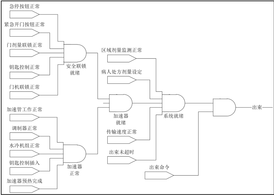
图 10-4 医用电子直线加速器联锁关系图
