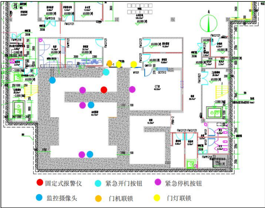
图 10-3 本项目辐射安全设施布置图
