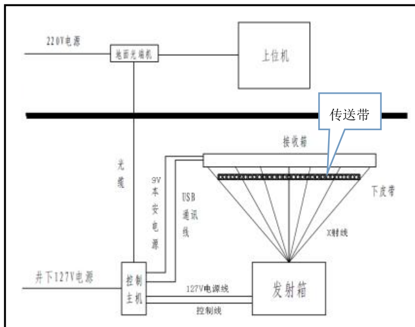
图 9-1 装置的布置及连接关系图
