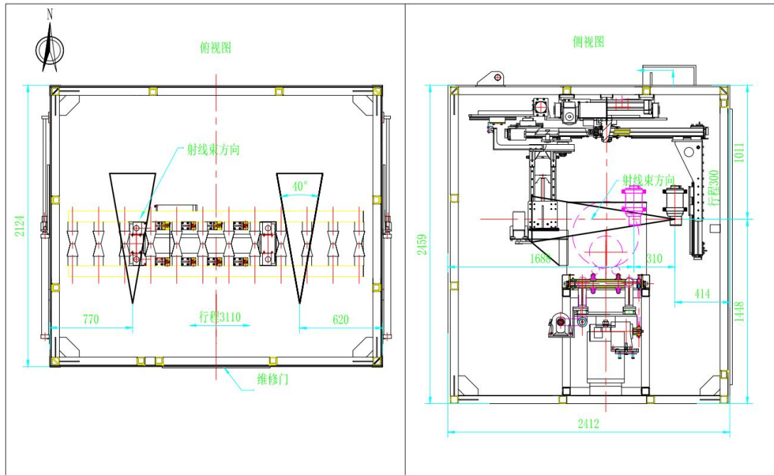
图 11-1 探伤机焦点运动范围及有用线束照射范围示意图
