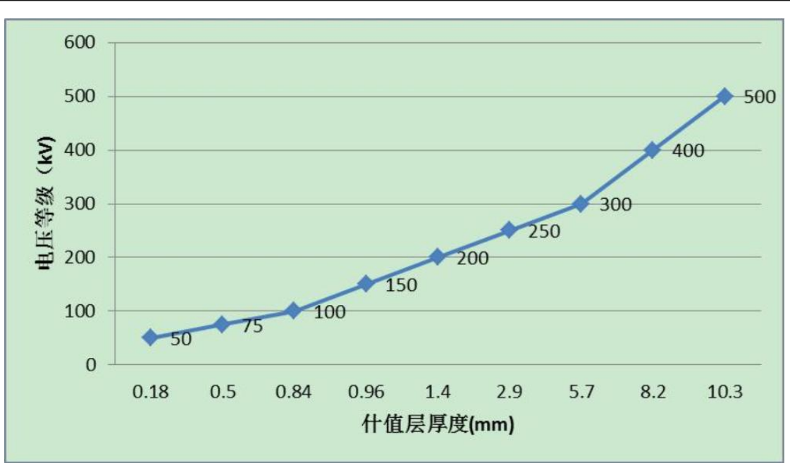
图11-2 不同电压X射线在铅中的半值层厚度相对关系
