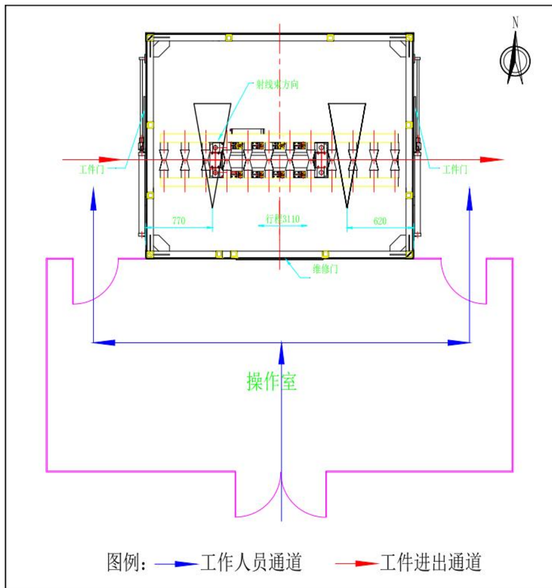
图 9-3 本项目工件及人员通道图
