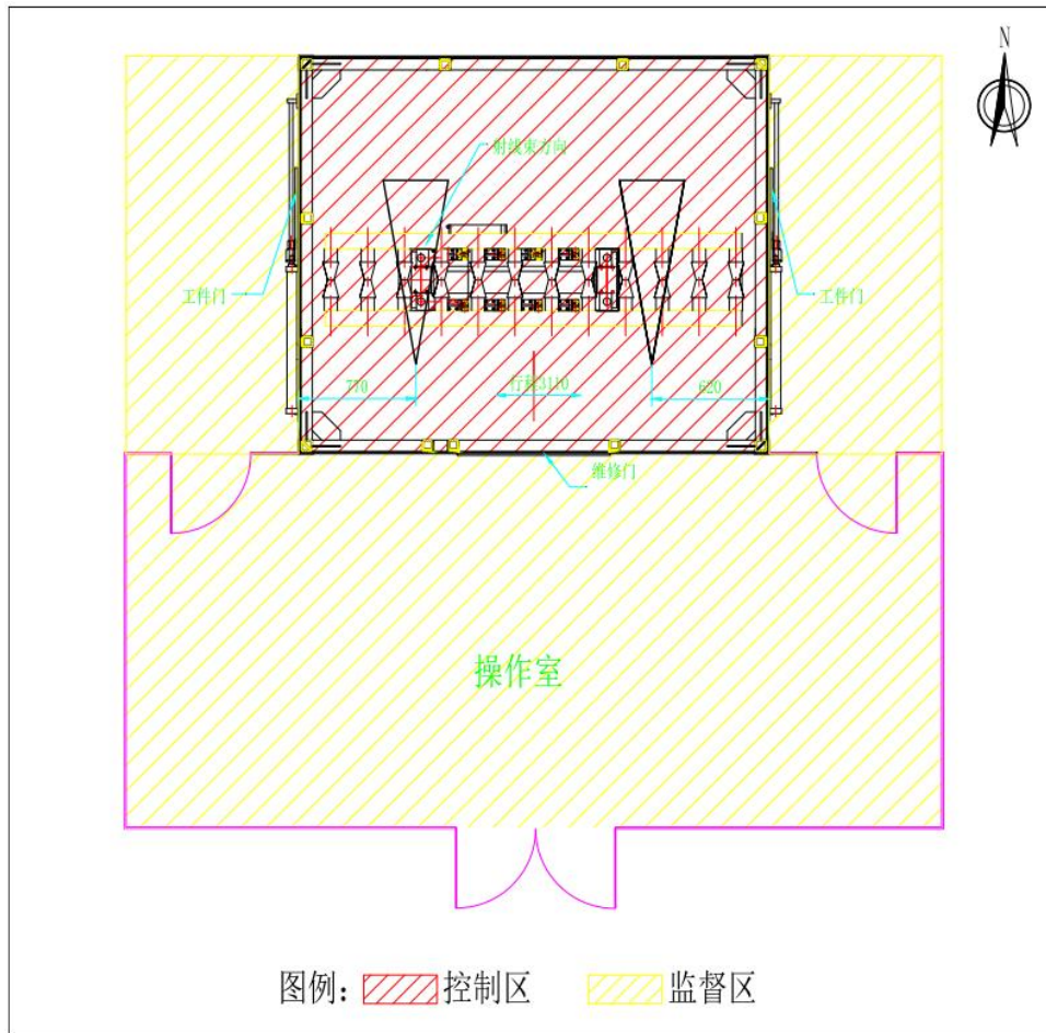
图 10-2 本项目两区划分示意图
