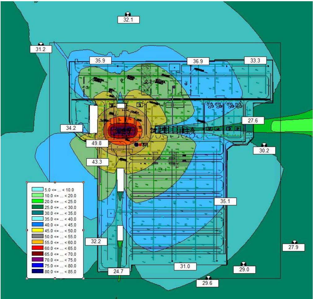
图 6-10 不采取噪声防治措施预测噪声贡献值等声级线图
