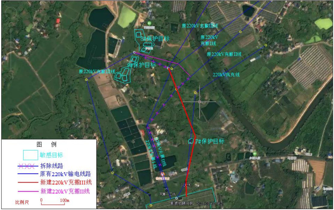
图 2-2 本工程输电线路与环境敏感目标相对位置关系图
