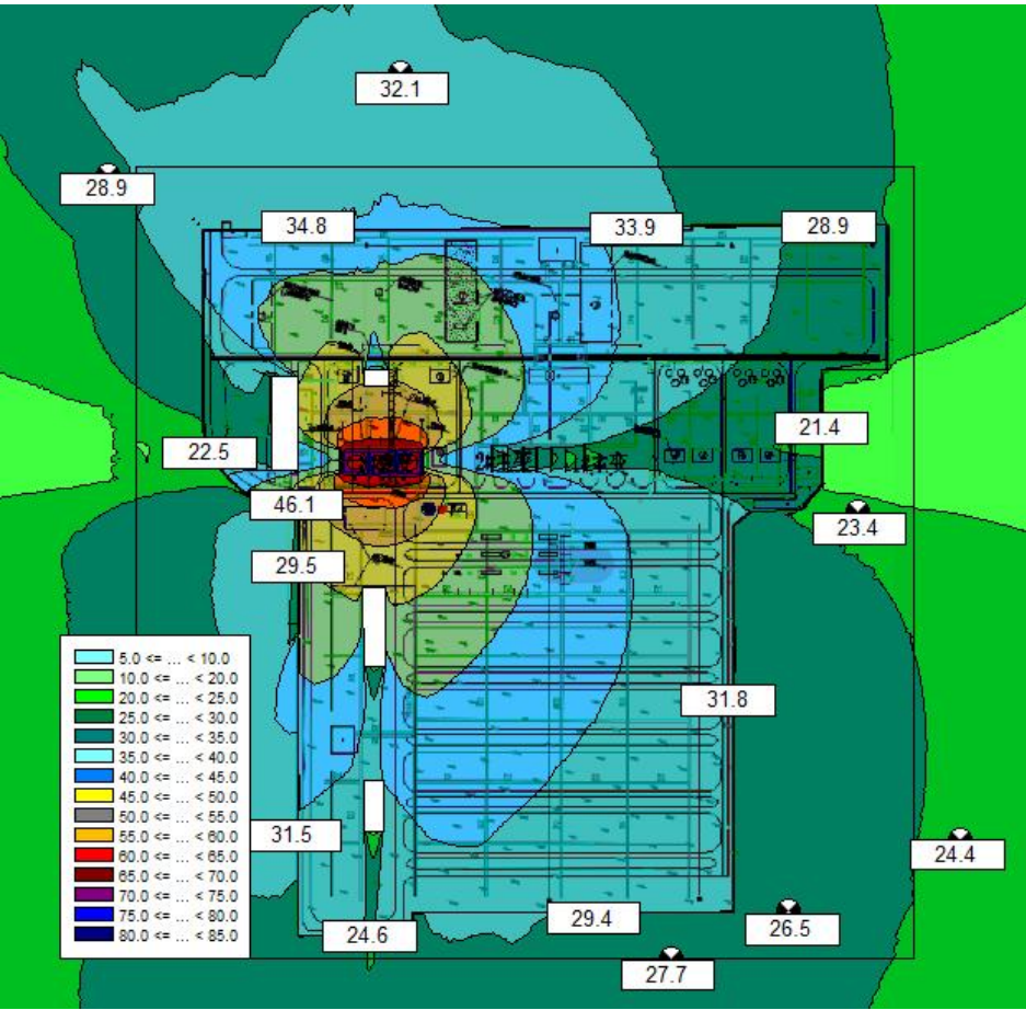
图 6-12 采用噪声防治措施后噪声贡献值等声级线图
