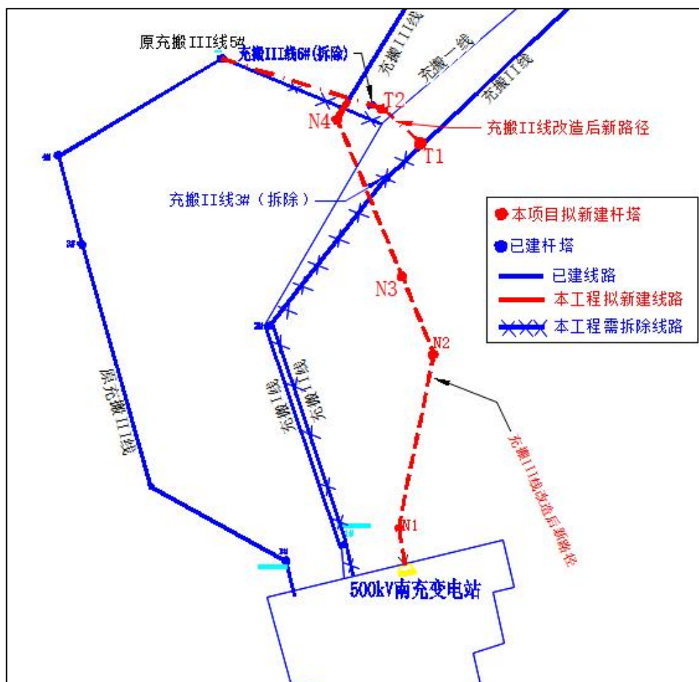
图 1-1 本工程改接线路示意图
