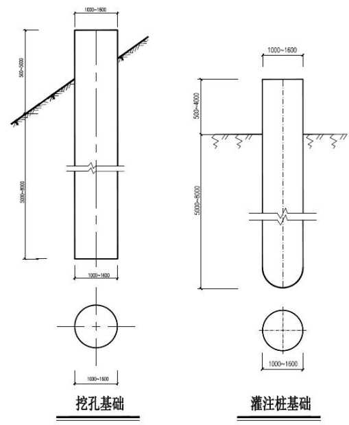
图 3-3 基础型式图
