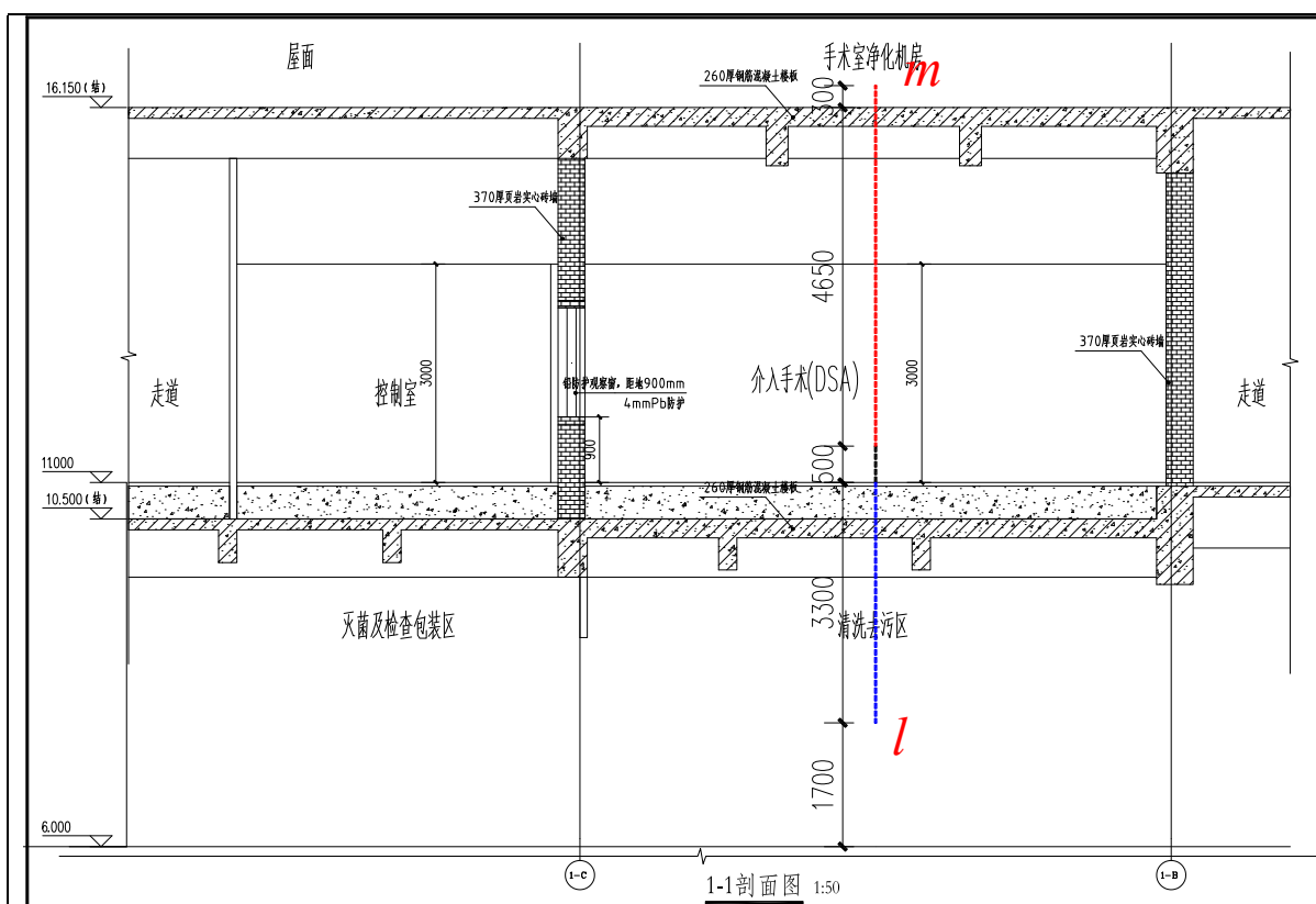
图 11-8 手术中心介入手术室预测点布设示意图
