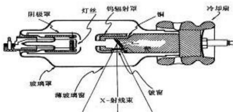
图 9-6 X 射线管基本结构示意图
