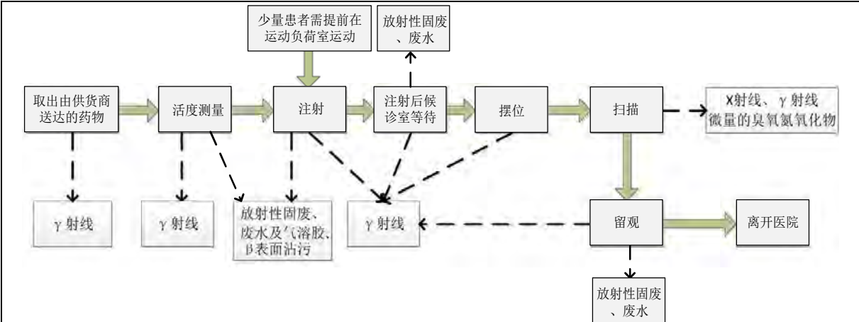
图 9-13 SPECT/CT 诊断项目工作流程及产污环节分析示意图
