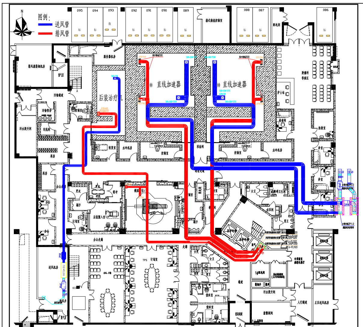
图 10-8 肿瘤科通排风管道布置图
