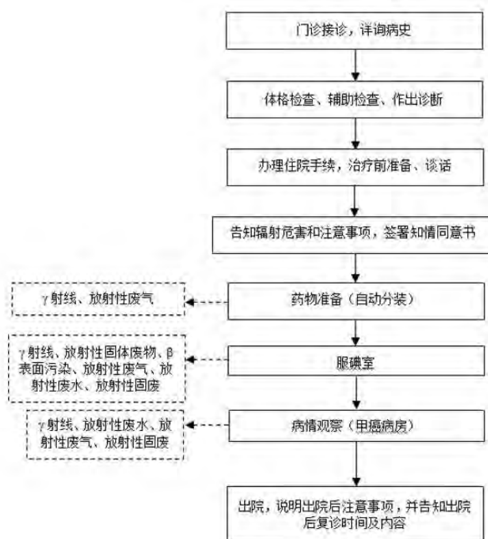
图 9-16 131 I 甲癌治疗项目工作流程及产污环节分析示意图
