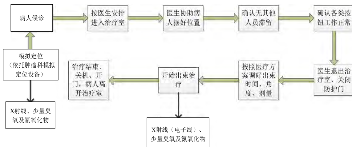
图 9-3 医用电子直线加速器放疗流程及产污环节示意图
