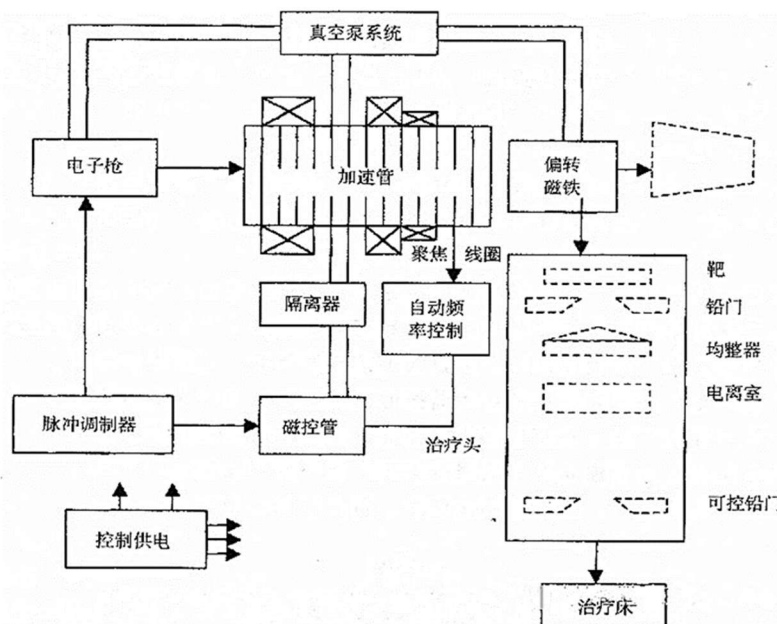
图 9-2 医用电子直线加速器系统示意图
