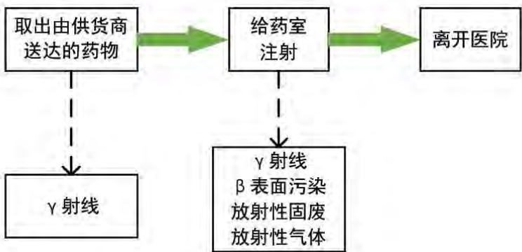
图 9-17 ^{89}\text{Sr} 和 ^{153}\text{Sm} 治疗骨转移项目工作流程及产污环节分析示意图
