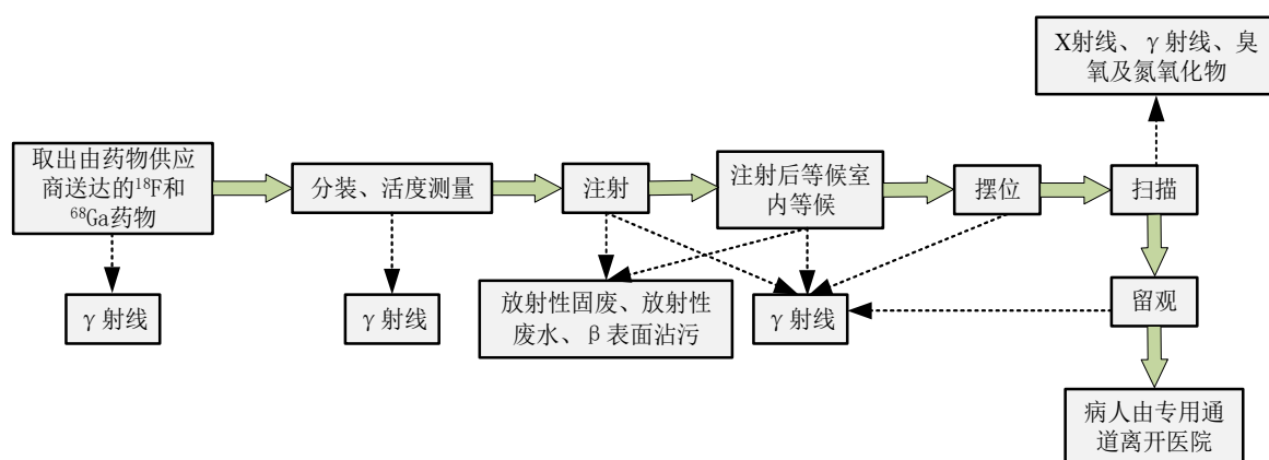
图 9-12 本项目核医学诊断流程及产污环节示意图
