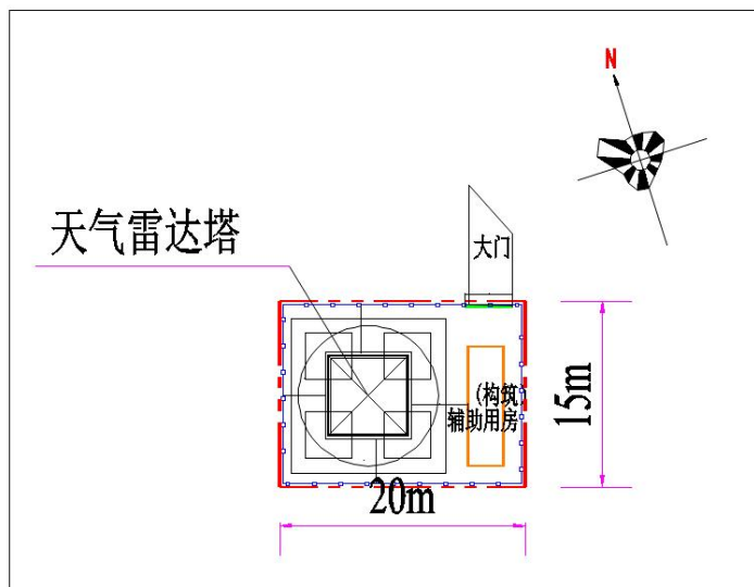
图 3-4 本项目雷达站平面布置图
