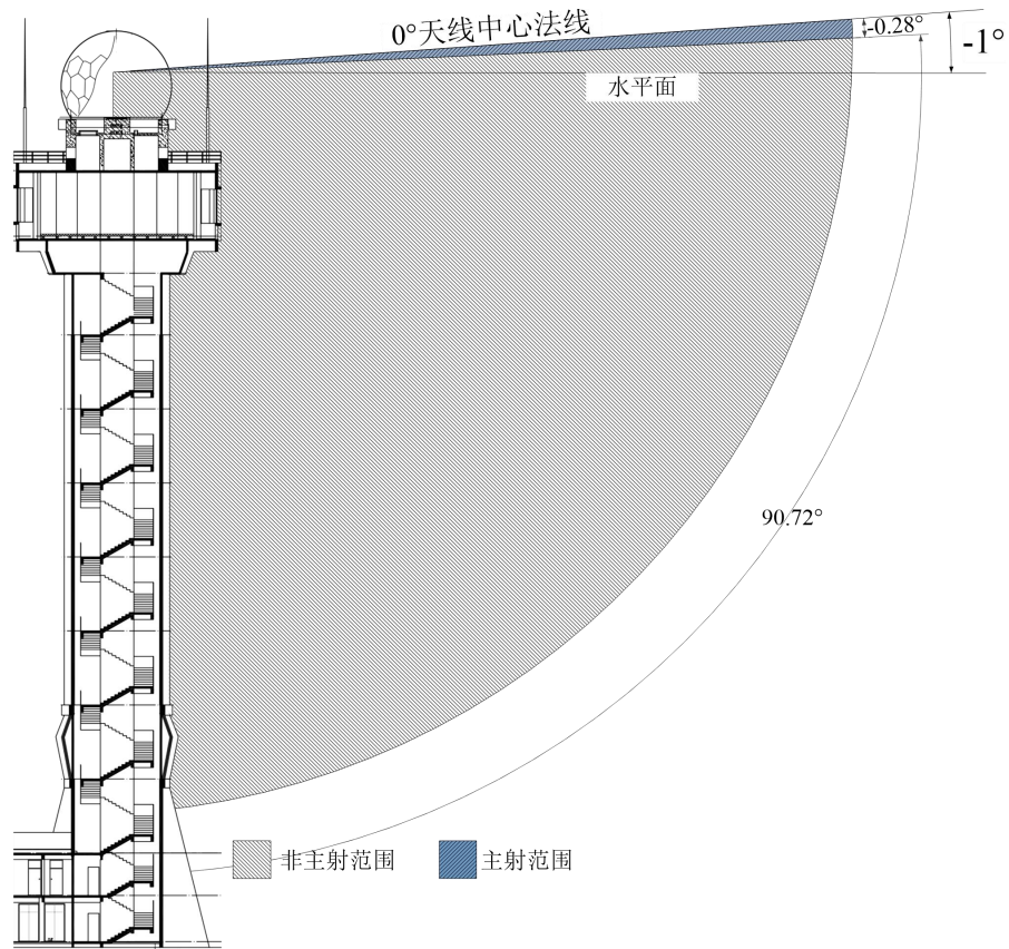
图 6-3 天线主射、非主射范围示意图
