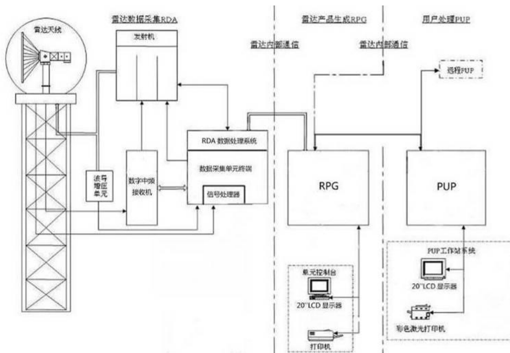
图 3-9 天气雷达系统组成图
