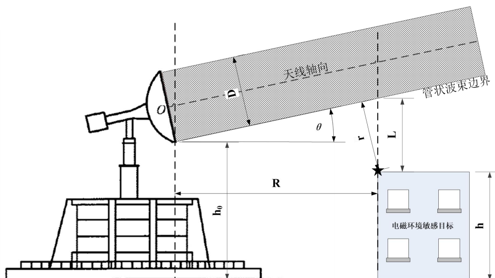
图 6-6 偏轴方向功率密度计算示意图
