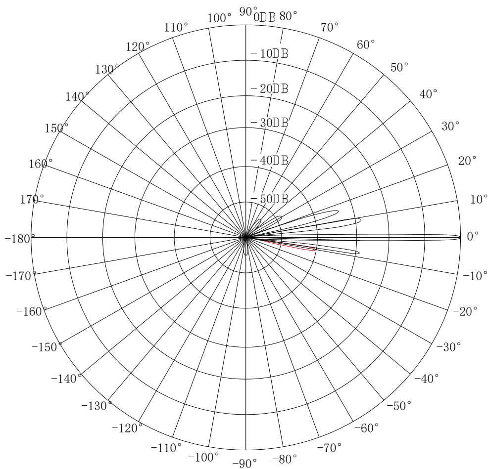
图 6-2 天线垂直方向图
