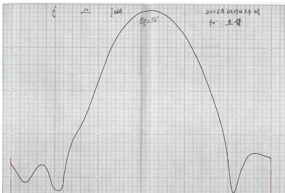
图 6-1 天线水平方向图
