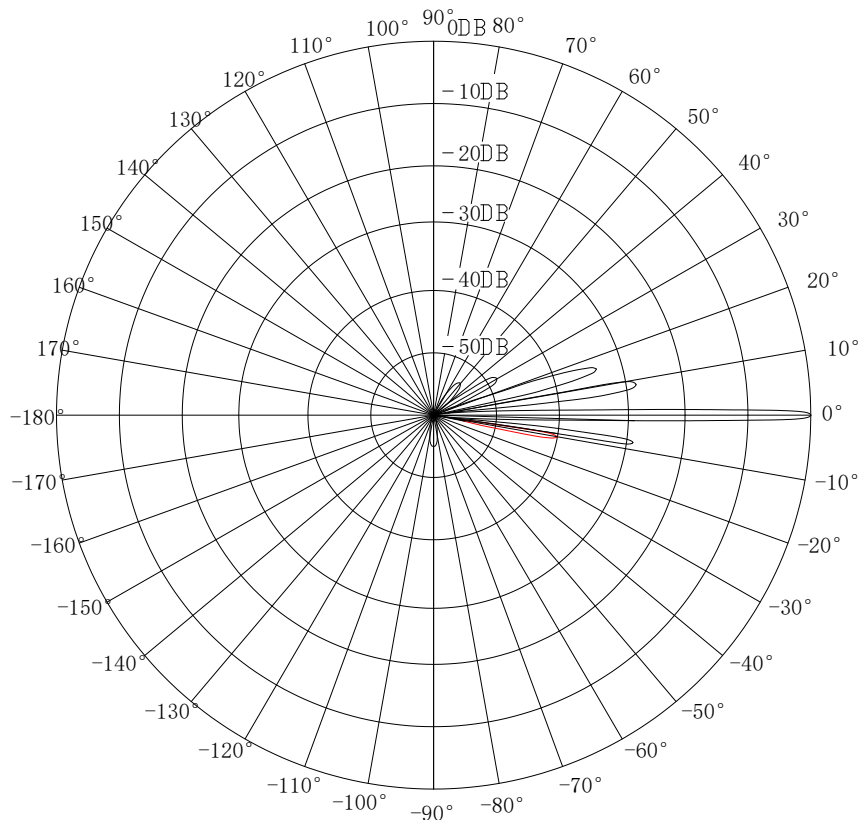
图 3-11 天线垂直方向图
