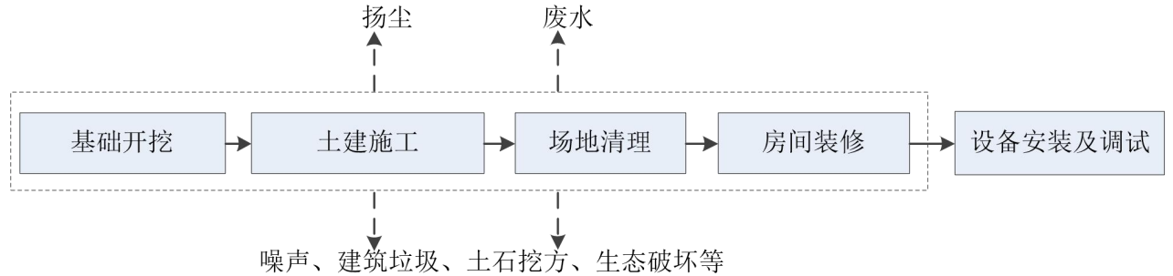
图 3-6 本项目施工期主要产污环节示意图
