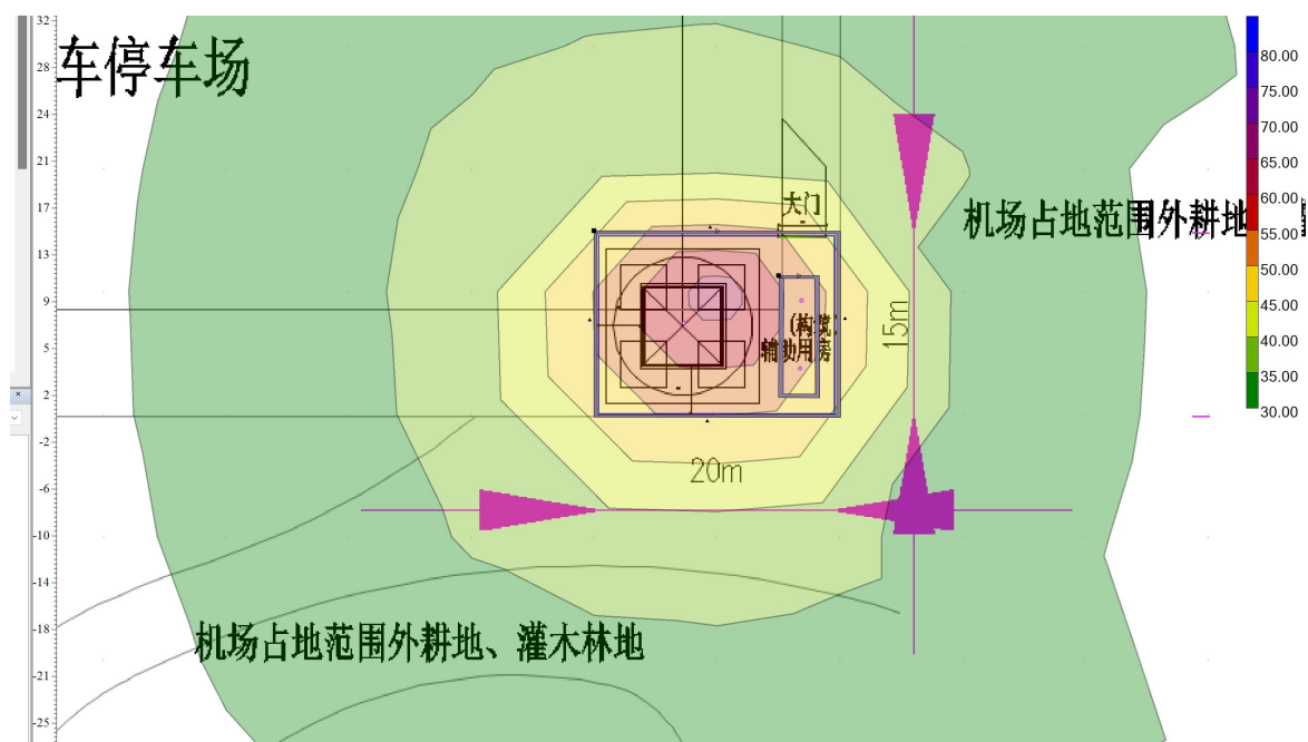
本工程雷达站台处噪声贡献值等声值线图
