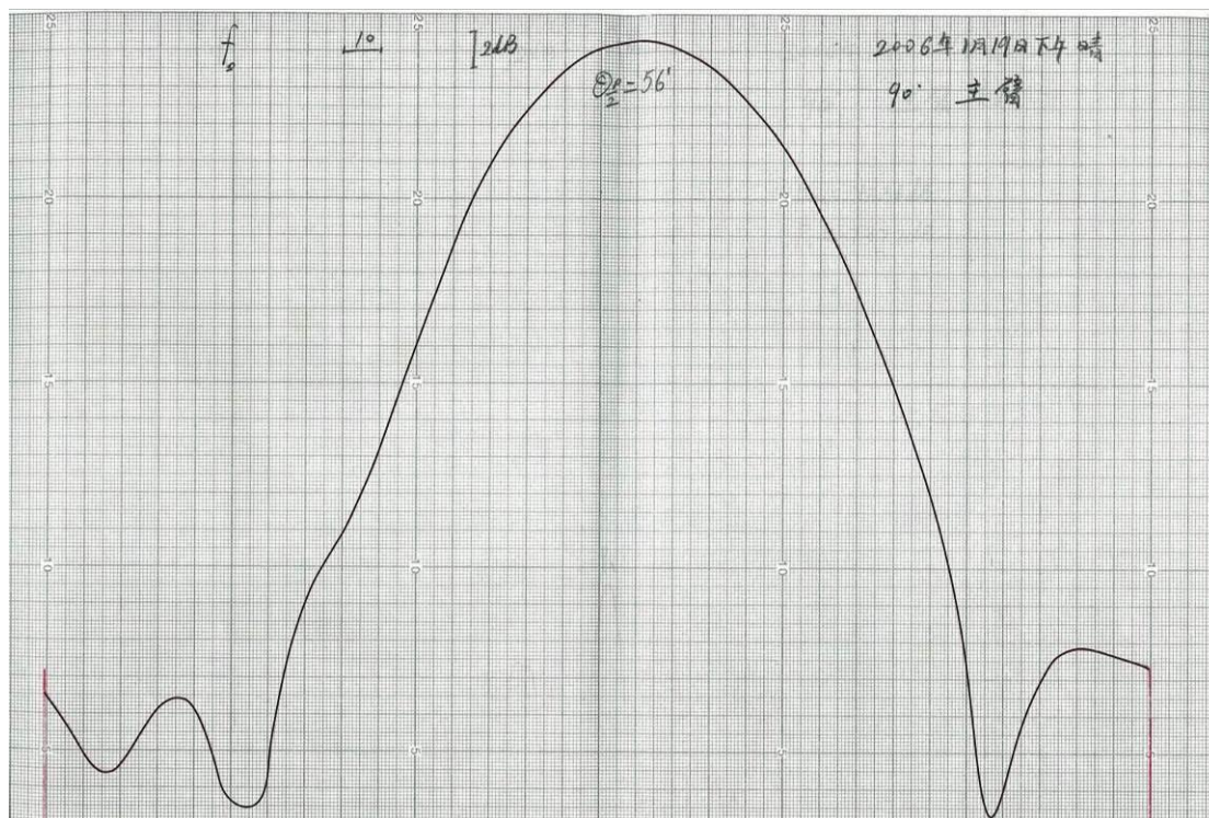
图 3-10 天线水平方向图
