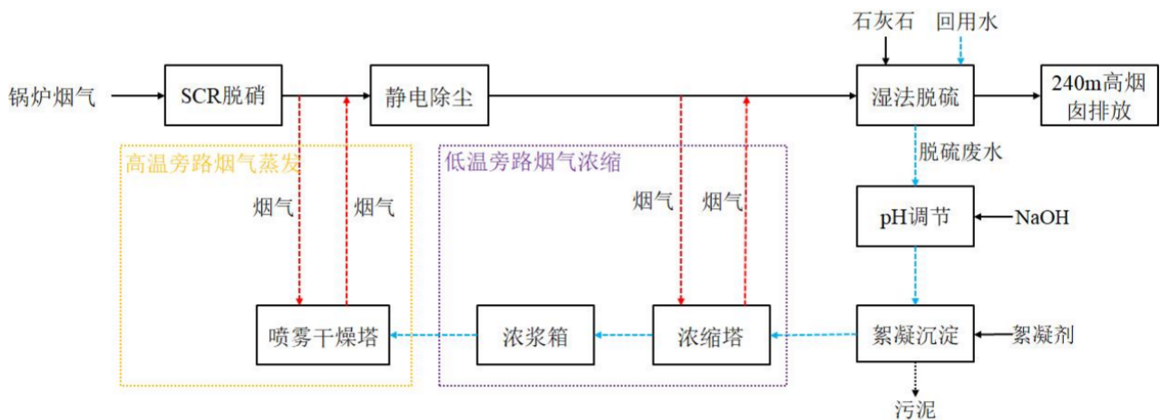
图 7.2-3 脱硫废水处理系统示意图
