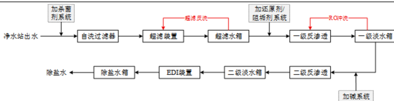
图 3.1-8 锅炉补给水处理流程示意图
