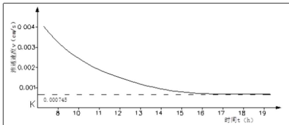
图 4.1-6 ST1 渗水试验渗透速度历时曲线图
