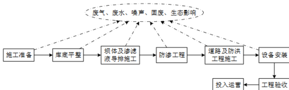
图 3.2-2 罗家湾灰场施工流程及产污环节图
