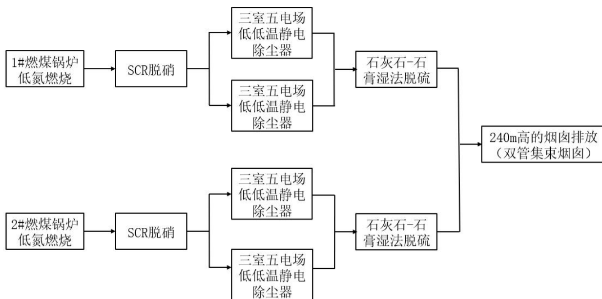
图 7.1-1 拟建项目烟气处理总体工艺路线图
