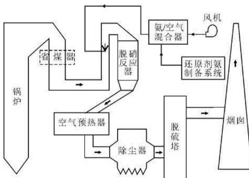
图 7.1-2 拟建项目烟气处理设施总体连接示意图
