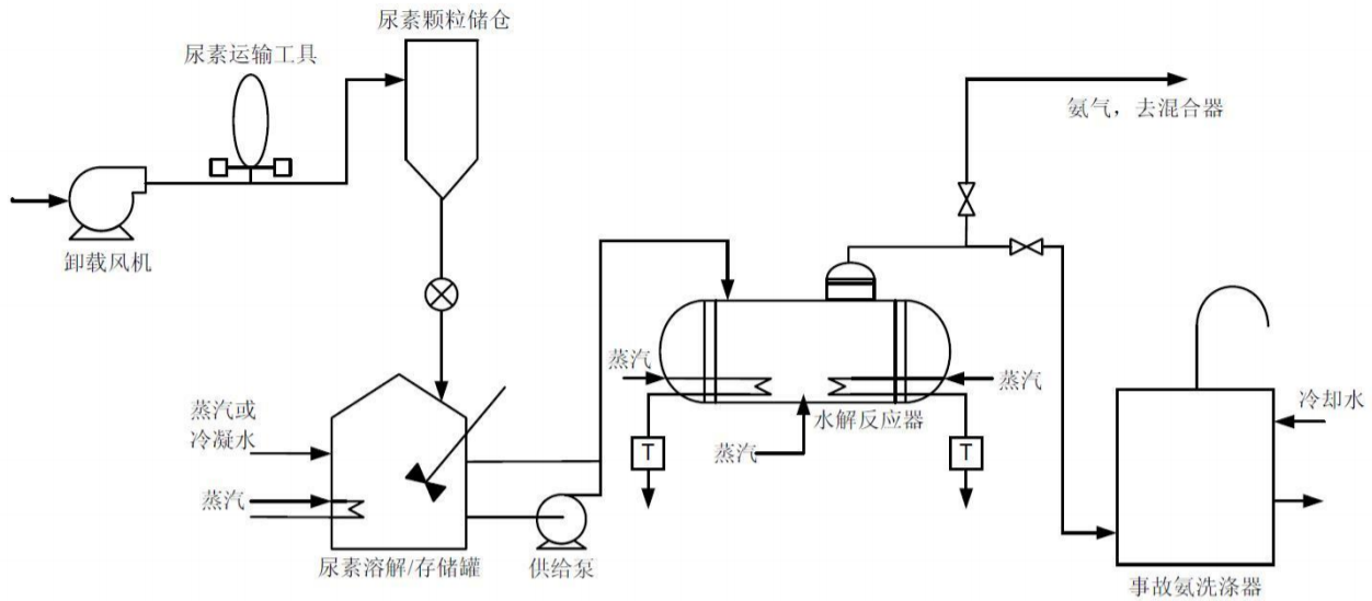
图 7.1-5 尿素水解制氨工艺系统示意图
