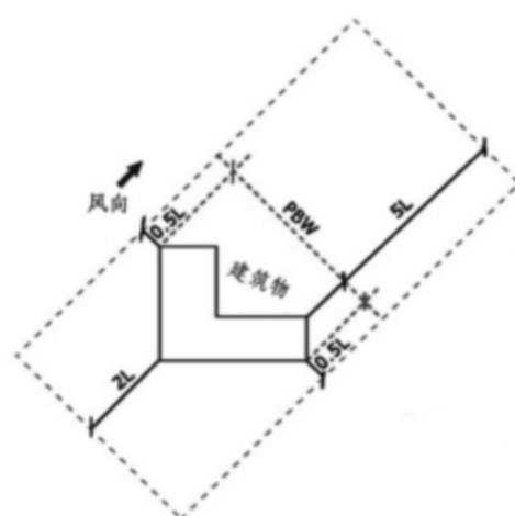
图 5.1-3 建筑物影响区域
