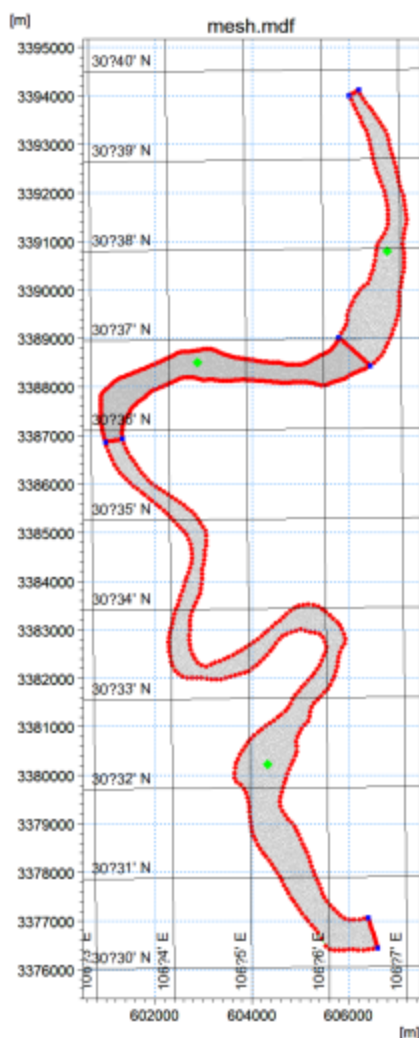
图 5.2-1 评价区河段网格剖分图
