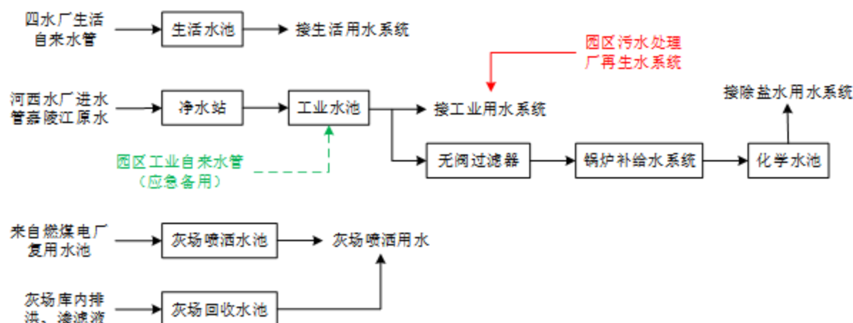
图 3.1-7 供水方案示意图
