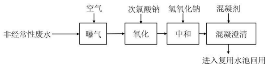
图 7.2-2 非经常性废水处理系统废水处理工艺流程图
