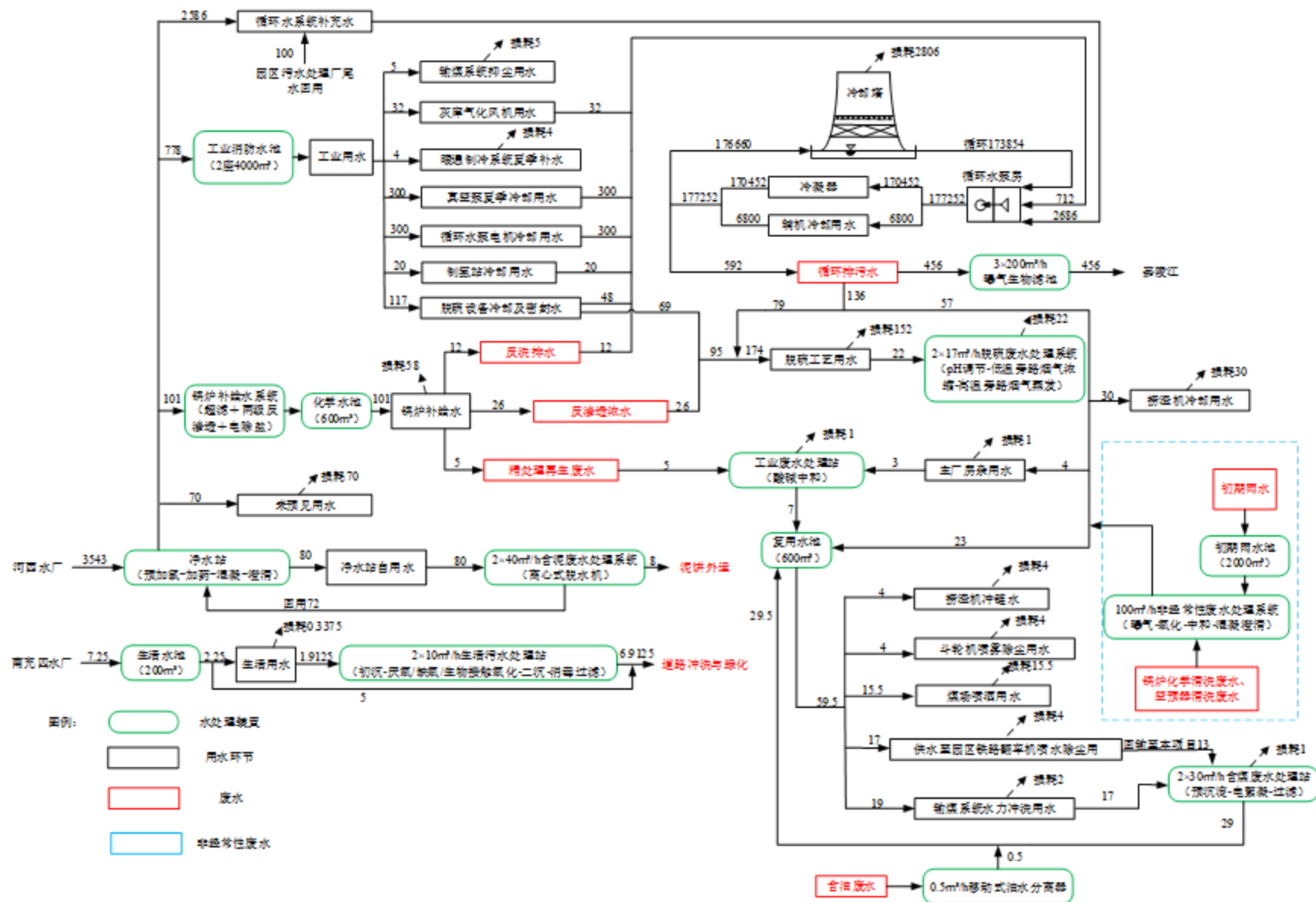
图 3.3-7 拟建 2×1000MW 机组夏季气象条件下水平衡图 (单位: \text{m}^3/\text{h} )
