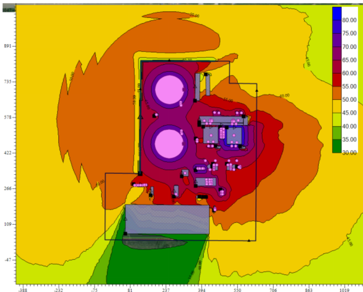
图 5.3-3 锅炉排汽偶发噪声等声值线图
