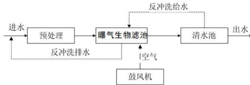
图 7.2-5 曝气生物滤池工艺流程
