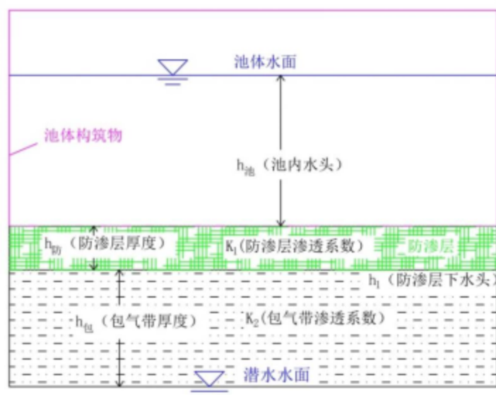
图 3.3-11 有防渗条件的池体构筑物废水下渗示意图
