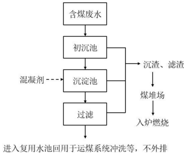
图 7.2-4 含煤废水处理系统工艺流程图
