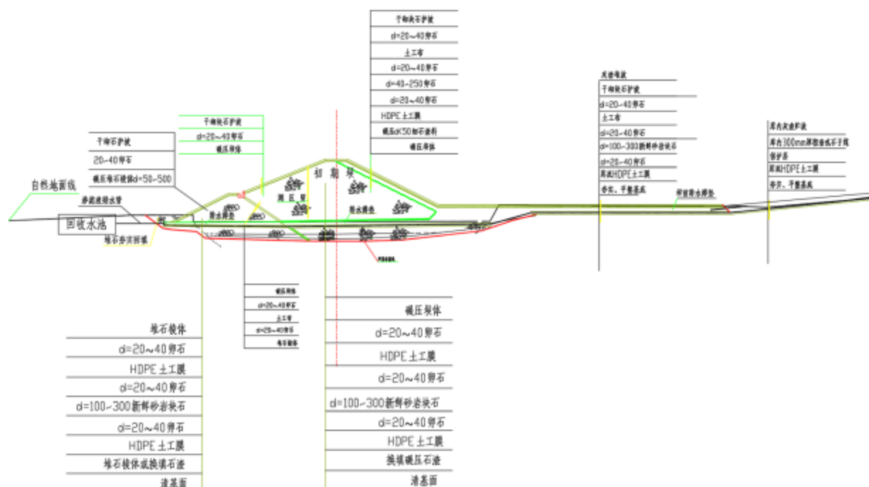
图 3.1-5 灰场防渗导排系统示意图
