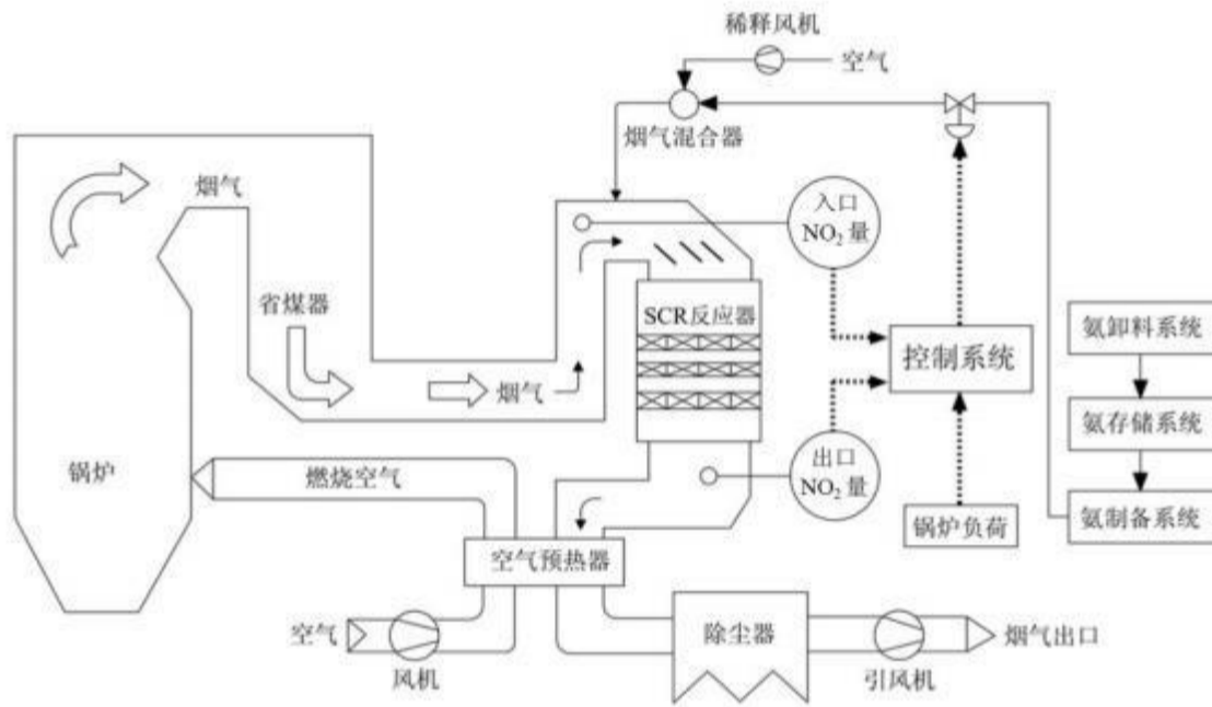
图 7.1-3 SCR 脱硝总体工艺流程图
