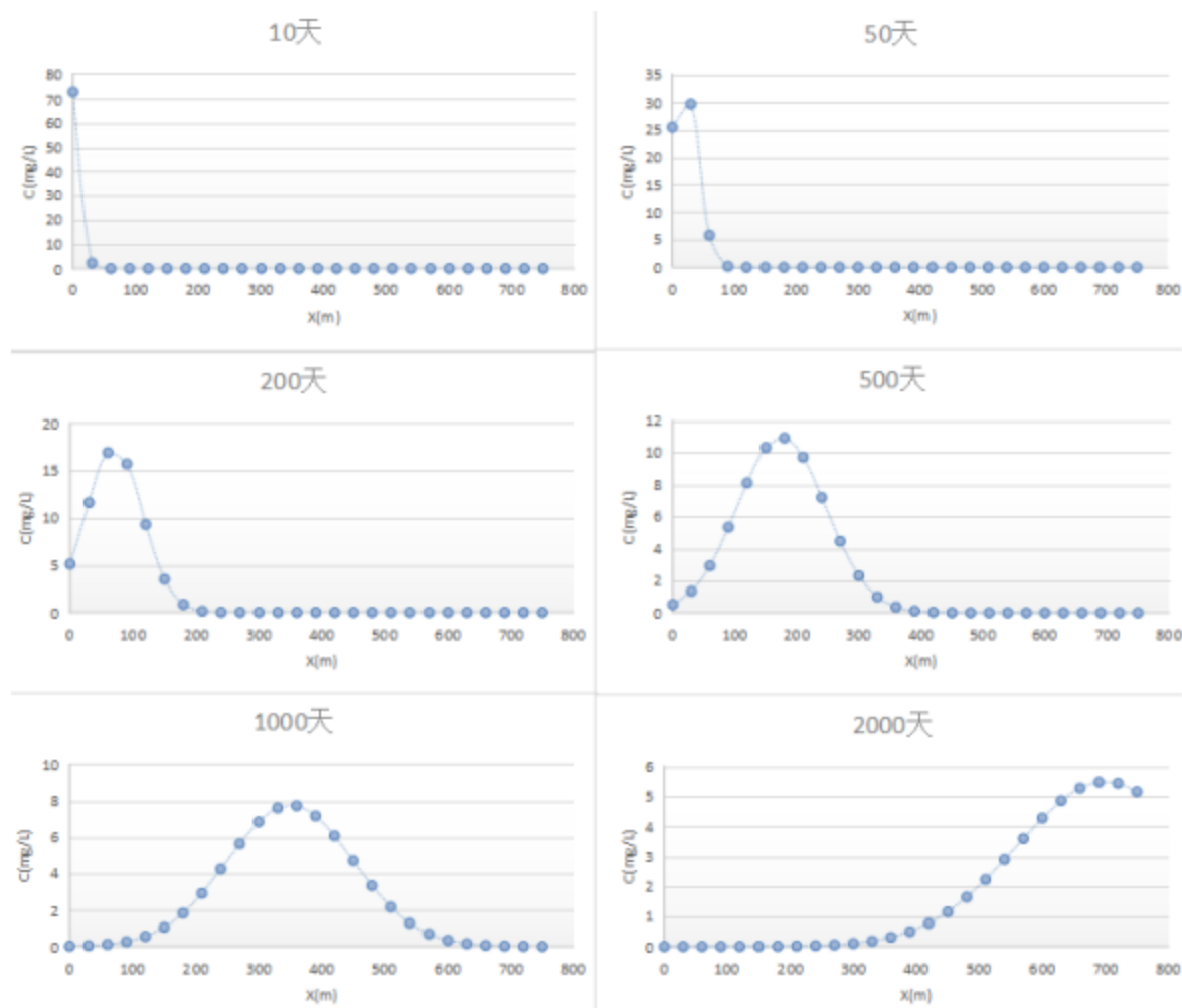
图 5.4-6 非正常工况石油类下渗进入下伏含水层迁移情况
