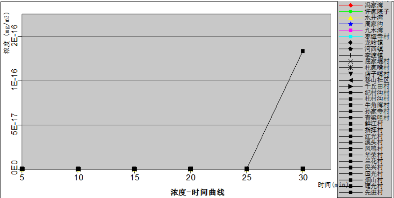
图 6.7-9 最不利气象条件下柴油火灾、爆炸事故各关心点一氧化碳浓度随时间变化情况
