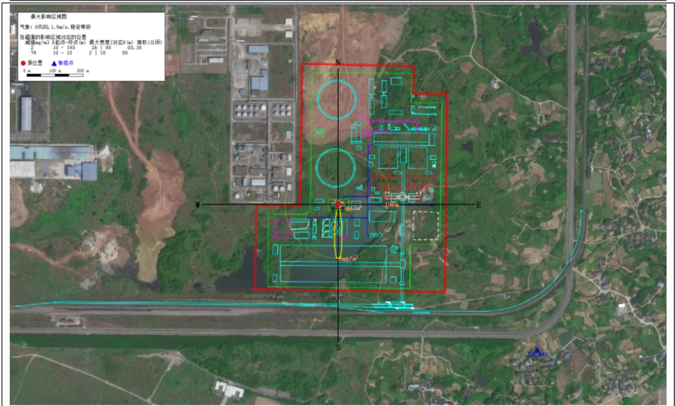
图 6.7-5 最不利气象条件下柴油火灾、爆炸事故下风向不同距离处二氧化硫出现浓度
