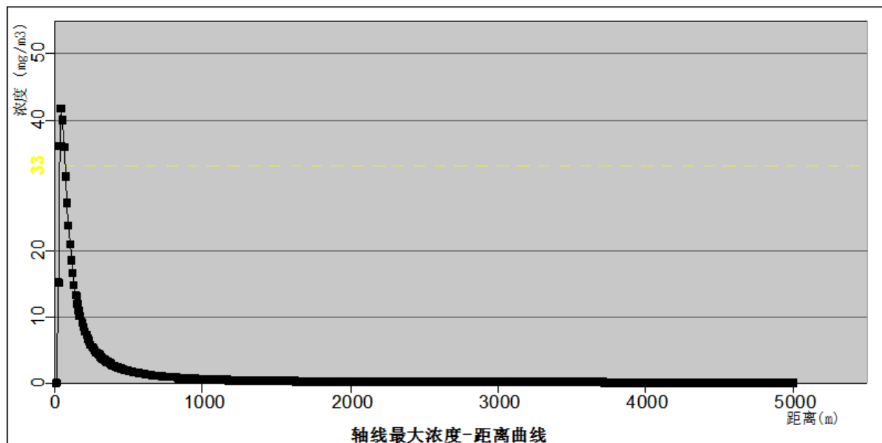
图 6.7-1 最不利气象条件下盐酸储罐泄漏下风向不同距离处有毒有害物质出现浓度
