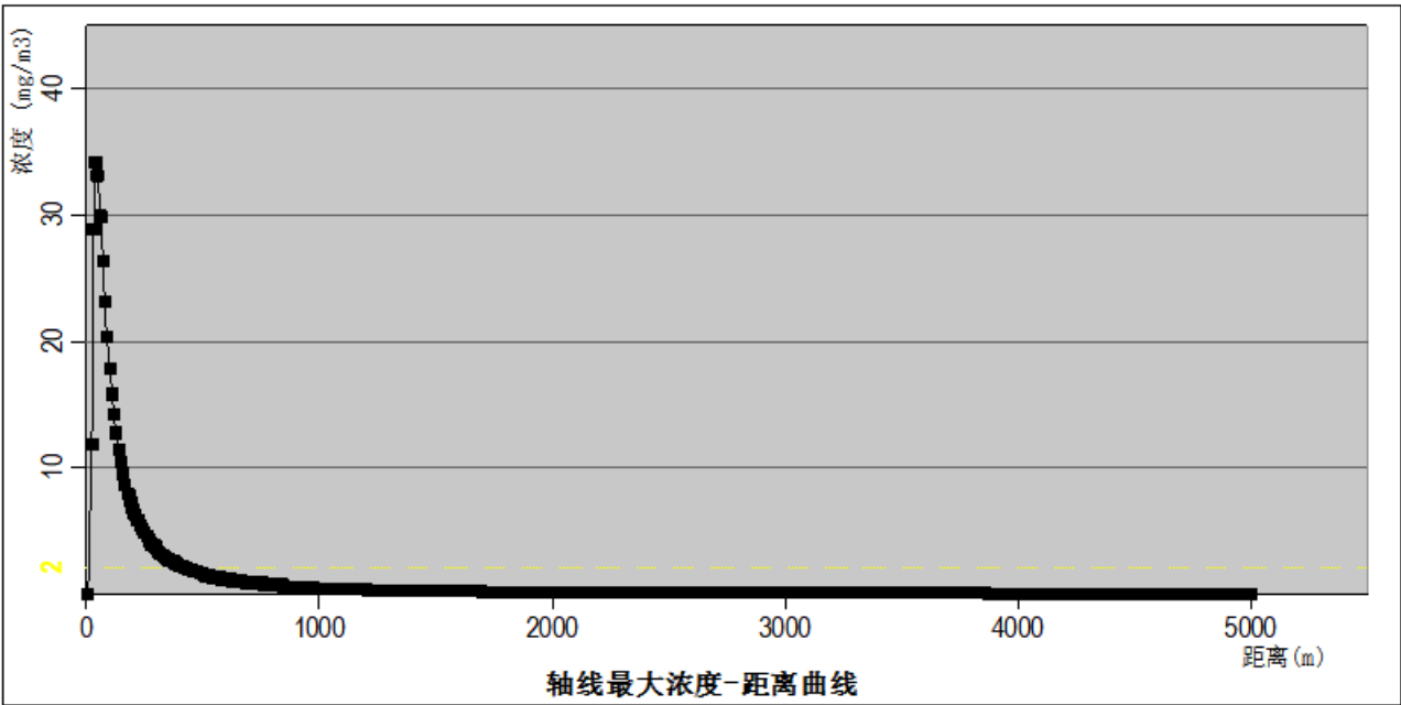
图 6.7-2 最不利气象条件下柴油火灾、爆炸事故下风向不同距离处二氧化硫出现浓度曲线图
