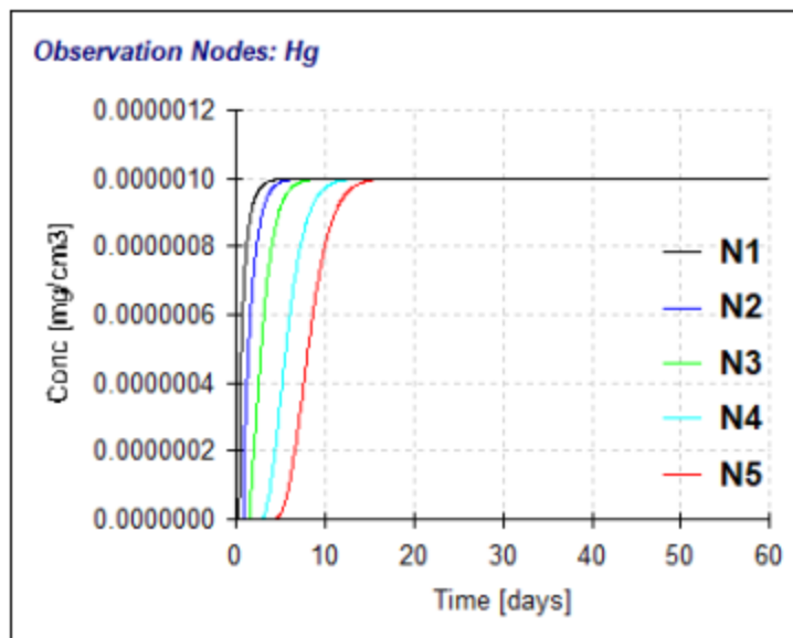
图 5.6-9 土壤不同深度汞浓度-时间预测曲线图
