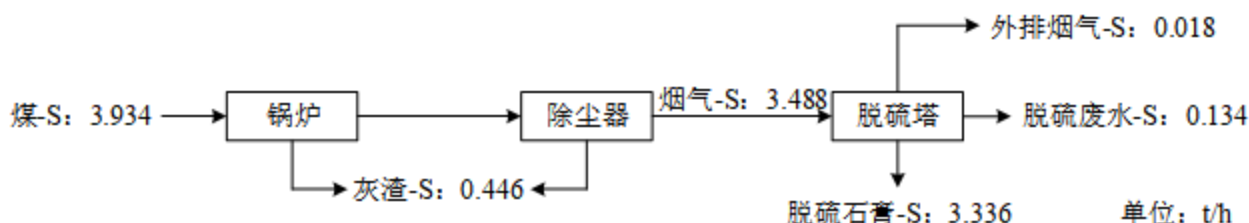
图 3.3-1 项目设计煤种硫平衡图
