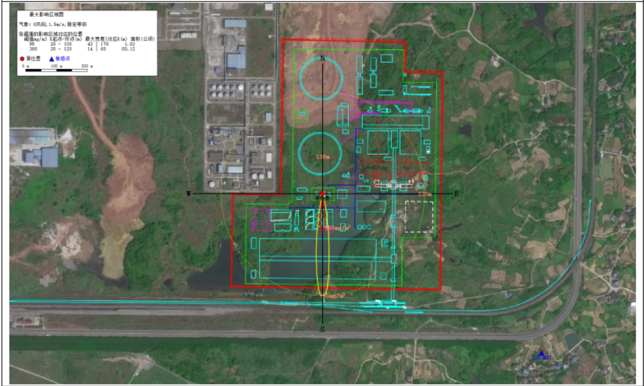
图 6.7-6 最不利气象条件下柴油火灾、爆炸事故下风向不同距离处一氧化碳出现浓度
