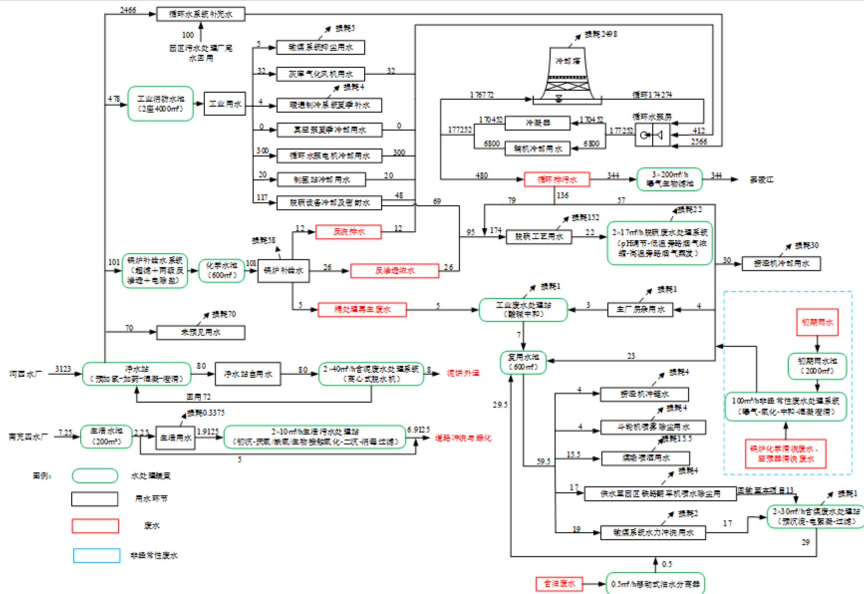
图 3.3-9 拟建 2×1000MW 机组年均气象条件下水平衡图 (单位: m^3/h )
