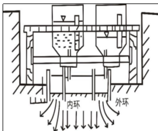
图 4.1-5 双环法渗水试验装置
