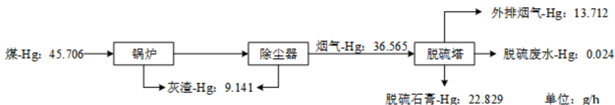
图 3.3-5 项目校核煤种 1 汞平衡图
