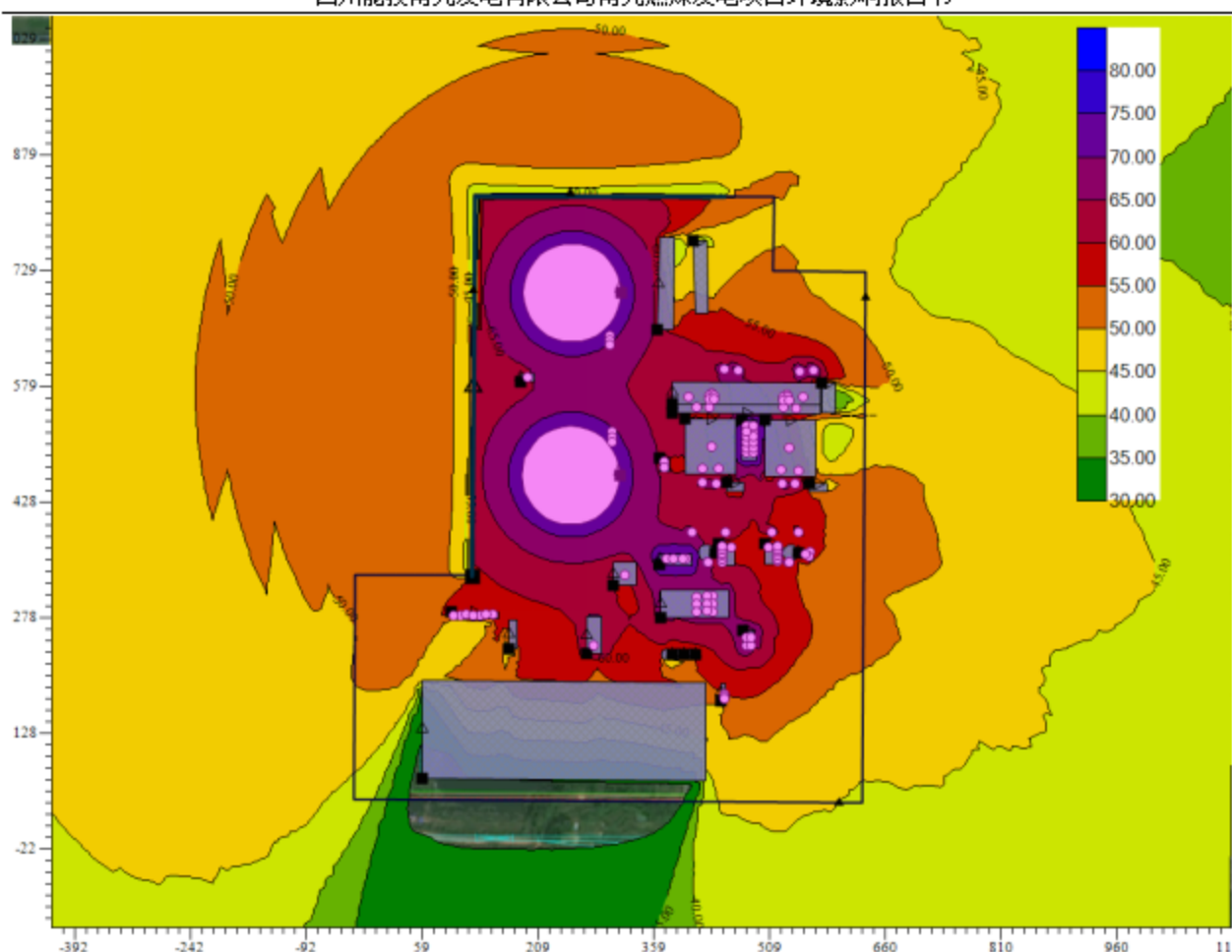
图 5.3-2 正常工况下燃煤电厂等声值线图
