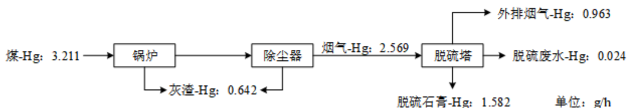
图 3.3-4 项目设计煤种汞平衡图
