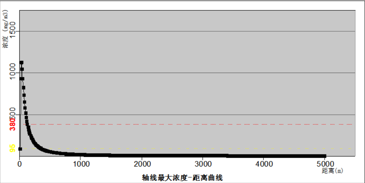
图 6.7-3 最不利气象条件下柴油火灾、爆炸事故下风向不同距离处一氧化碳出现浓度曲线图
