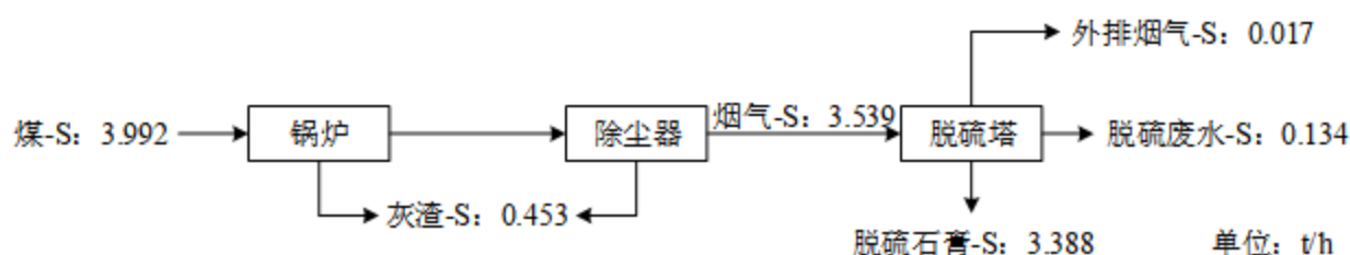
图 3.3-1 项目设计煤种硫平衡图
