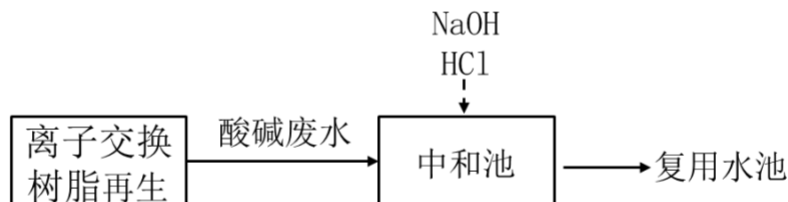
图 7.2-1 锅炉补给水处理系统废水处理工艺流程图
