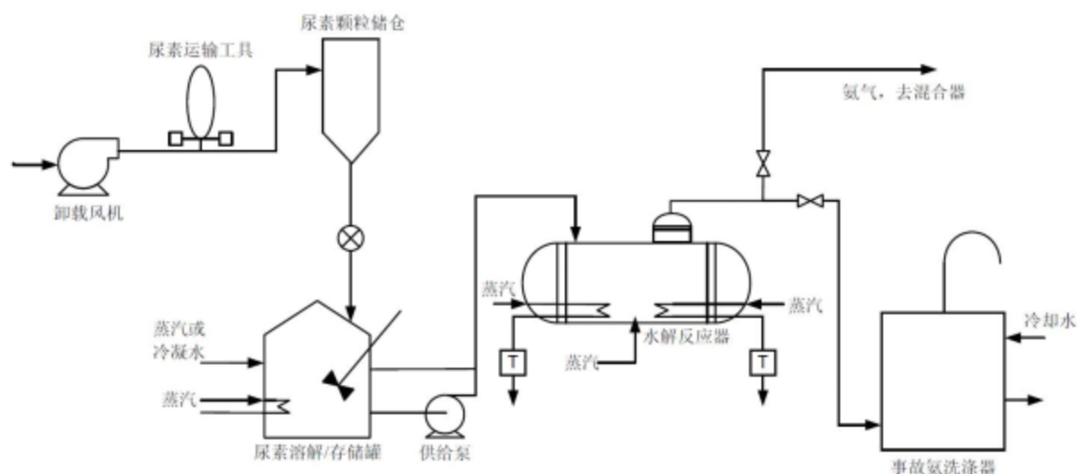
图 3.2-4 尿素水解制氨工艺原理图
