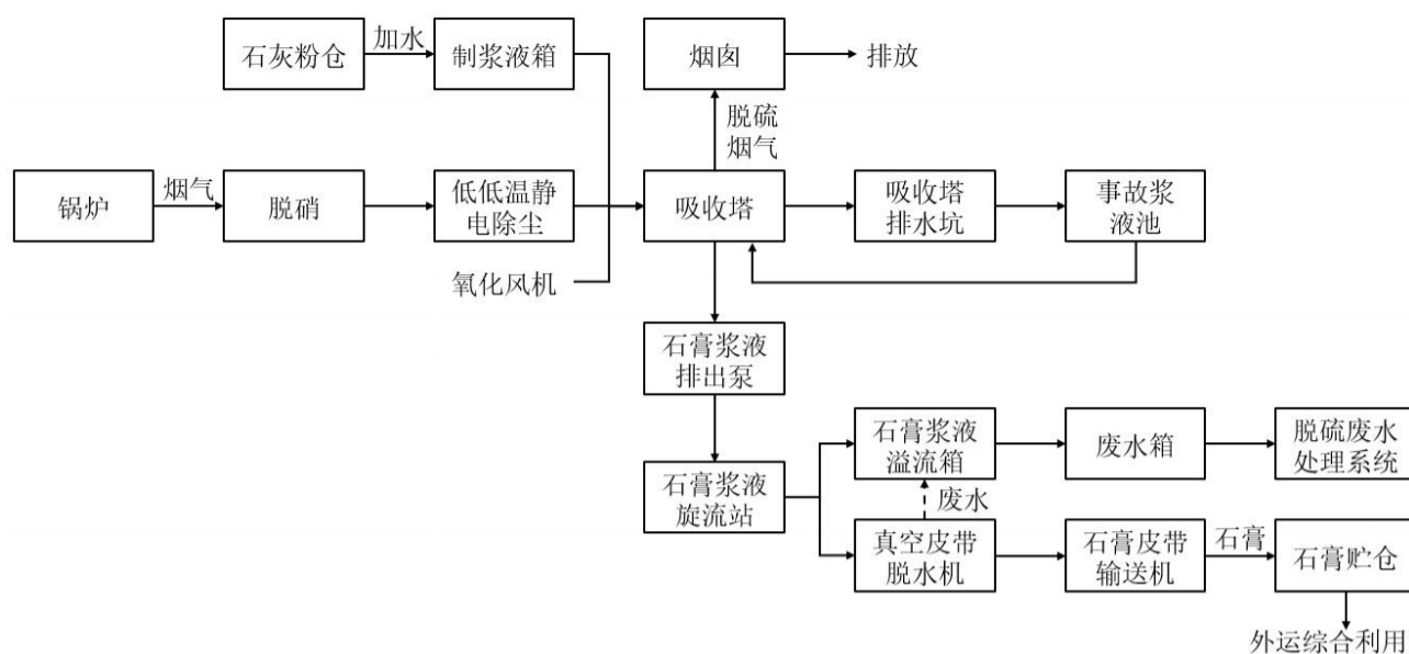
图 7.1-6 脱硫系统工艺流程示意图
