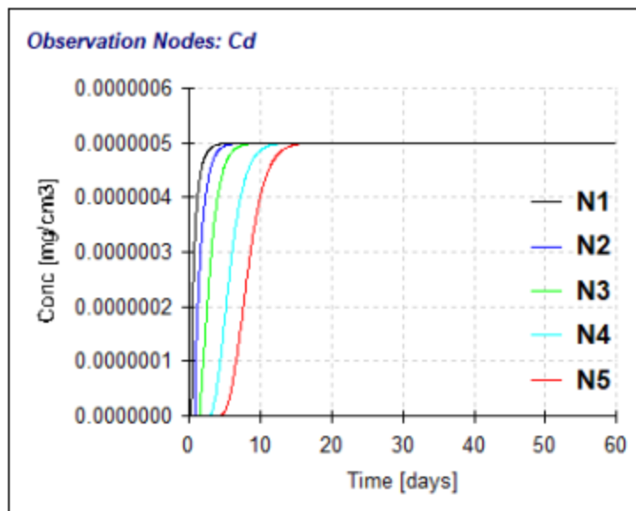
图 5.6-10 土壤不同深度镉浓度-时间预测曲线图
