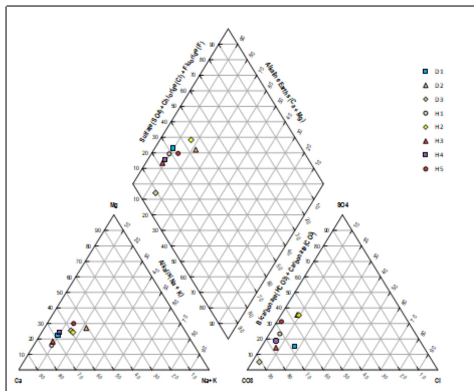
图 4.1-8 水化学 piper 三线图
