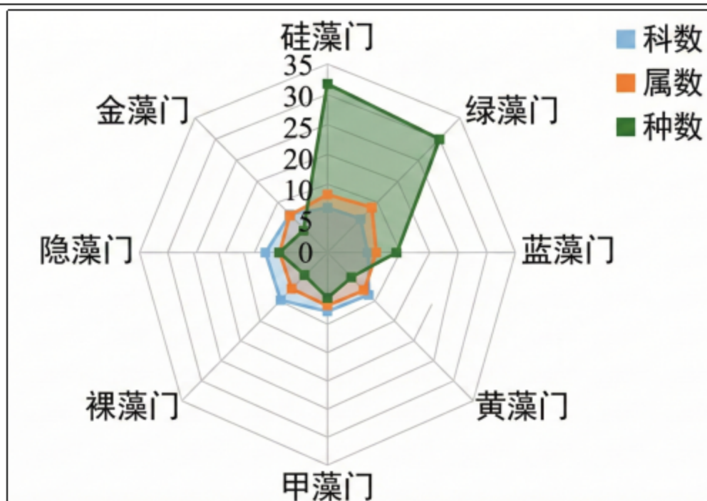
图 4.3-6 各门类浮游植物科、属、种数量雷达图
