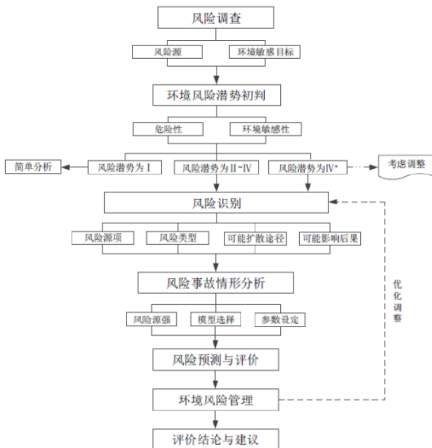
图 6.1-1 环境风险评价程序图
