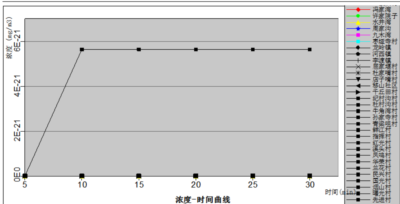
图 6.7-7 最不利气象条件下盐酸储罐泄漏各关心点有毒有害物质浓度随时间变化情况
