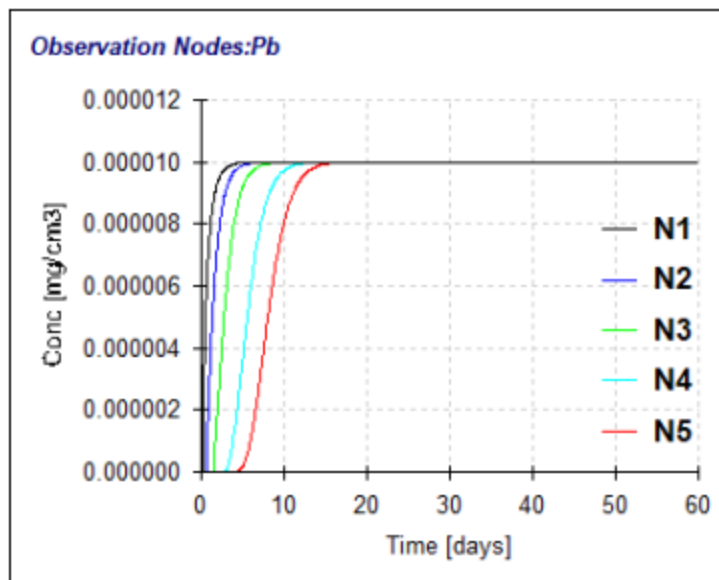
图 5.6-13 土壤不同深度铅浓度-时间预测曲线图
