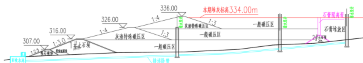
图 3.1-4 罗家湾灰场剖面示意图
