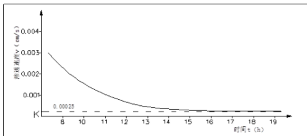
图 4.1-7 ST2 渗水试验渗透速度历时曲线图
