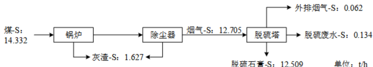
图 3.3-2 项目校核煤种 1 硫平衡图
