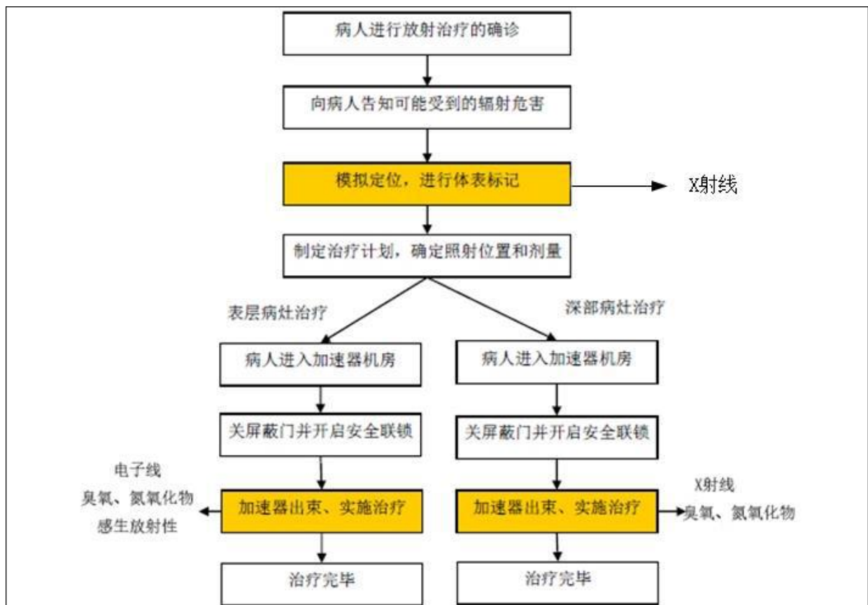
图 9-5 医用直线加速器放疗流程及产污环节示意图
