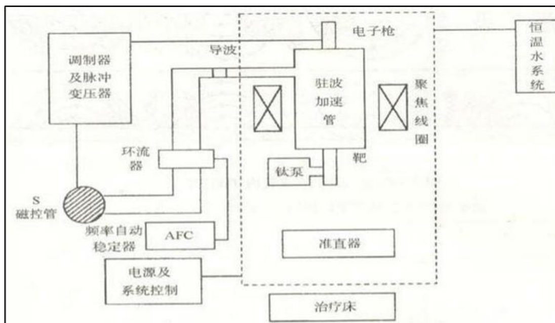
图 9-1 医用电子直线加速器内部结构图
