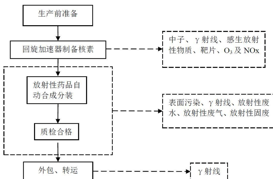
图9-7 回旋加速器制药场所流程及产污环节图
