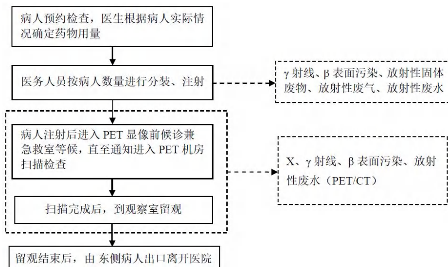
图9-9 PET诊断项目工作流程与产污流程图
