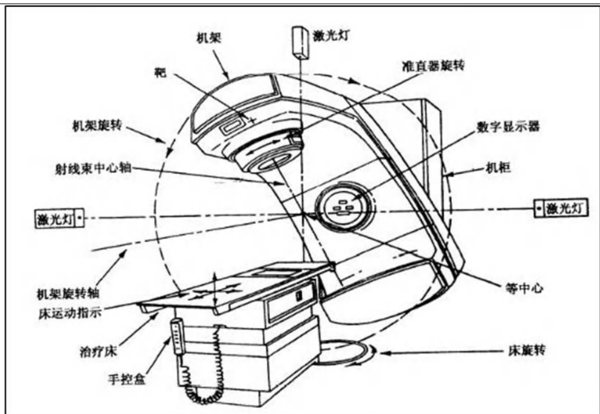
图 9-3 典型医用直线加速器外观结构图
