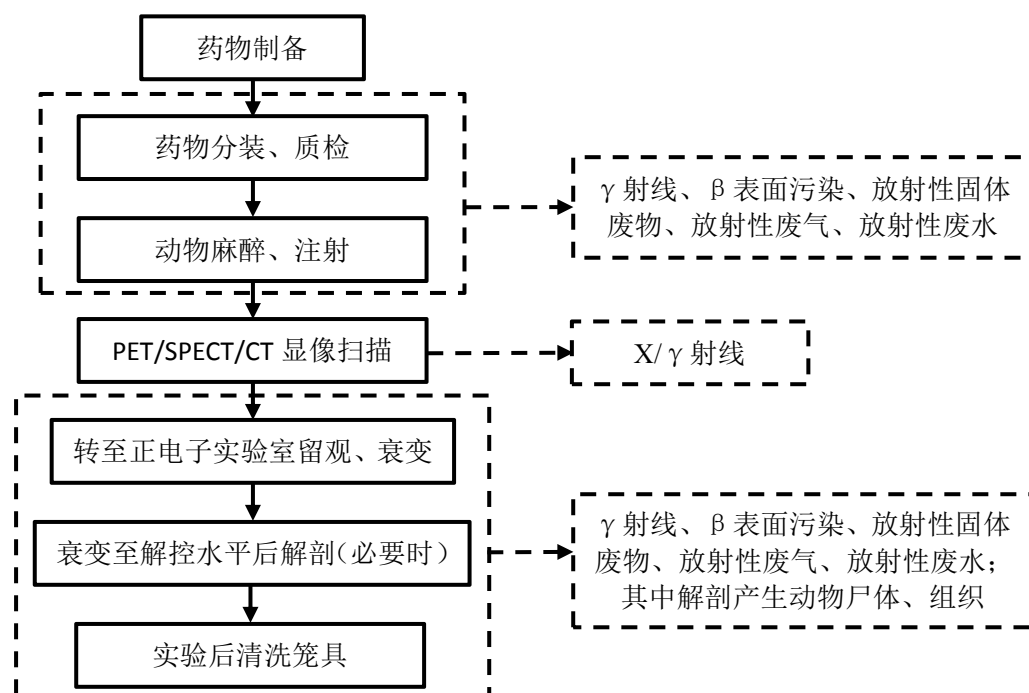
图9-8 动物实验流程及产污流程图
