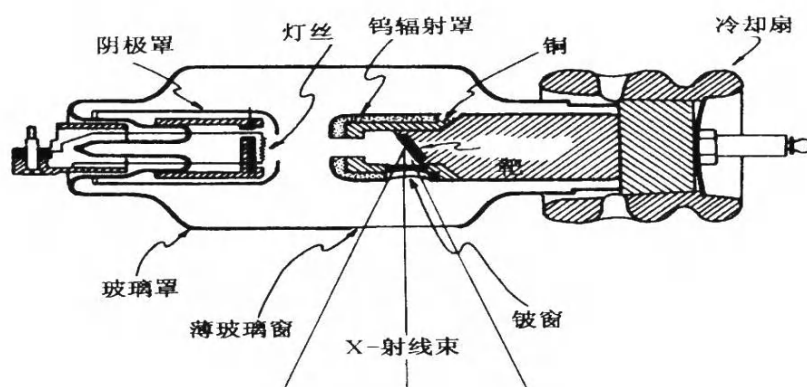
图 9-16 典型 X 射线管结构图
