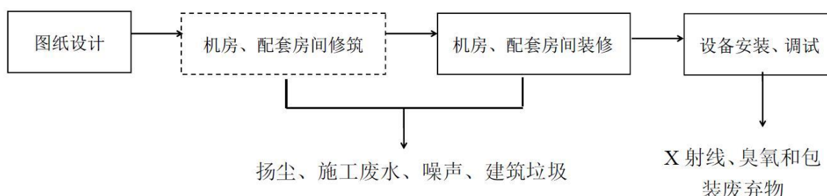
图 9-20 施工期施工工序及产污位置图（虚线框不属于本次评价内容）
