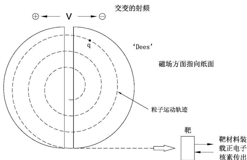
图9-6 回旋加速器工作原理示意图
