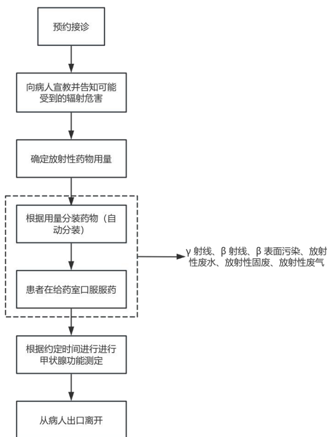
图 9-12 甲吸检查项目工作流程及产污环节分析
